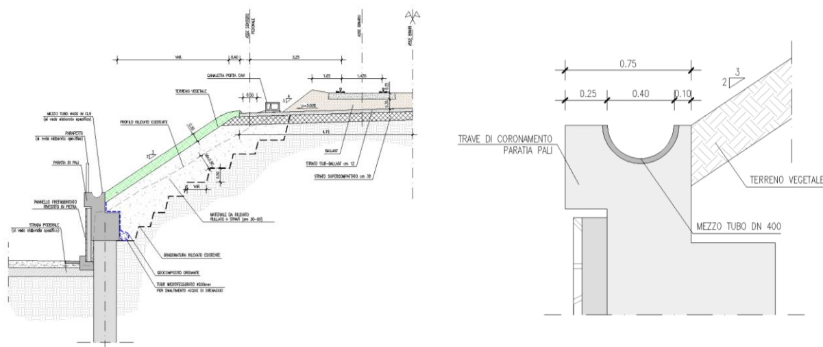
Schema di drenaggio acque di piattaforma in corrispondenza della paratia di pali
