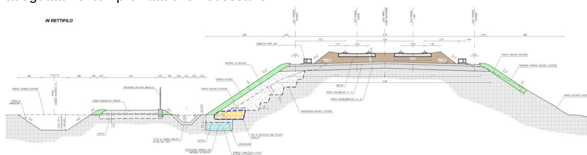
Sezione tipologica con il nuovo rilevato in sovrapposizione all'esistente
