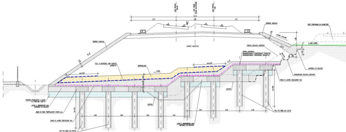
Sezione con consolidamento terreno mediante pali CFA
