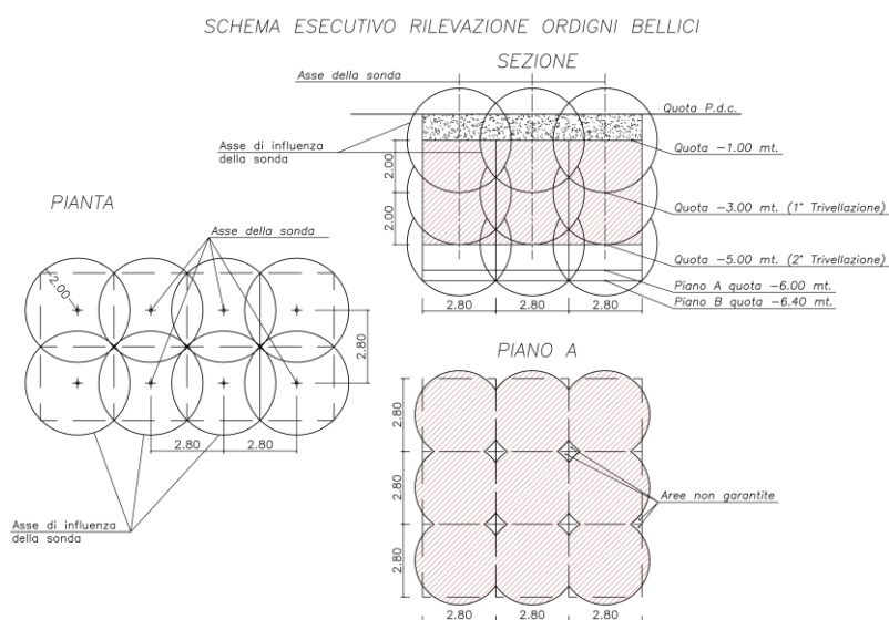
Schema esecutivo rilevazione ordigni bellici
