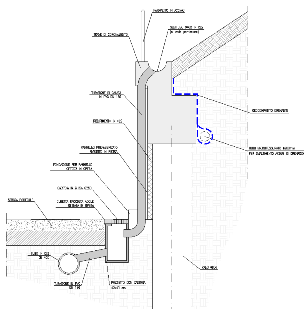
Dettaglio dello scarico della canaletta semicircolare
