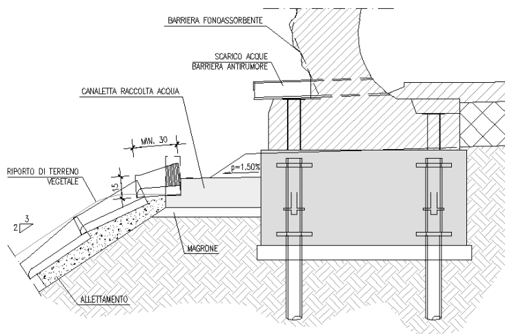
Dettaglio del drenaggio acque di piattaforma in corrispondenza di barriere antirumore
