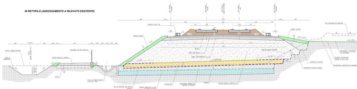
Sezione tipologica con il nuovo rilevato in affiancamento all'esistente
