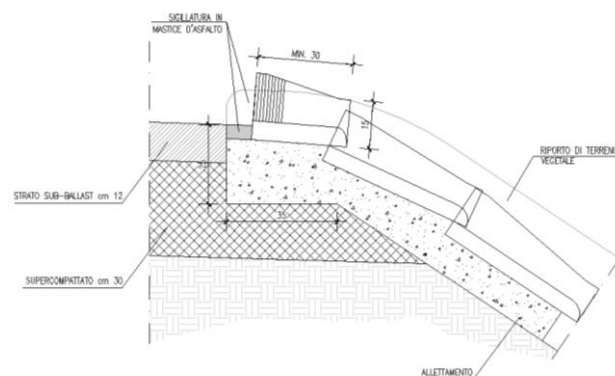
Dettaglio dello scarico delle piogge nell'embrice
