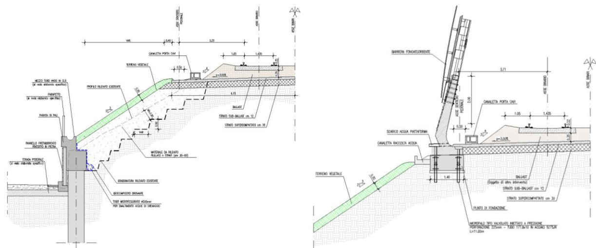
Dettaglio della sezione tipologica con paratia di pali e barriera antirumore
