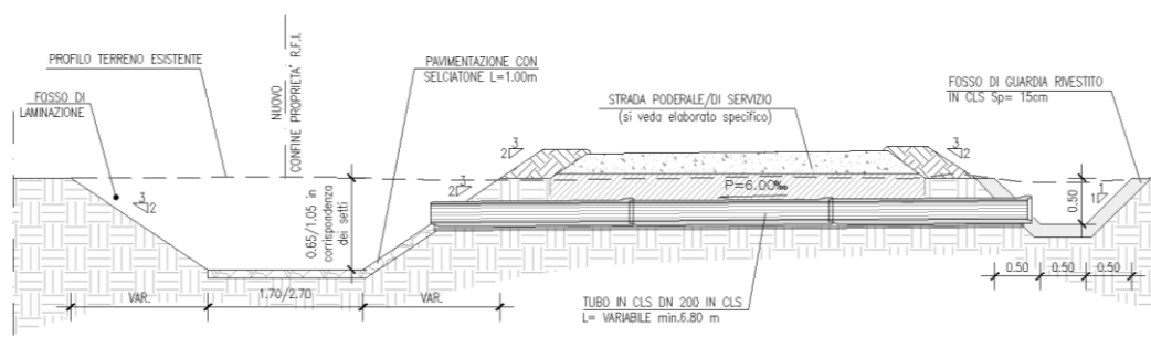
Dettaglio dello scarico del fosso di guardia verso quello di laminazione
