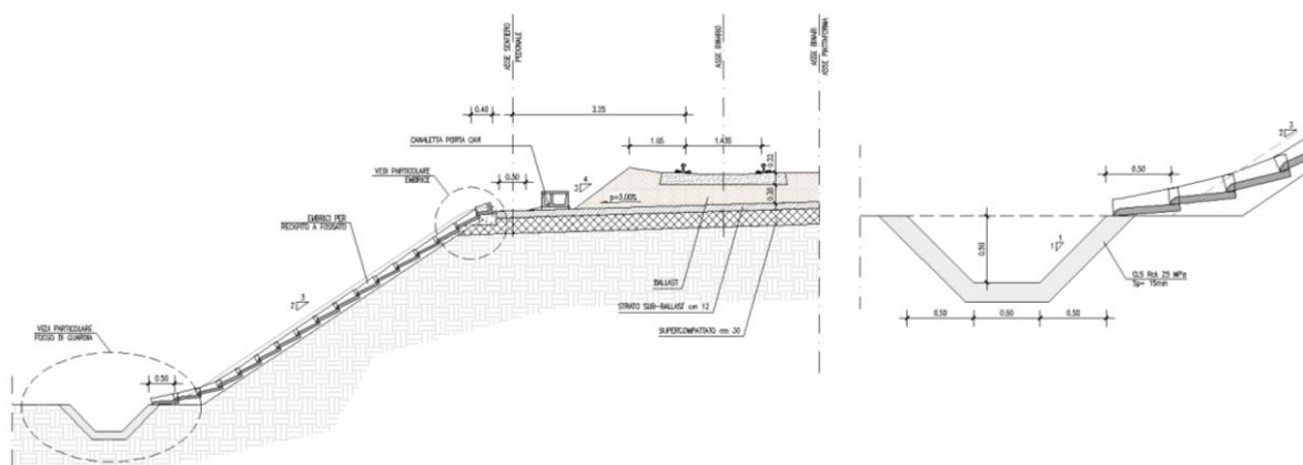
Schema di drenaggio acque di piattaforma in rilevato
