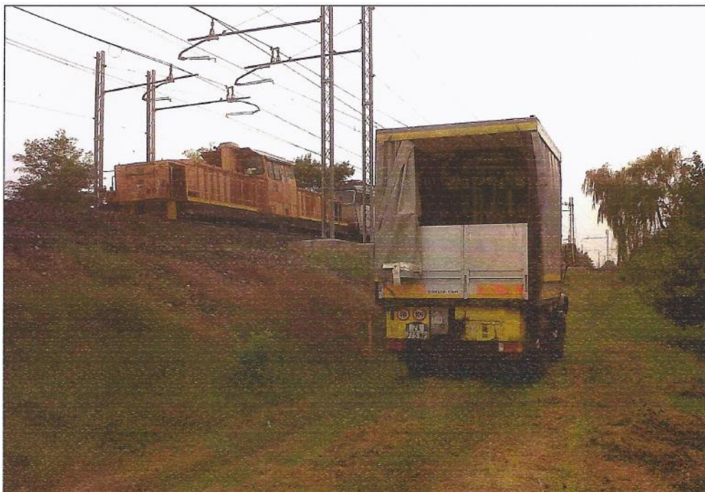
Foto 7 – Prova CPTU7
