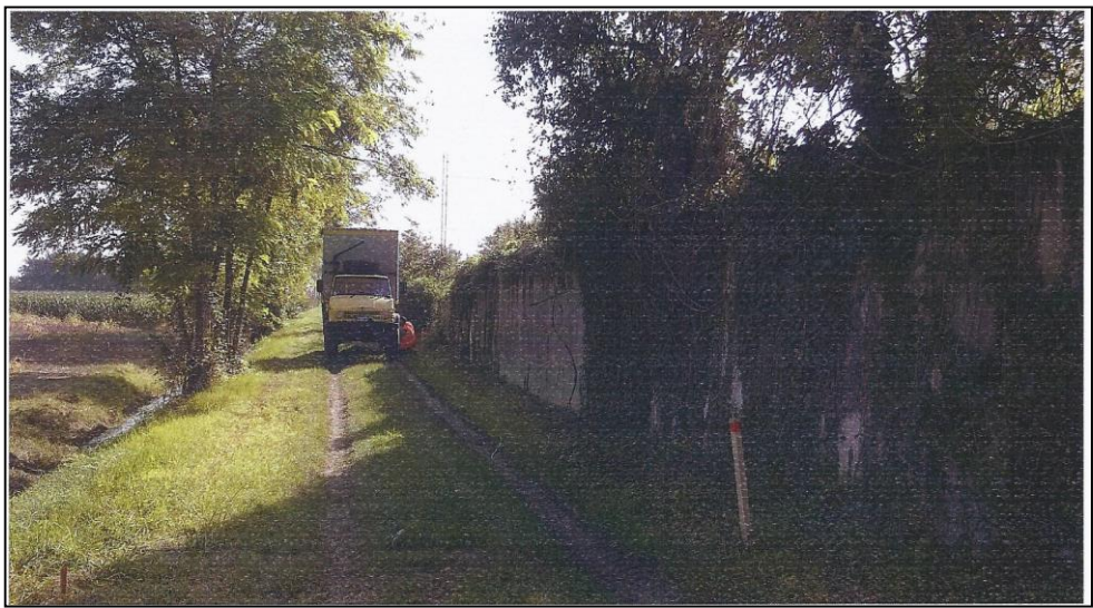
Foto 3 – Prova CPTU3
