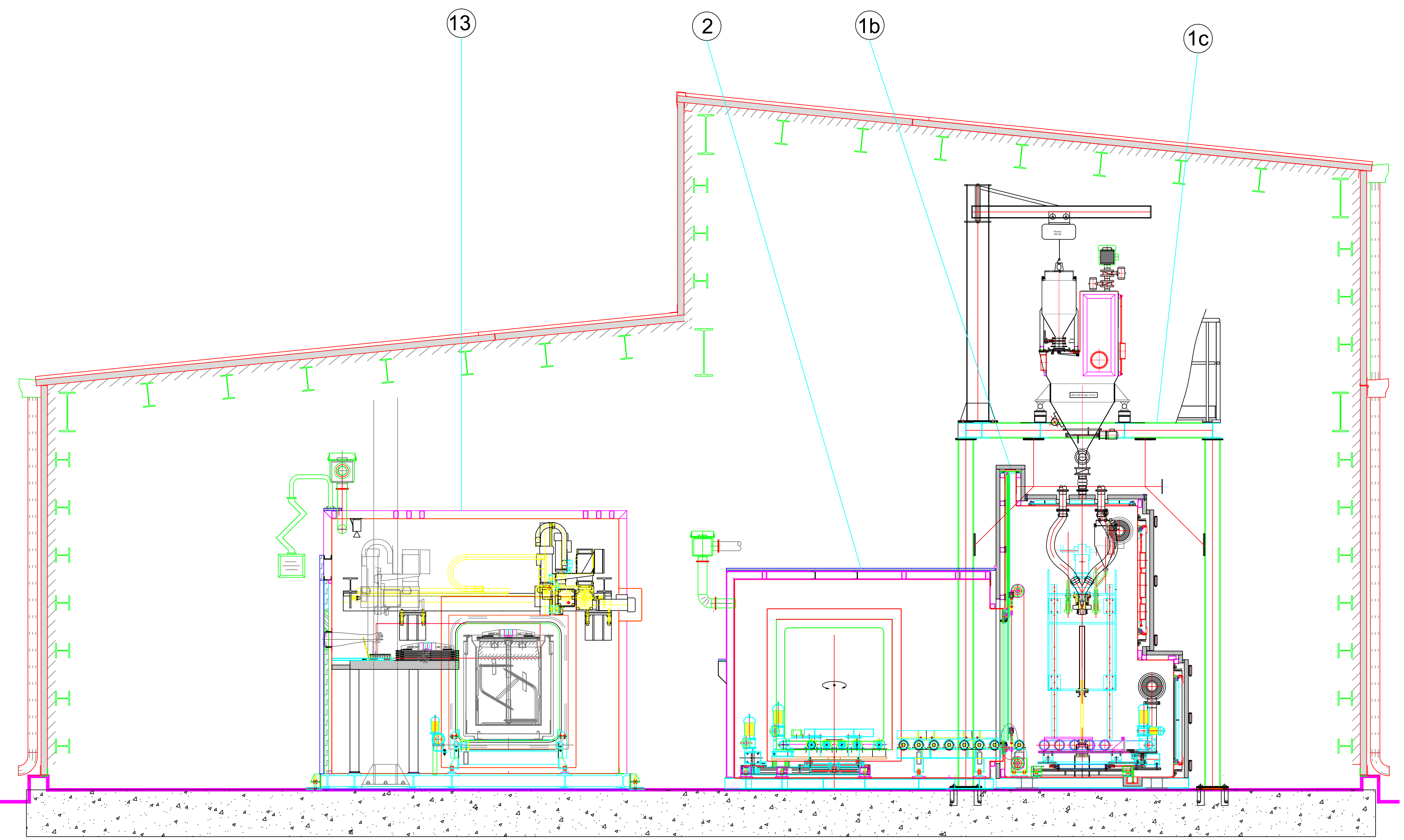
SEZIONE D-D SCALA 1:30
