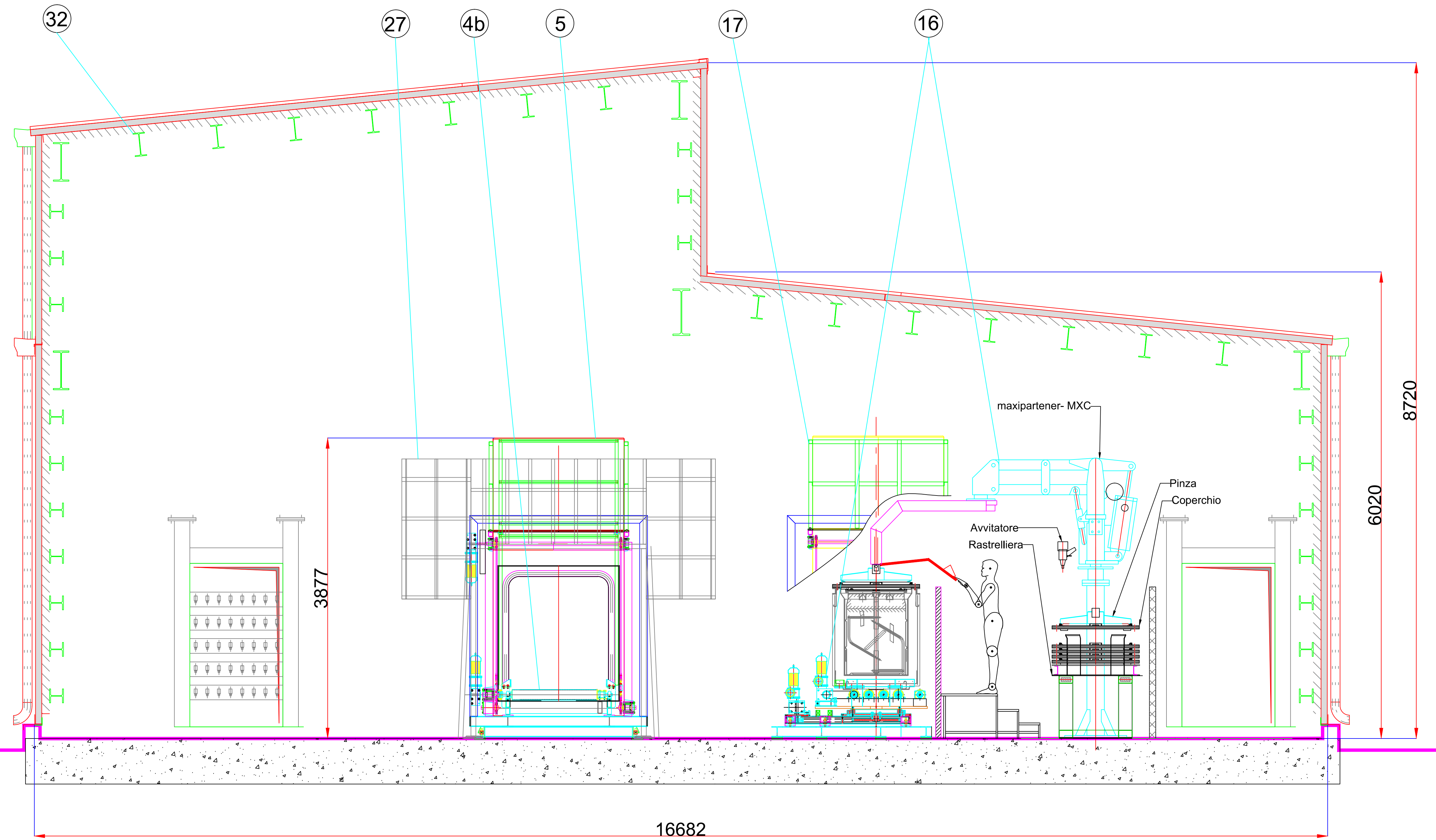
SEZIONE G-G SCALA 1:30
