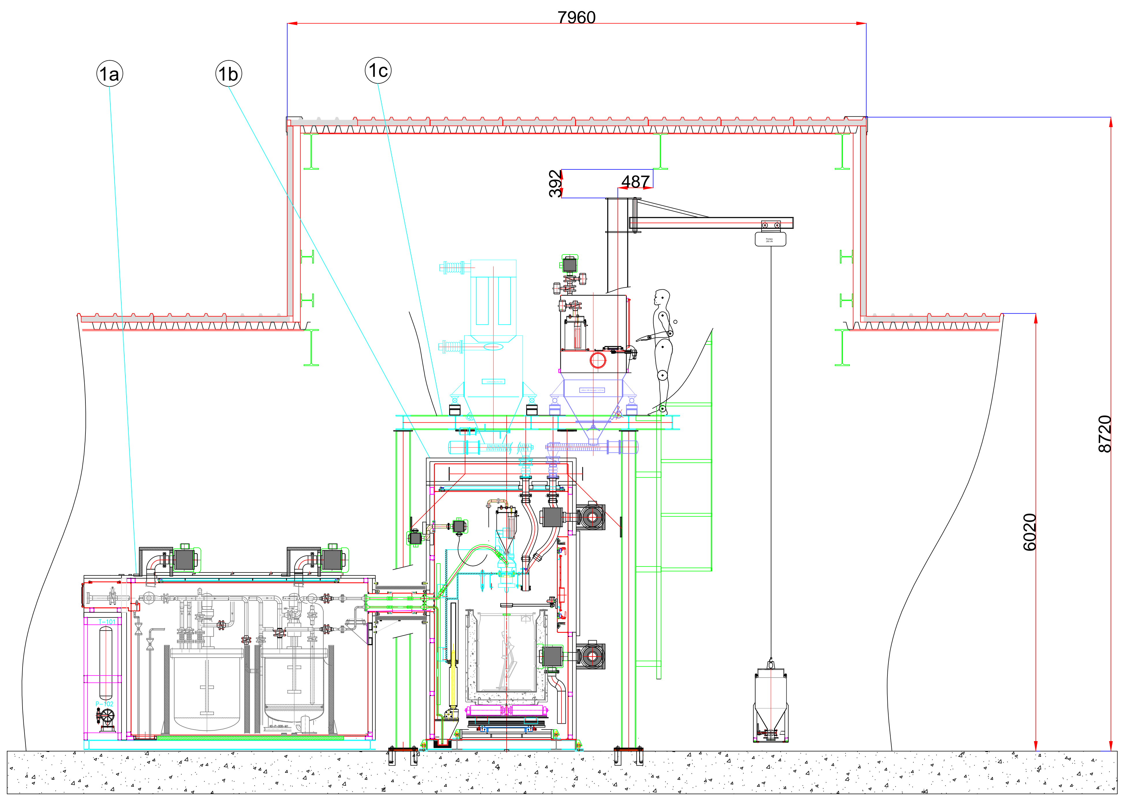
SEZIONE F-F SCALA 1:30
