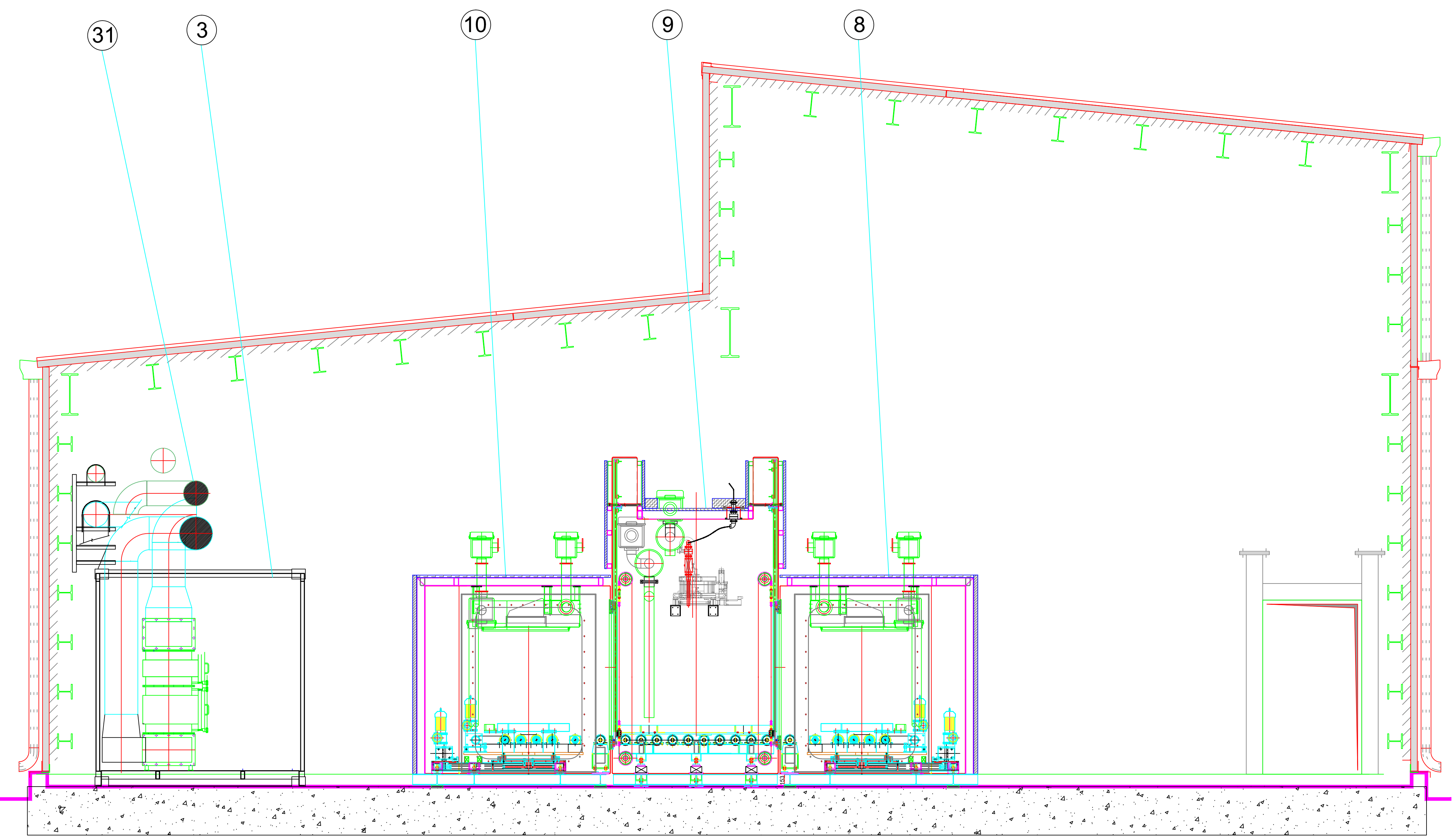
SEZIONE C-C SCALA 1:30
