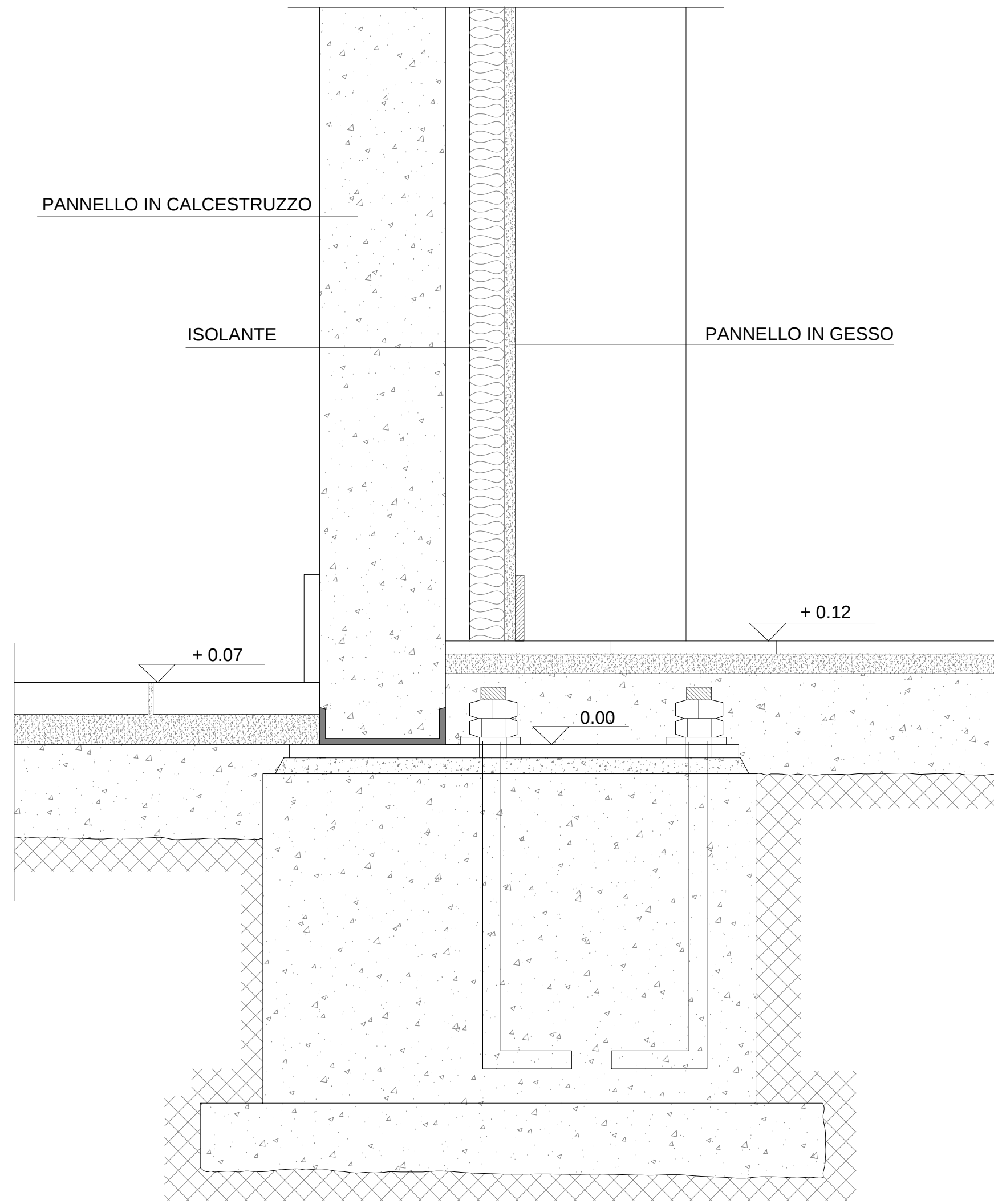
SEZIONE VERTICALE NODO PAVIMENTO
