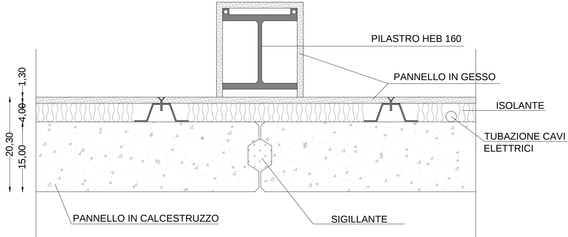
SEZIONE ORIZZONTALE
