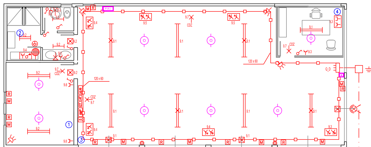
PIANTA EDIF SCALA 1:100
