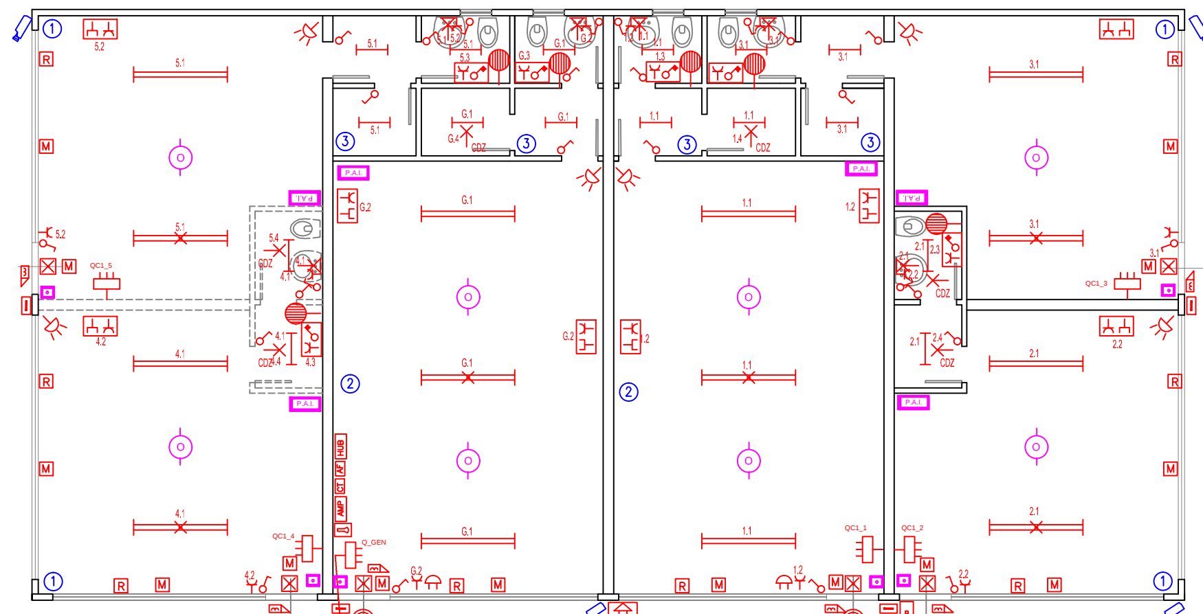
PIANTA EDIFICIO C.1 SCALA 1:100
