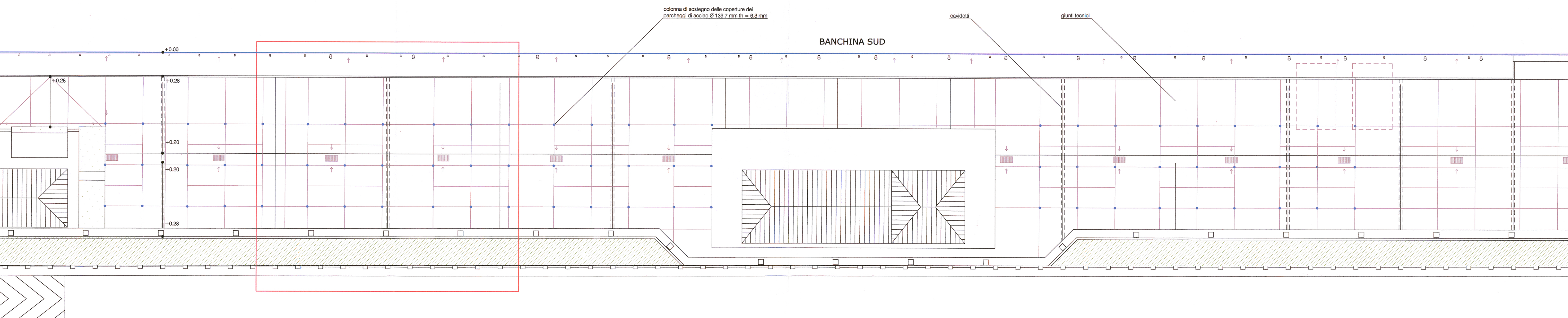
PLANIMETRIA DI DETTAGLIO DELL'AREA DEI PARCHEGGI DELLA BANCHINA SUD - SCALA 1:250
