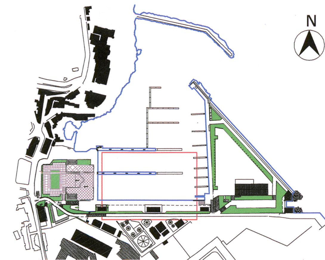
STRALCIO PLANIMETRICO
