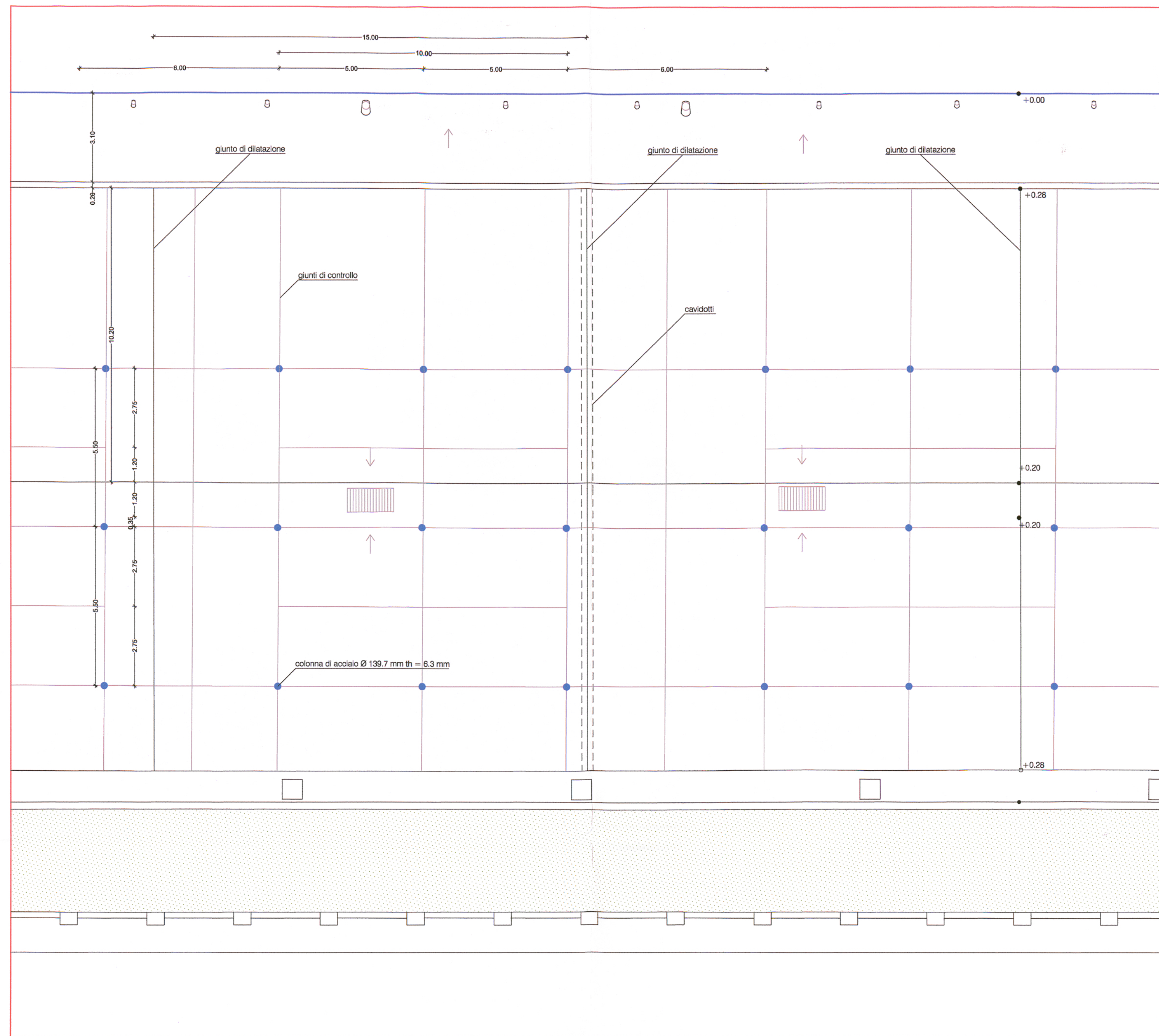
DETTAGLIO DI UNA PORZIONE DEI PARCHEGGI - SCALA 1:100
