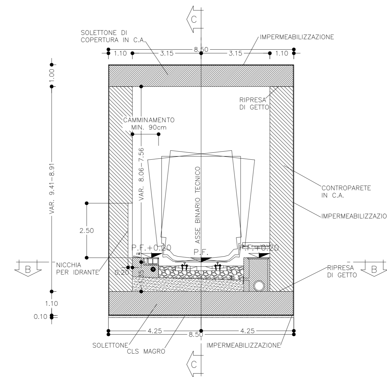
SEZIONE B-B SCALA 1:100 PIANTA
