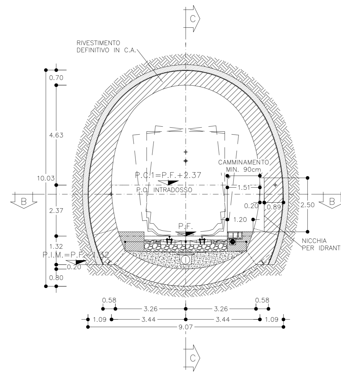
SEZIONE A-A SCALA 1:100 PROFILO NICCHIA
