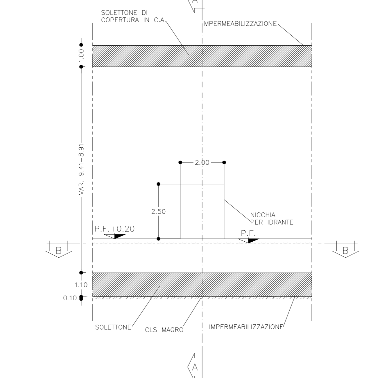
SEZIONE C-C SCALA 1:100 PROFILO NICCHIA
