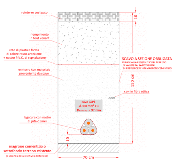
Figura 2-19 Sezione tipica di posa del tratto di cavidotto terrestre in corrente alternata, su terreno naturale
