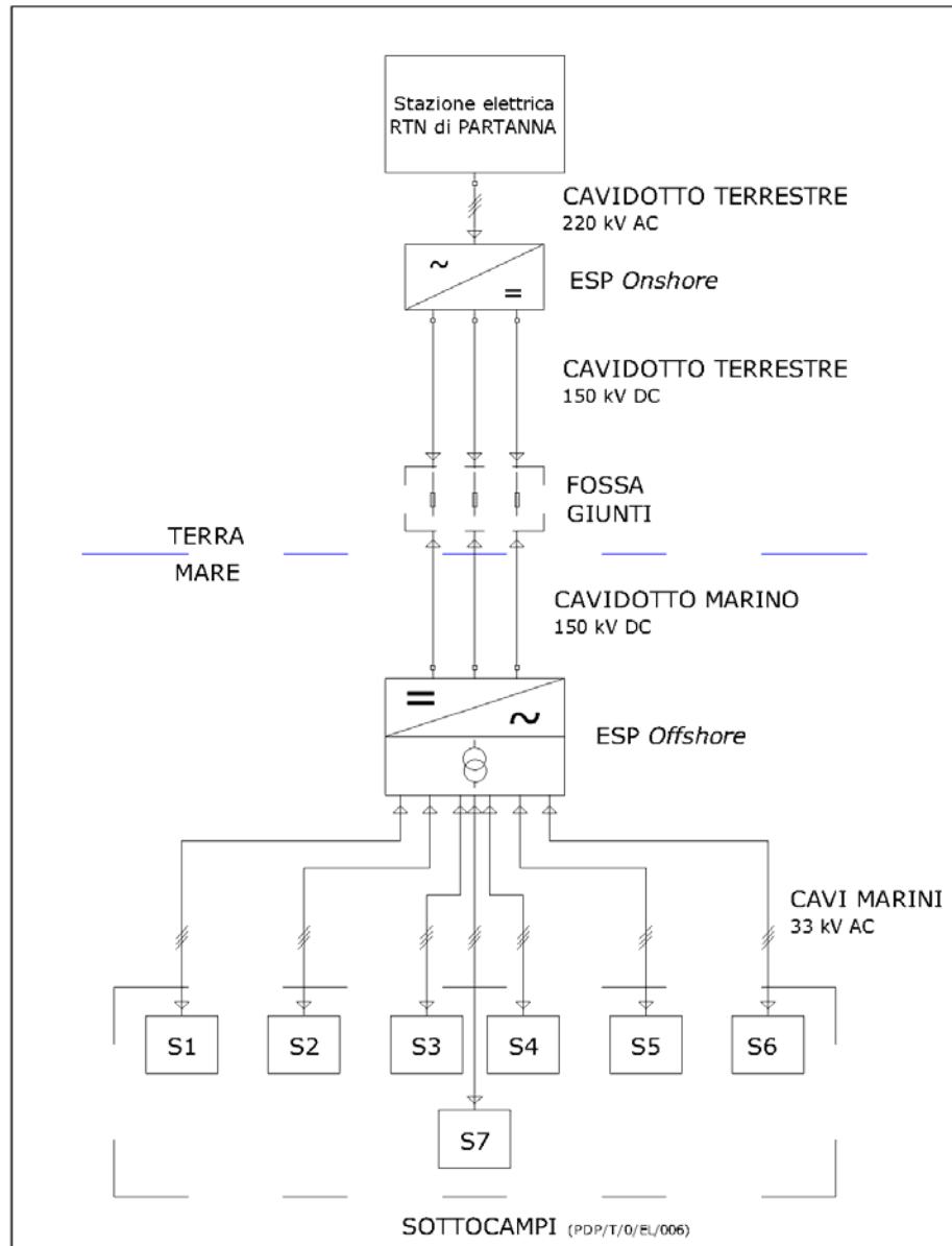
Figura 2-2 schema a blocchi semplificato dell'impianto
