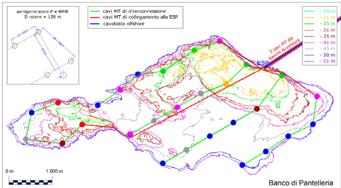
Figura 2-9 Banco di Pantelleria: layout impianto
