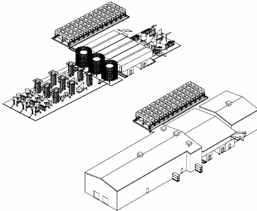
Figura 2-20 Layout tipico di un impianto da 350 MW di dimensioni 80x25x11,5 metri
