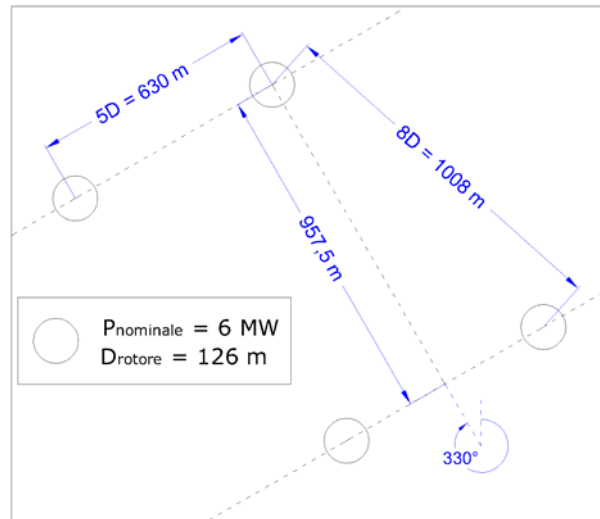
Figura 2-7 Criterio generale di disposizione degli aerogeneratori
