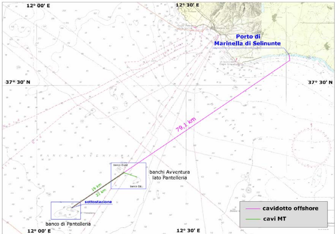
Figura 2-8 Percorso del cavidotto marino e dei cavi MT di collegamento dai Banchi Avventura – lato Pantelleria alla sottostazione elettrica offshore
