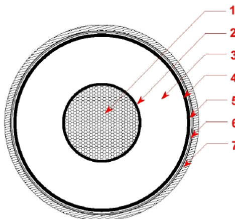
Figura 2-18 Sezione tipica del cavo XLPE: 1) conduttore; 2) schermo del conduttore; 3) isolamento; 4) schermo isolante; 5) barriera antiacqua; 6) schermo metallico esterno; 7) guaina esterna
