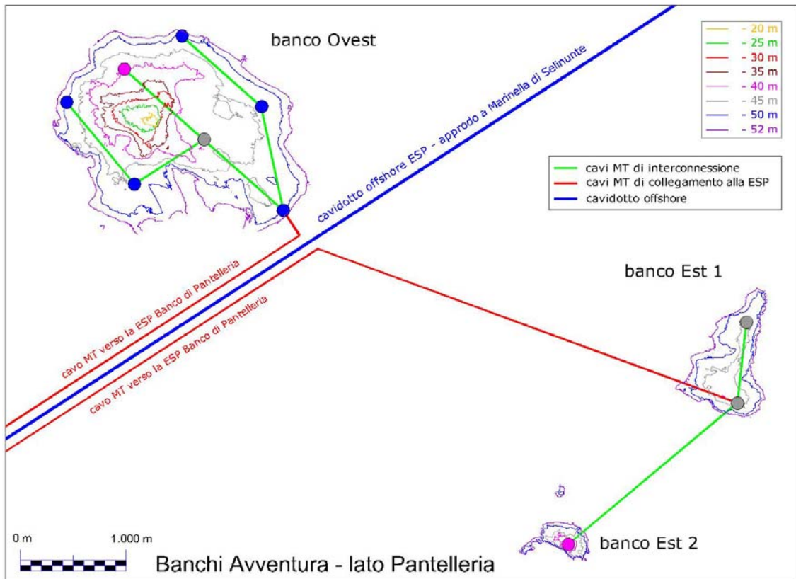
Figura 2-10 Banchi Avventura – lato Pantelleria: layout impianto
