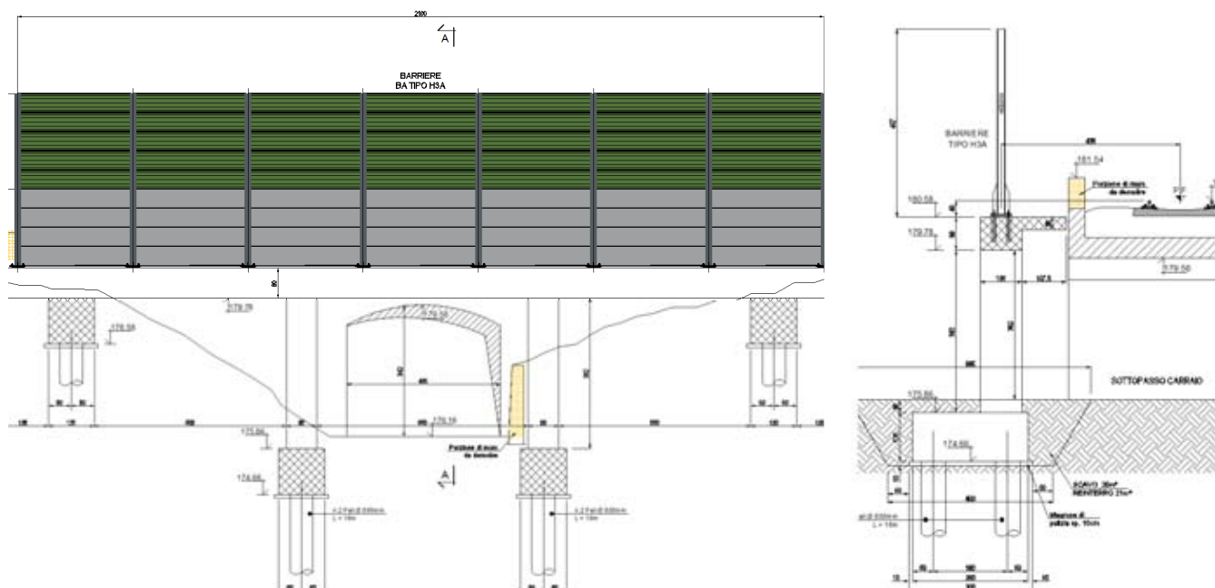
Figura 5-25 Prospetto della barriera realizzata su Opere di scavalco sottovia PK109+570
