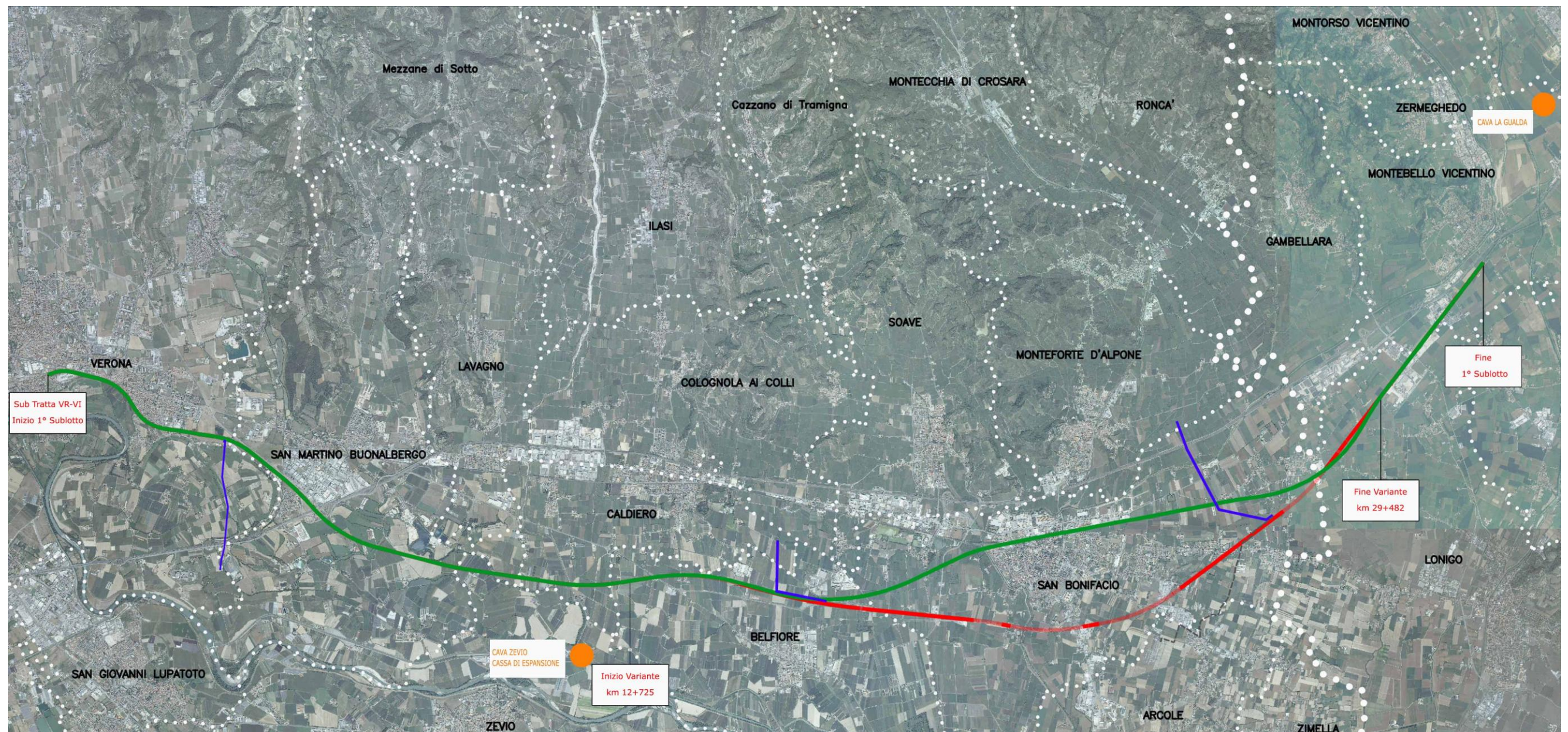
Figura 1— Corografia “Opere in variante” del 1° sublotto Verona - Montebello Vicentino
