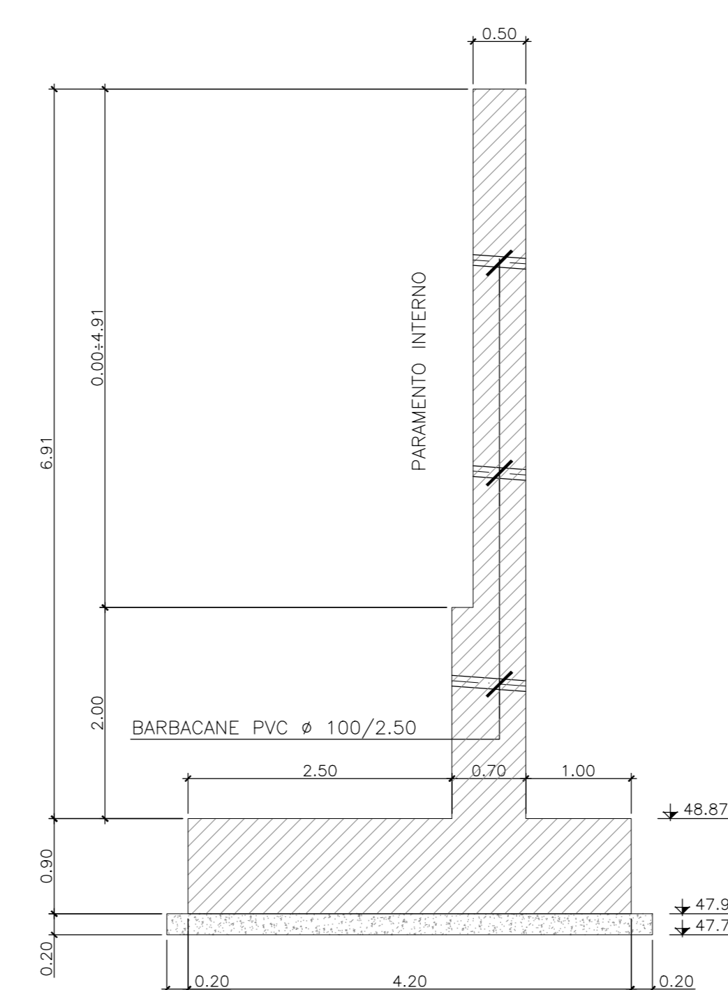
SEZIONE MURO TIPO "A1" 1:50
