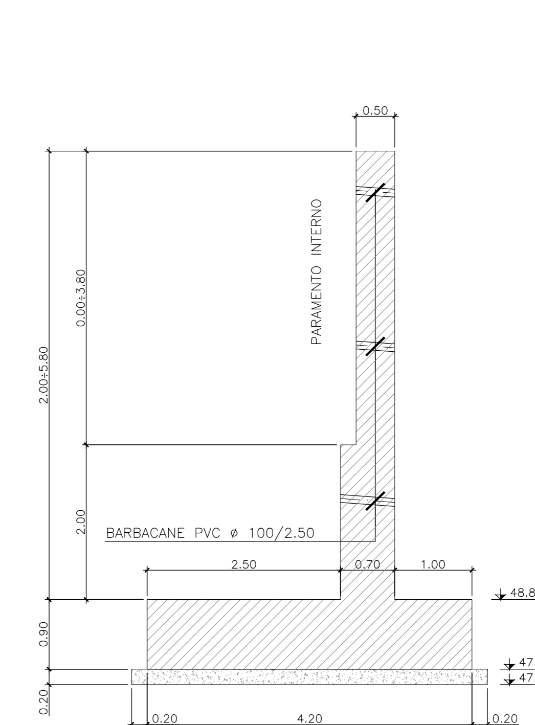
SEZIONE MURO TIPO "A2" 1:50
