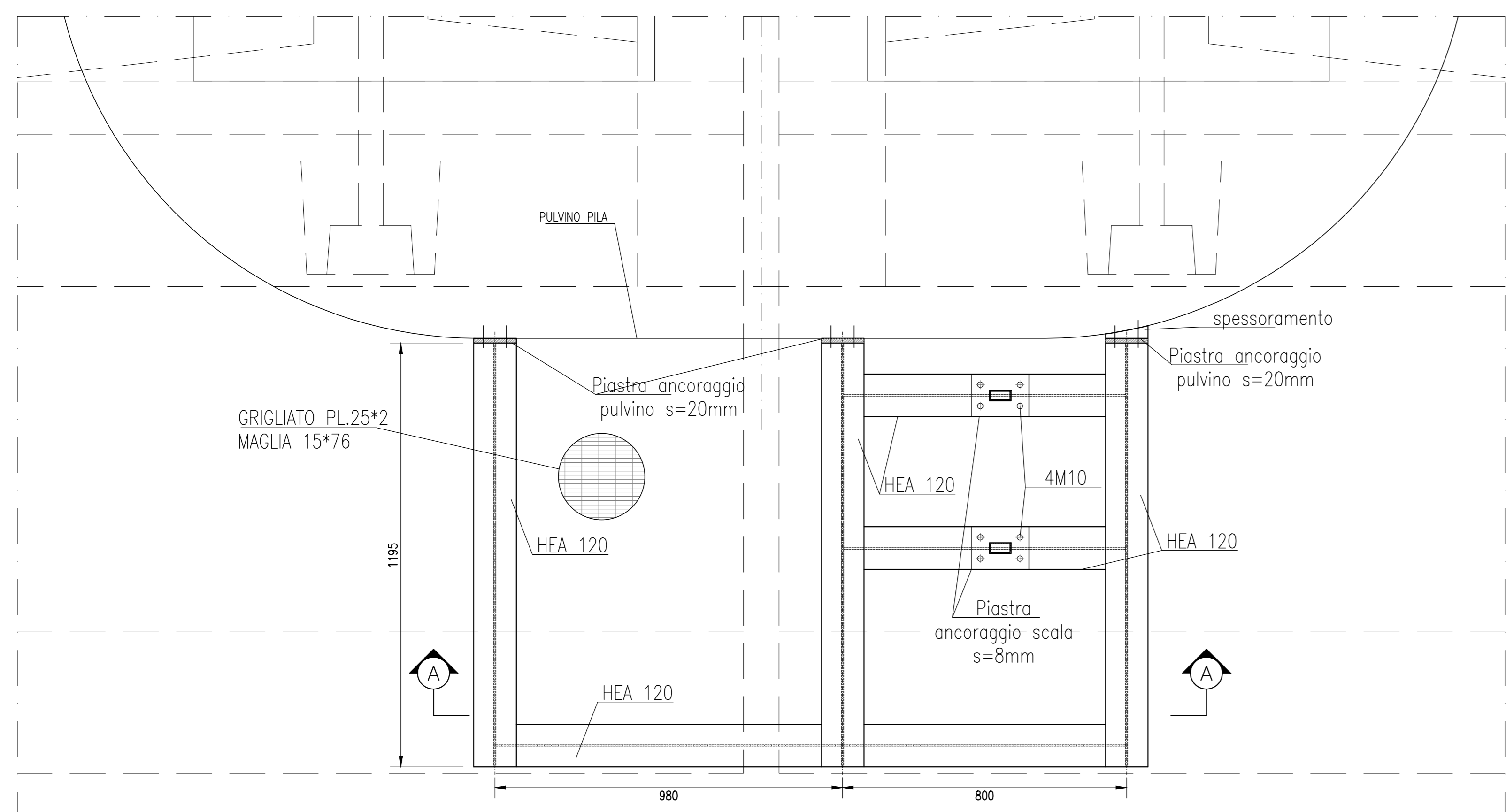
PIANTA QUOTA PULVINO scala 1:10
