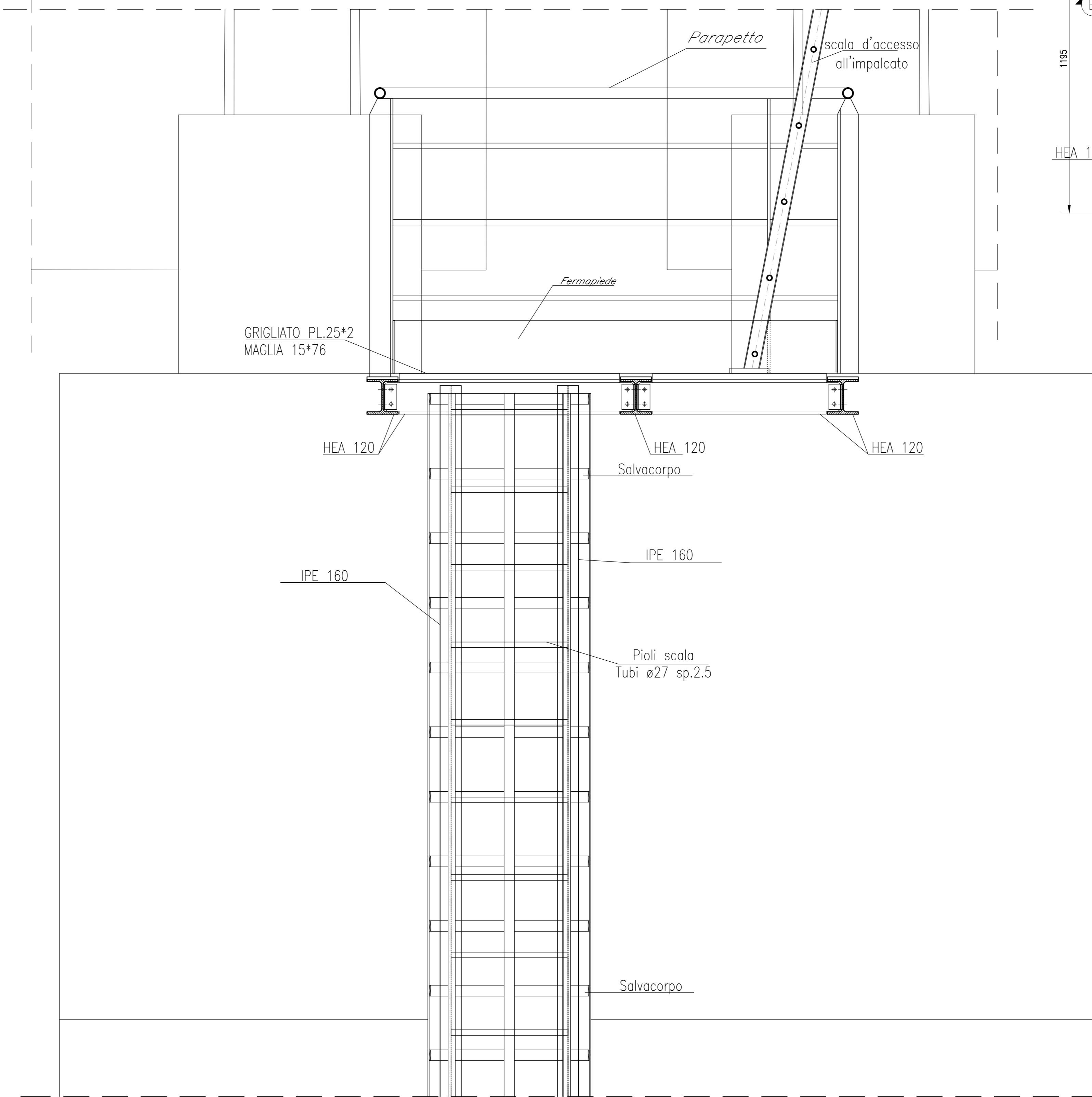
SEZIONE B-B scala 1:10
