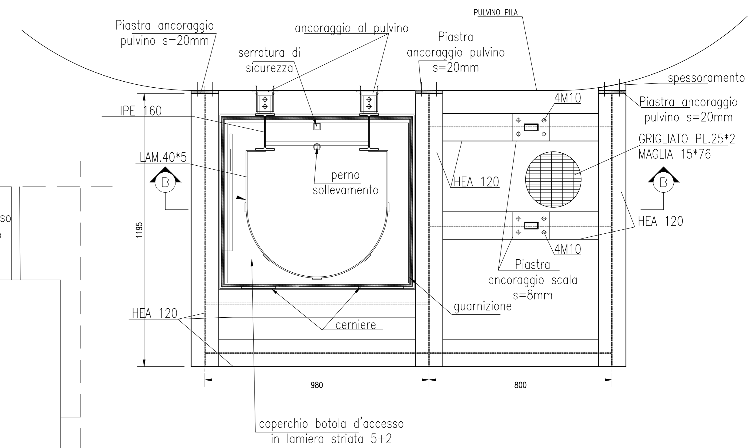
PIANTA QUOTA PULVINO scala 1:10
