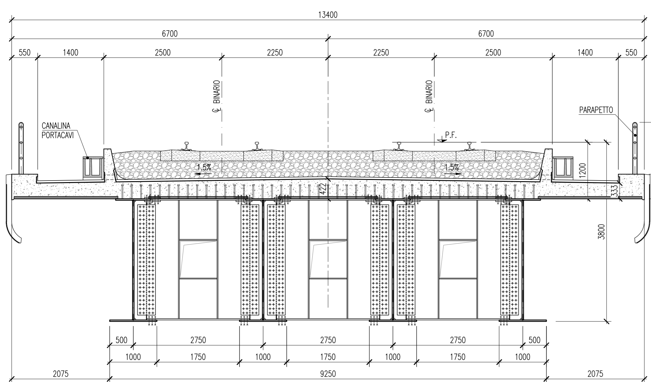
SEZIONE A-A (DIAFRAMMA TIPO 1) SCALA 1:50
