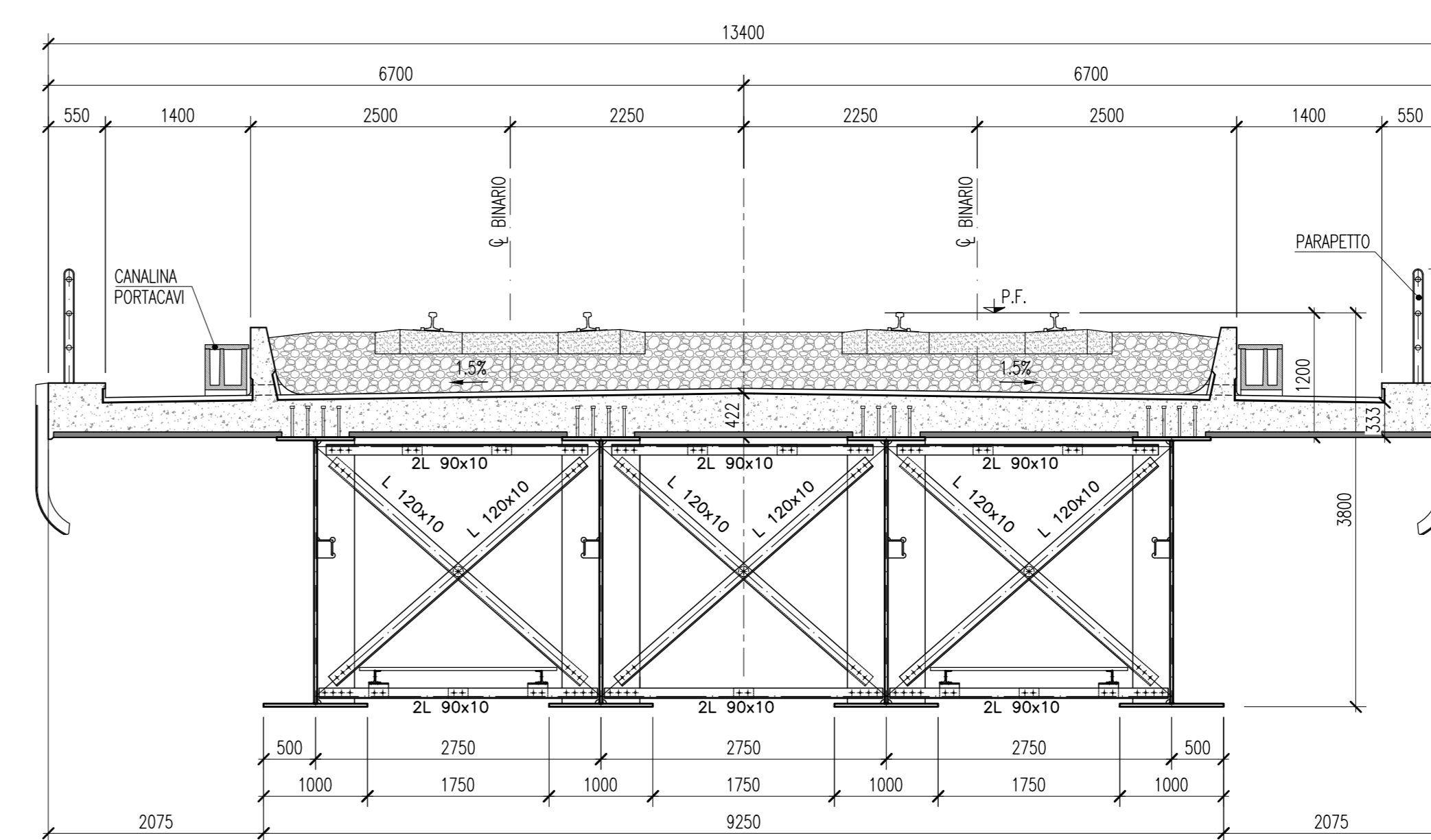
SEZIONE C-C (DIAFRAMMA TIPO 3) SCALA 1:50
