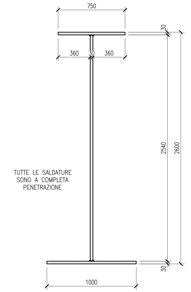
TRAVE LONG. TIPO B
