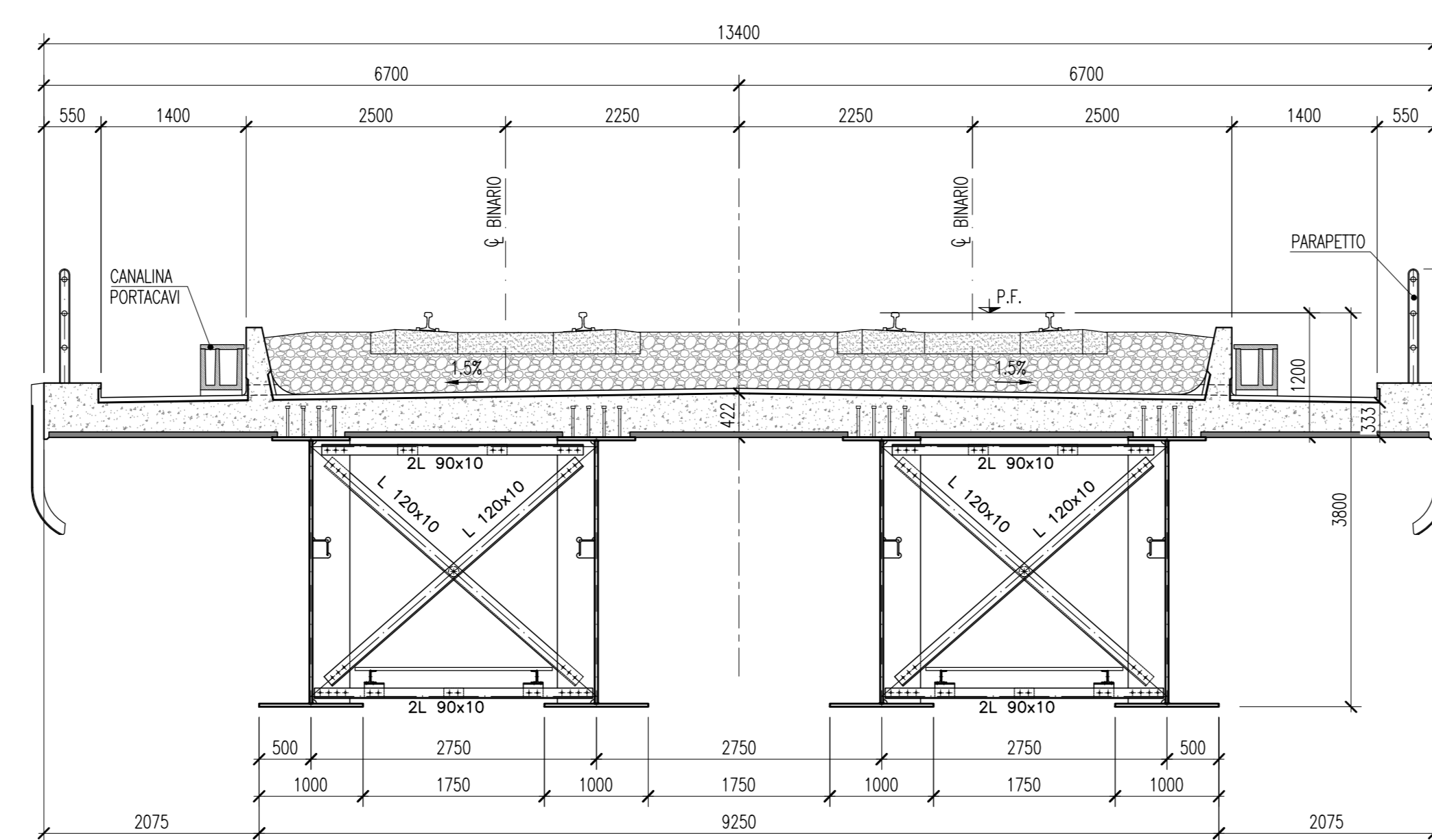
SEZIONE B-B (DIAFRAMMA TIPO 2) SCALA 1:50
