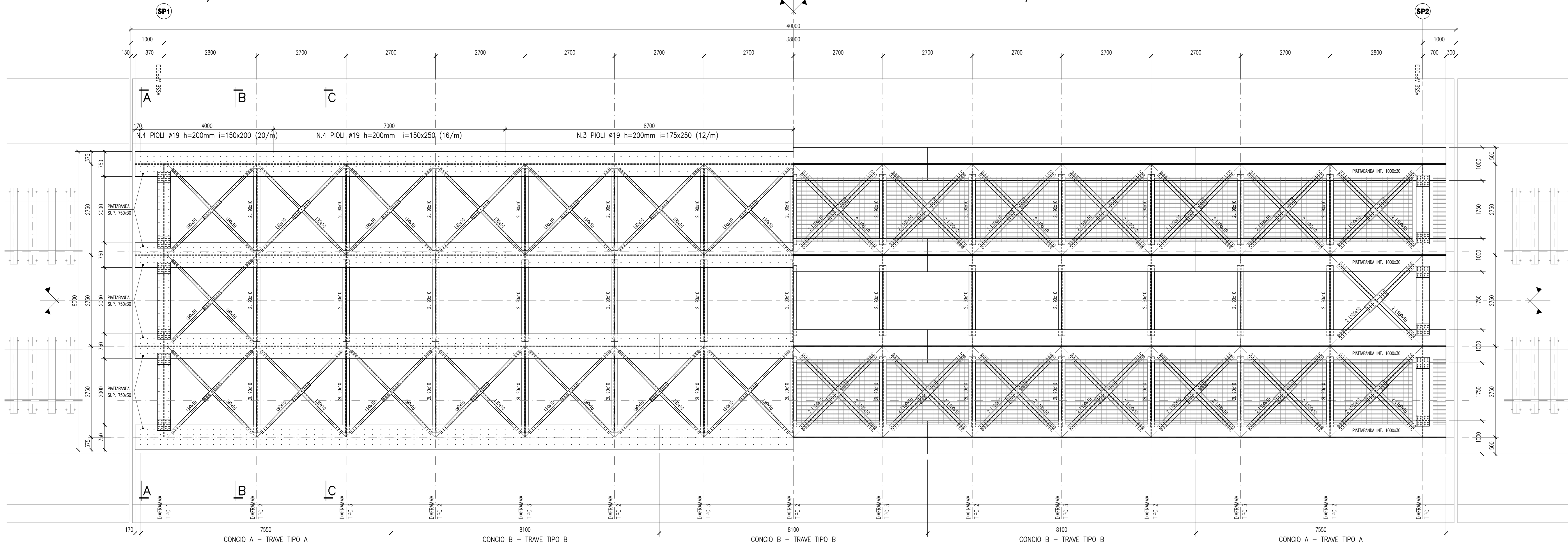
1/2 PIANTA PIATTABANDA SUPERIORE SCALA 1:50
