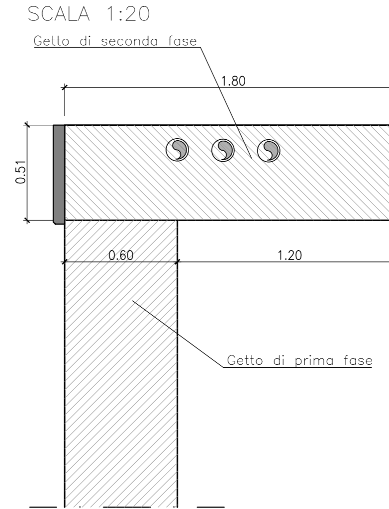
DETTAGLIO 1 SCALA 1:20
