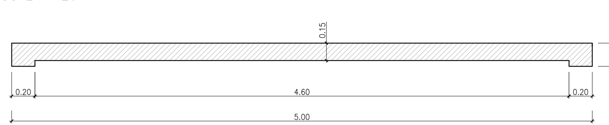
CARPENTERIA SOLETTA BASCULANTE SCALA 1:20
