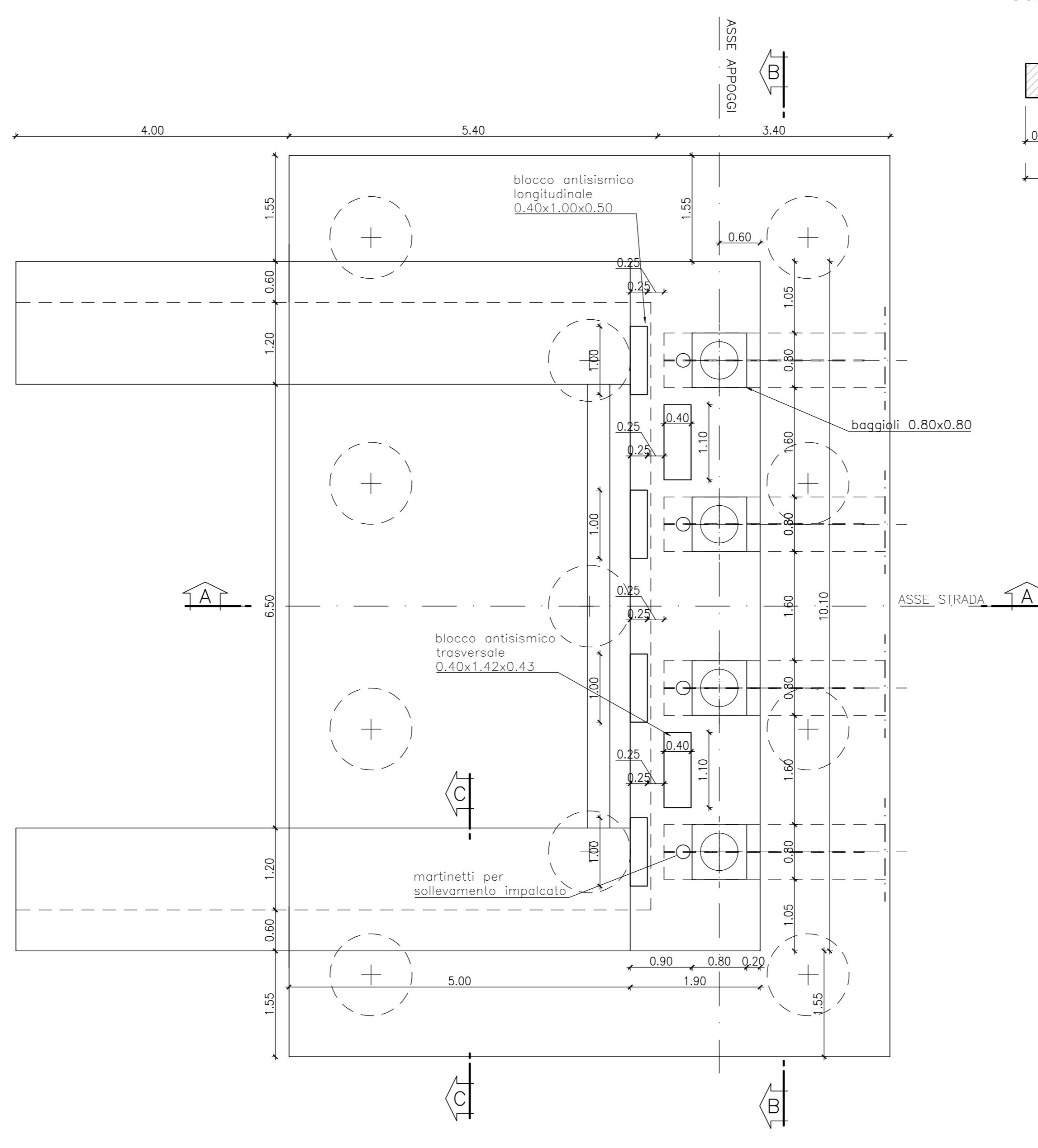
VISTA DALL'ALTO SCALA 1:50
