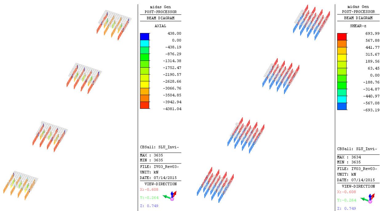
Figura 36: Combinazione SLU SISMA: – Involuppo Sforzo Normale e tagli
