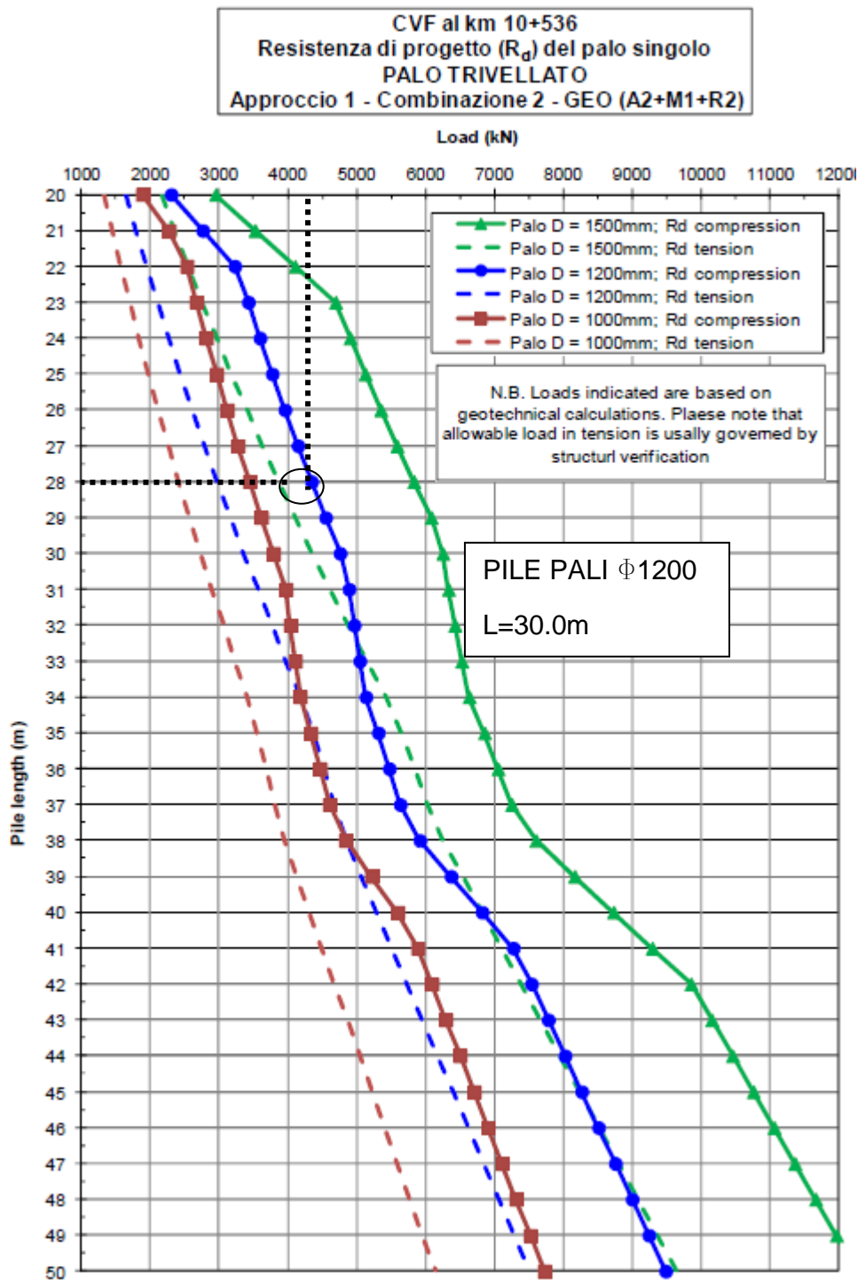
Figura 38: Approccio 1 Combinazione 2 – A2M1R2: Resistenza di progetto
