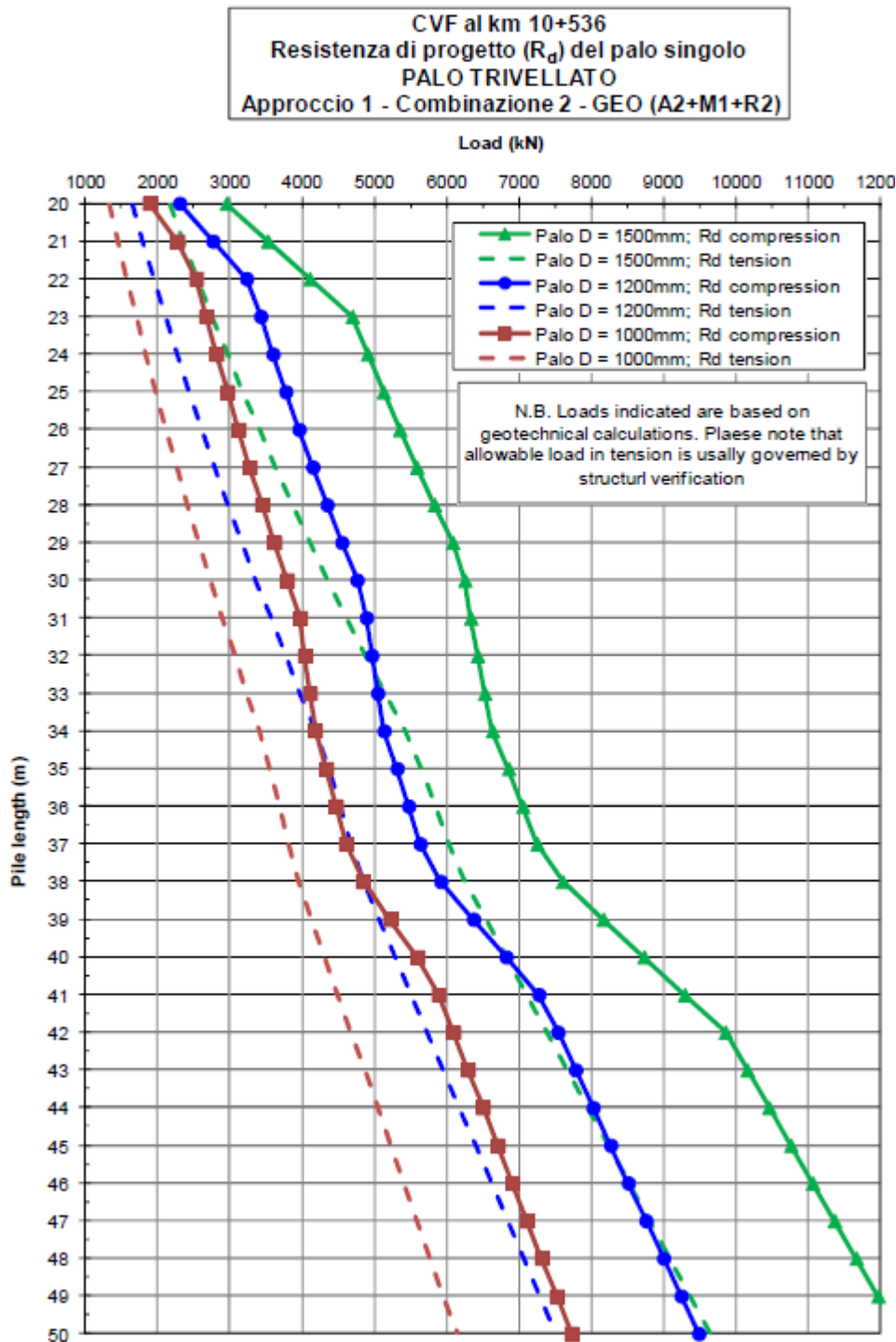
Figura 34: Approccio 1 Combinazione 1 - A1M1R1: Resistenza di progetto
