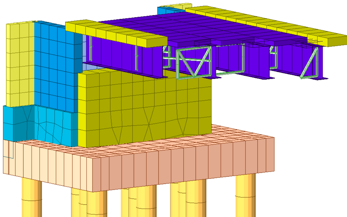
Figura 31: Modellazione tridimensionale Elementi finiti – spalla
