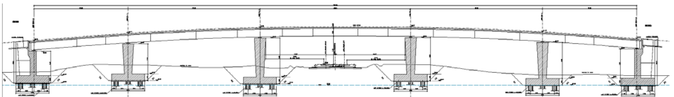
Figura 3: Profilo longitudinale
