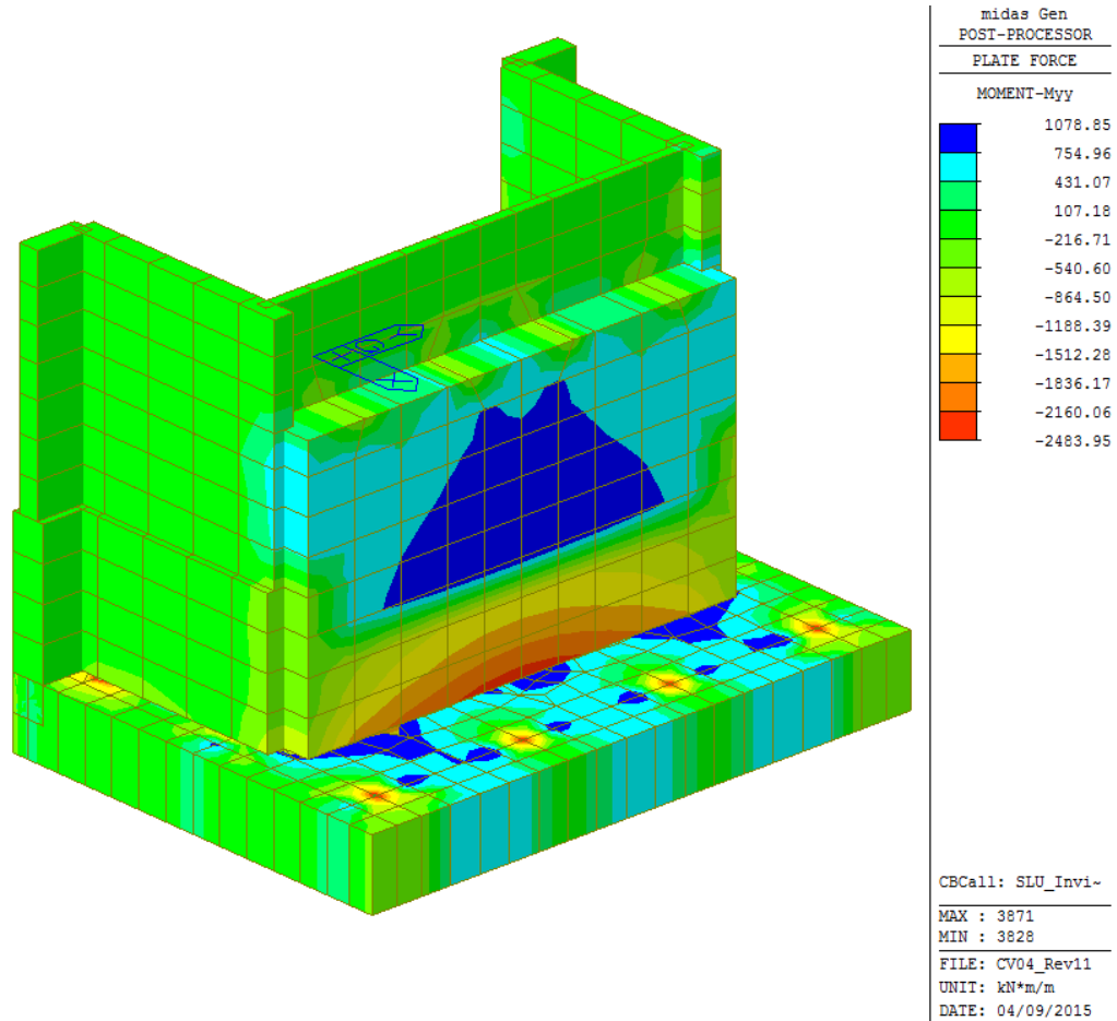
Figura 37: Combinazione involucro Sisma all - Momenti Myy
