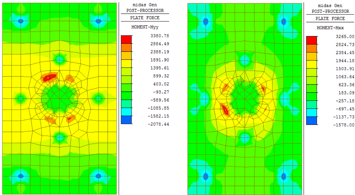
Figura 42 Comb. SISMA: – Involuppo Momenti Mtrasv (a sinistra) ;Mlong (a destra)
