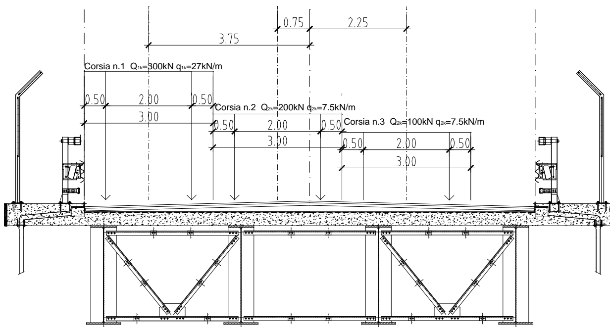
Figura 14: Disposizione delle colonne di carico sull'impalcato
