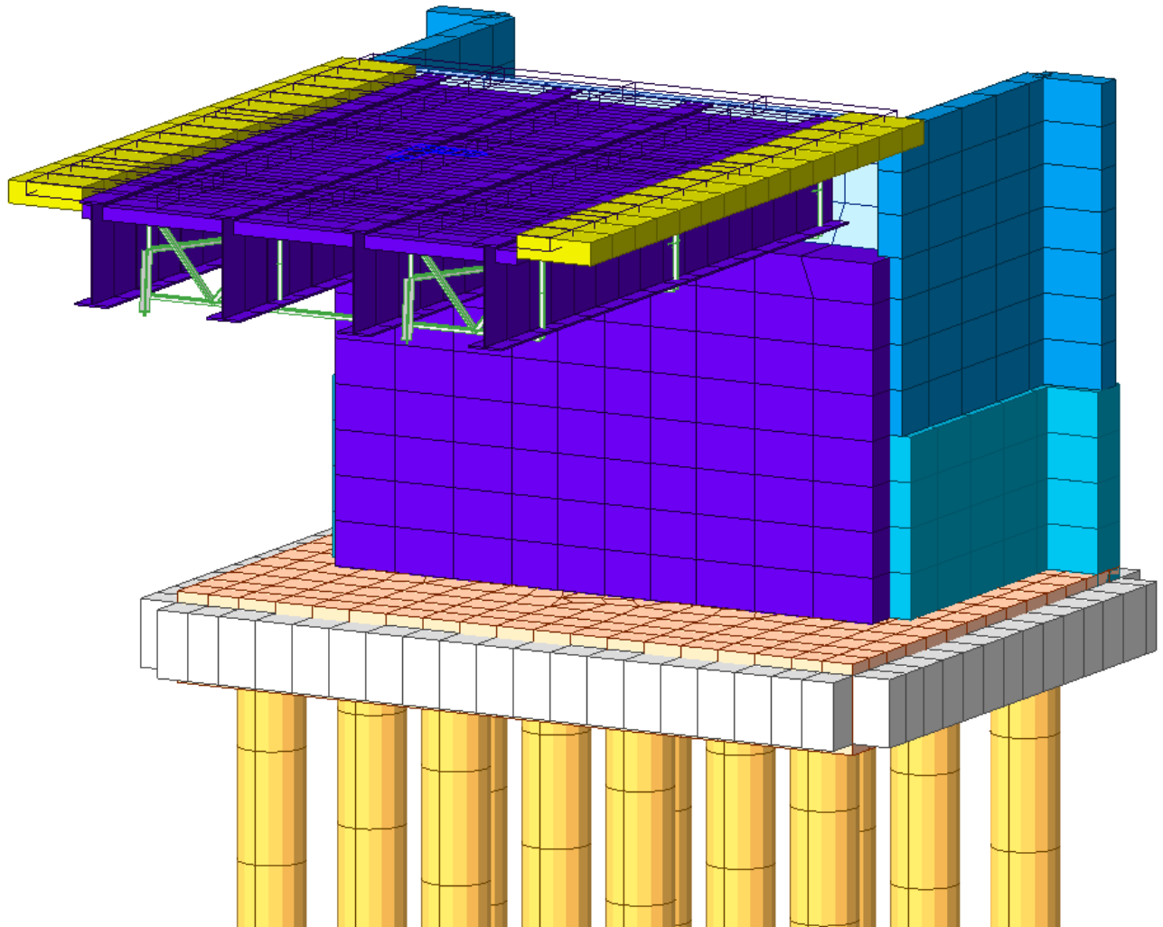
Figura 31: Modellazione tridimensionale Elementi finiti – spalla
