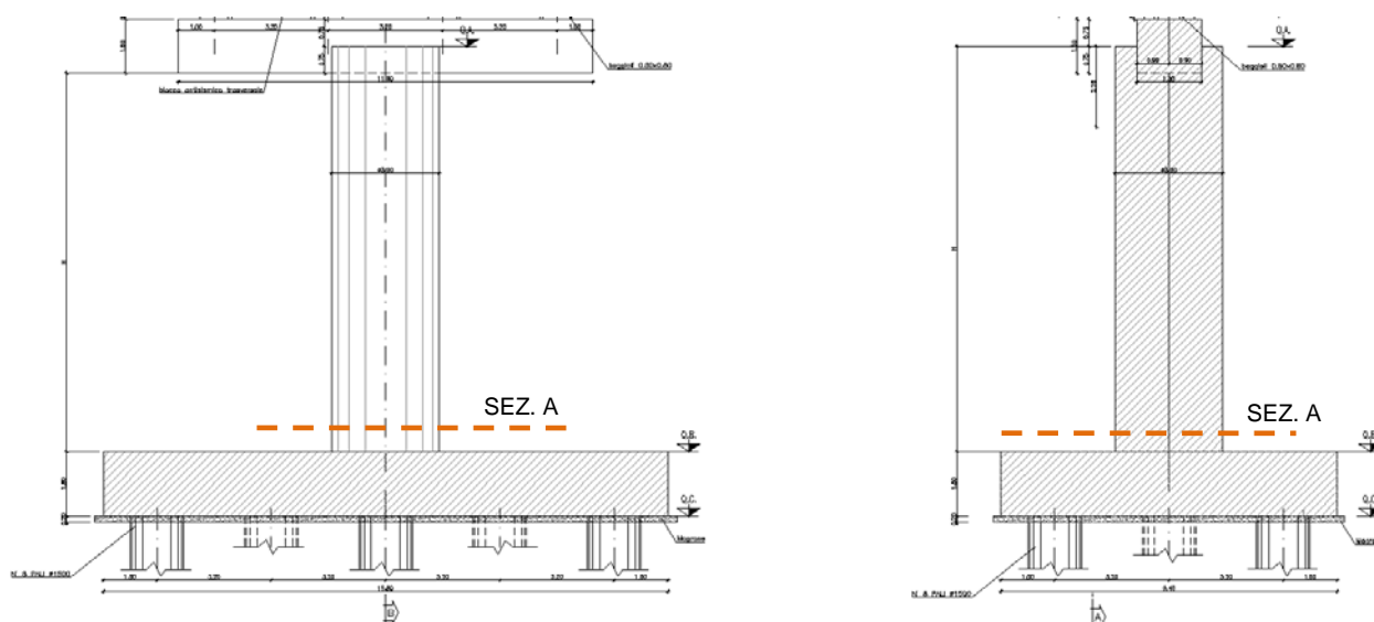
Figura 39: Identificazione delle sezioni di calcolo
