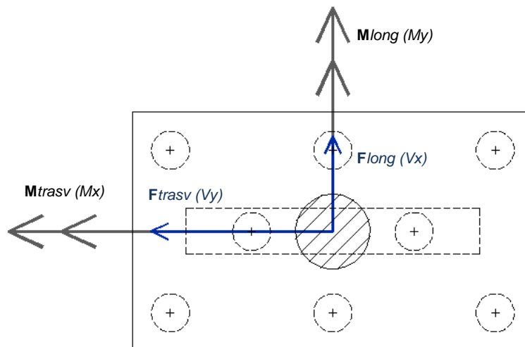
Figura 40: Indicazione delle direzioni di azione delle sollecitazioni sulla pila
