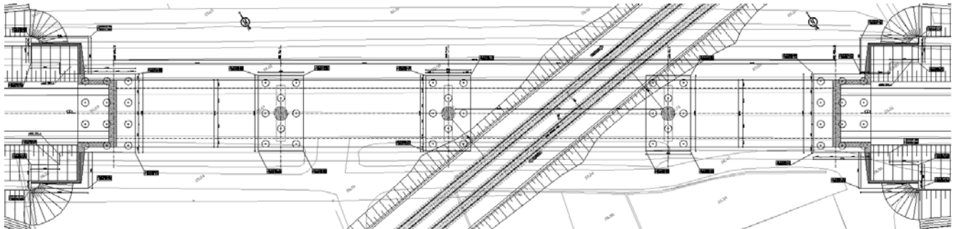
Figura 2: Pianta fondazioni
