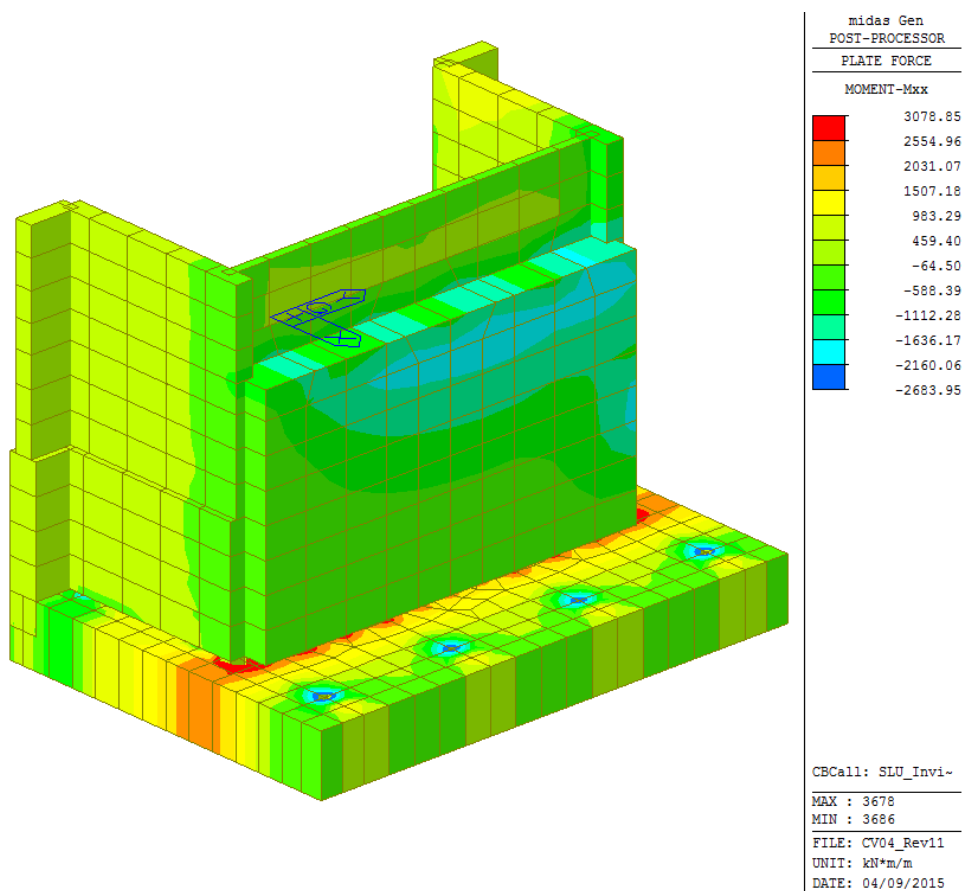
Figura 36: Combinazione involucro Sisma all - Momenti M_{xx}
