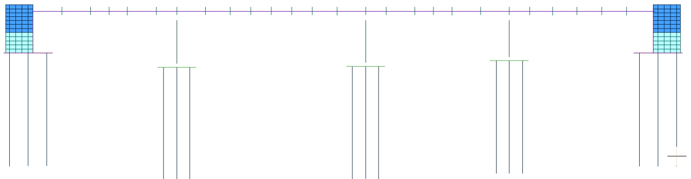
Figura 32: Modellazione tridimensionale Elementi finiti – prospetto longitudinale
