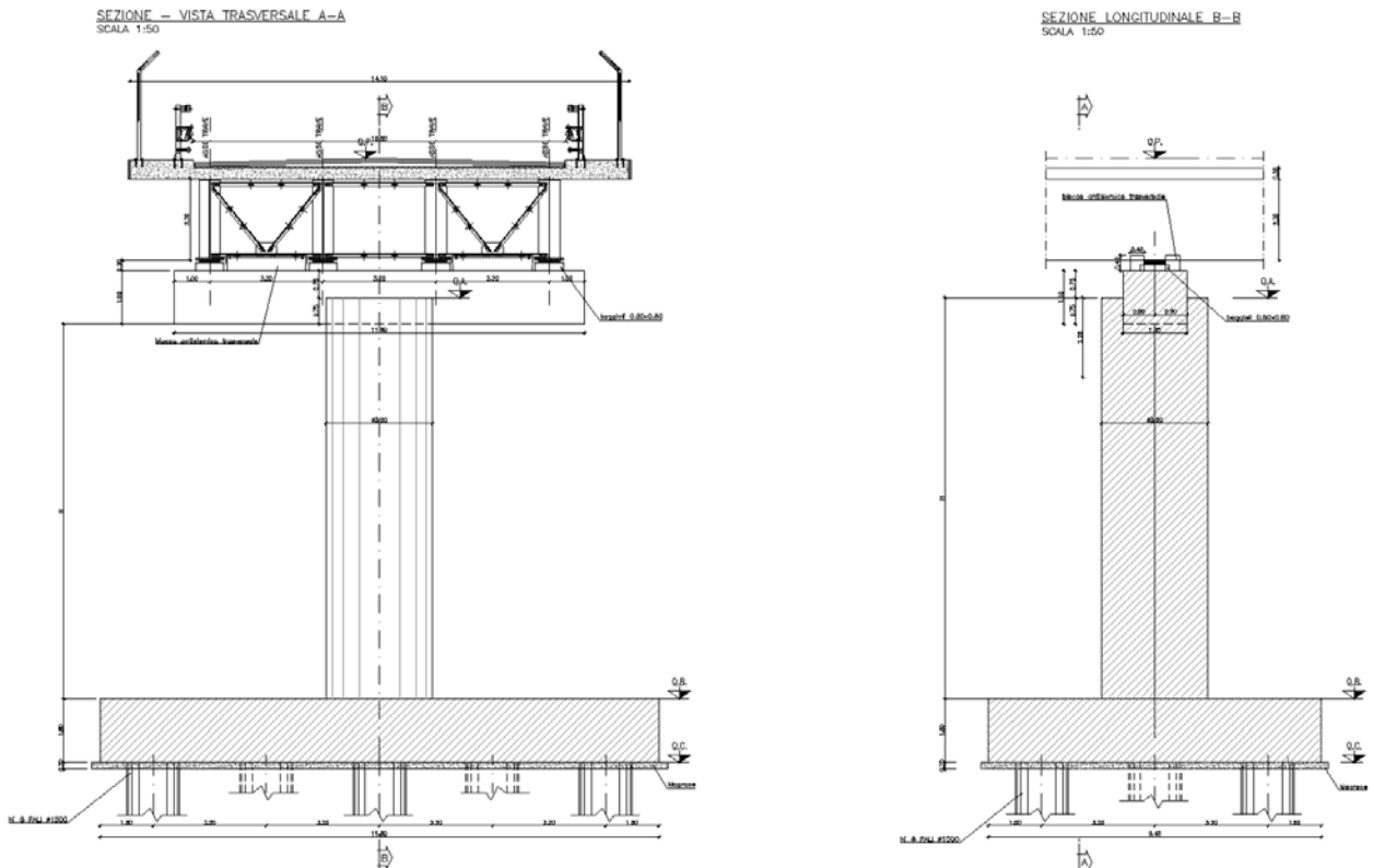
Figura 6: Carpenteria pile
