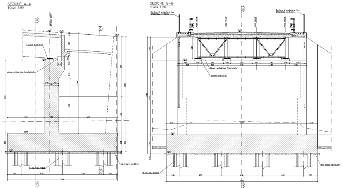
Figura 5: Carpenteria spalla B
