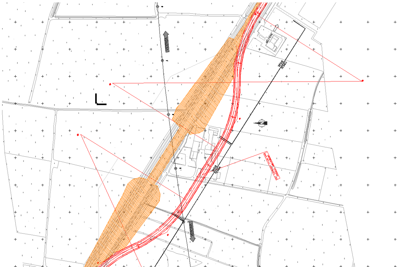
Figura 9: Deviazione provvisoria
