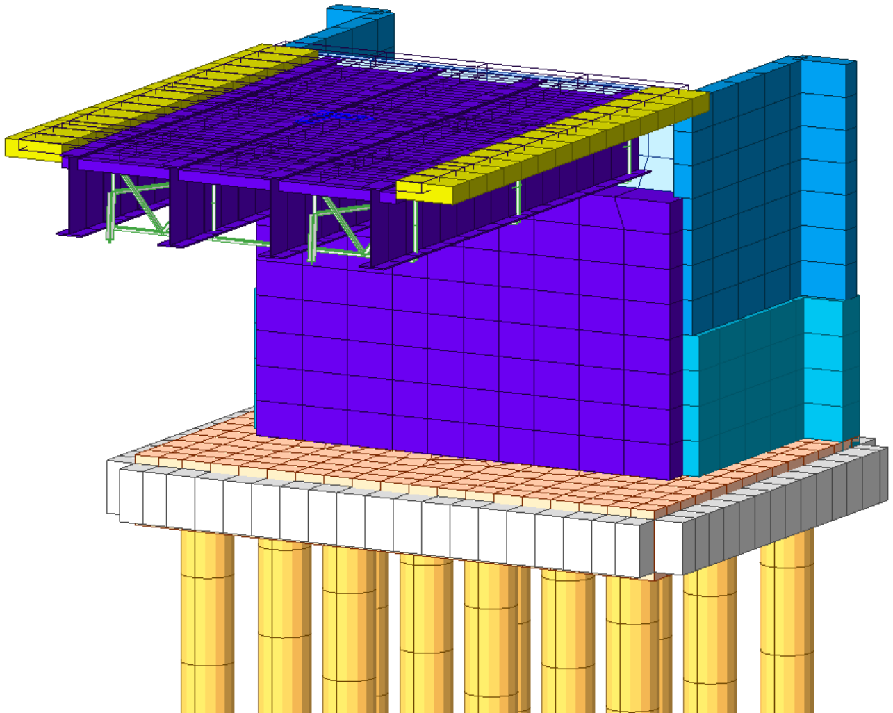
Figura 31: Modellazione tridimensionale Elementi finiti – spalla
