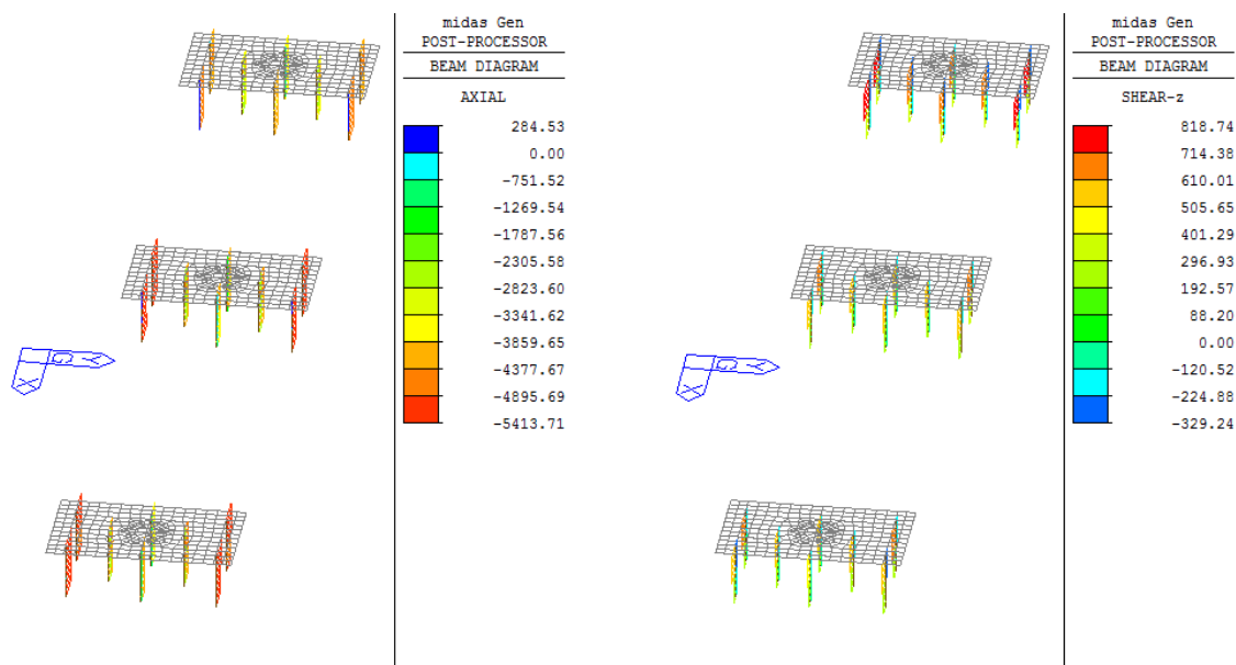
Figura 37: Combinazione SLU SISMA: – Involuppo Sforzo Normale e tagli
