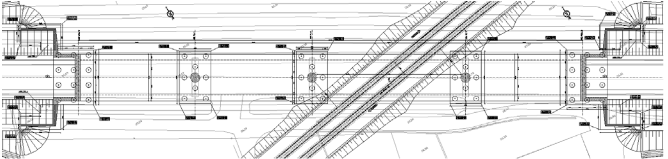
Figura 2: Pianta fondazioni
