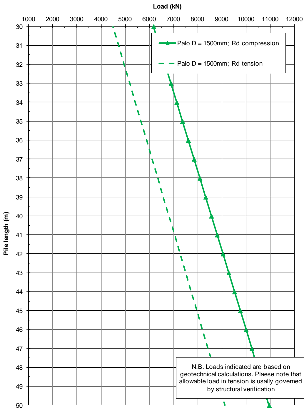
Figura 39: Approccio 1 Combinazione 2 – A2M1R2: Resistenza di progetto
