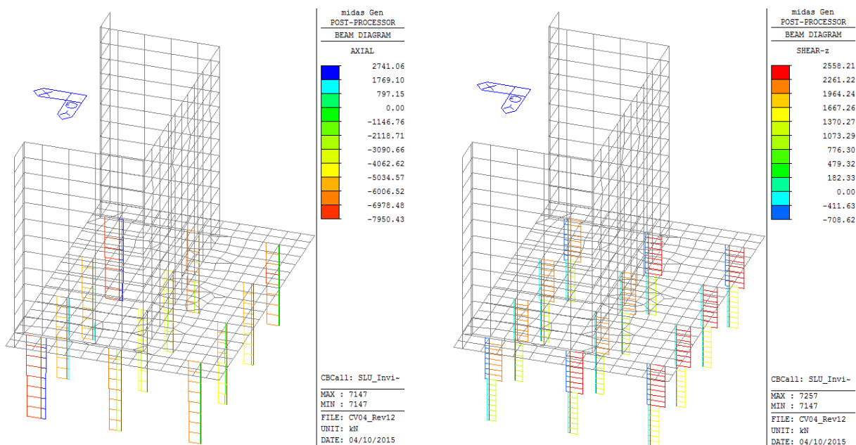
Figura 34: Combinazione SLU SISMA: – Involuppo Sforzo Normale e tagli
