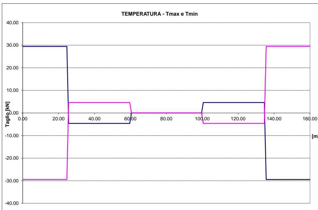
Figura 40 – Temperatura
