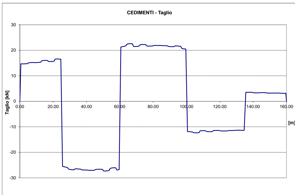
Figura 42 – Cedimento vincolare
