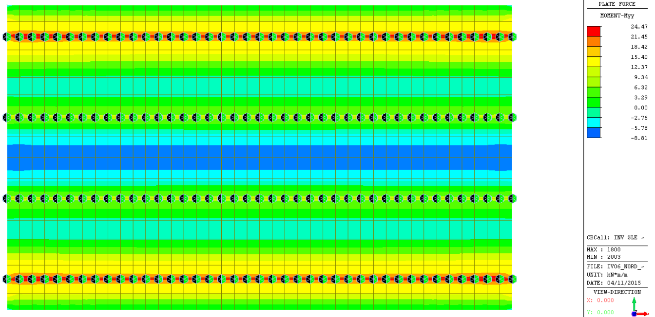
Figura 67: Sollecitazione flessionale allo SLE QUASI PERMANENTE (INVUPPO)
