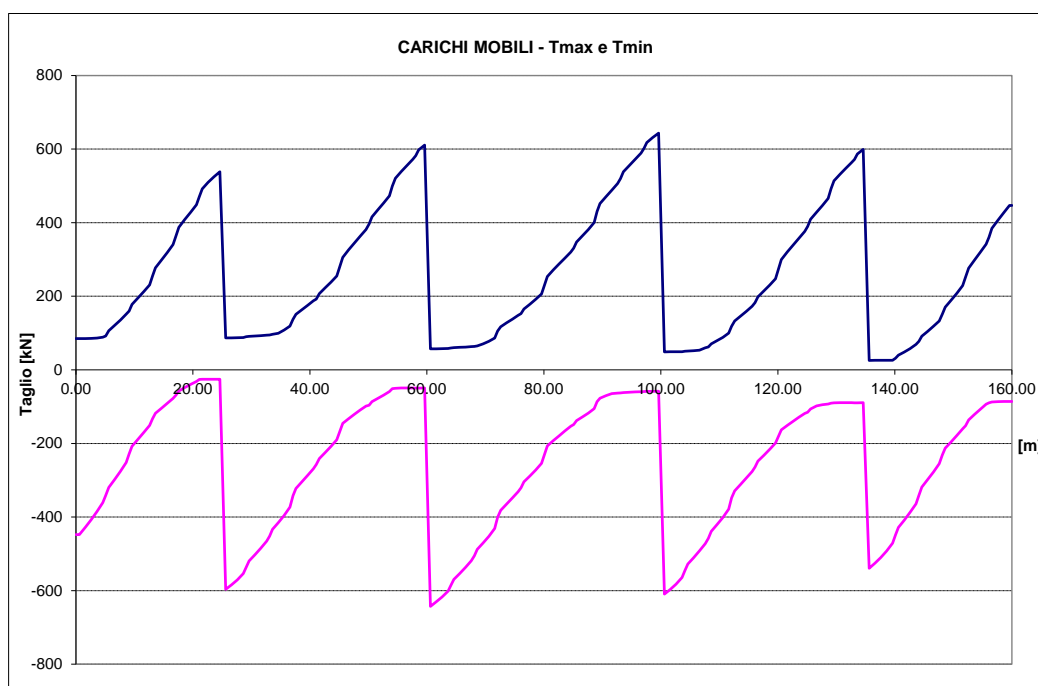
Figura 38 – Carichi accidentali (Momento e Taglio)
