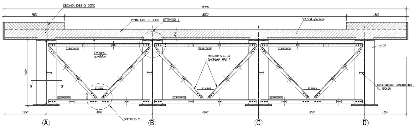
Figura 56: Sezione impalcato
