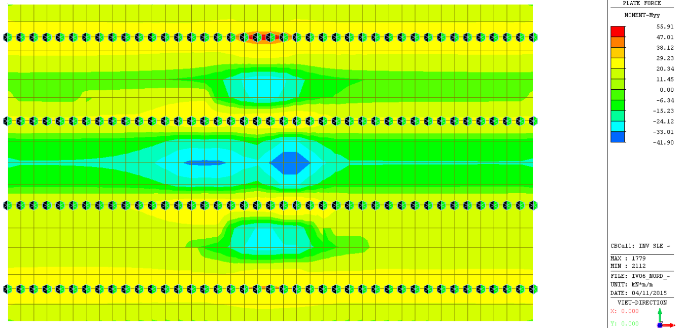
Figura 66: Sollecitazione flessionale allo SLE RARA (involuppo)
