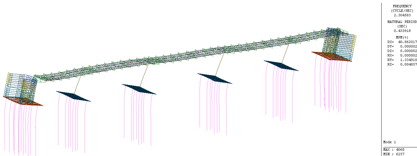
Figura 43: Modo 1: T=0.43 sec
