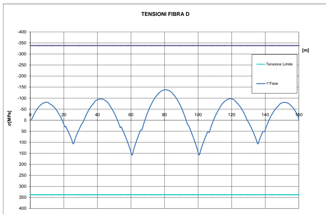
Figura 46 – Peso travi + Peso Soletta (Tensioni normali )
