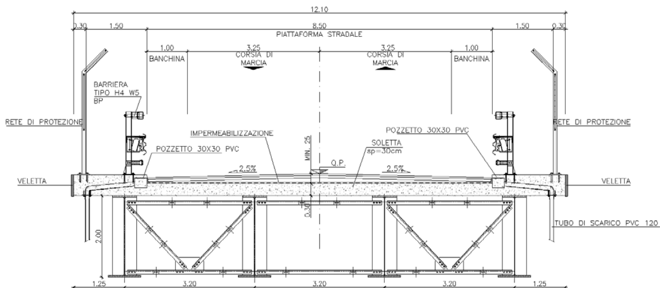
Figura 7: Sezione trasversale
