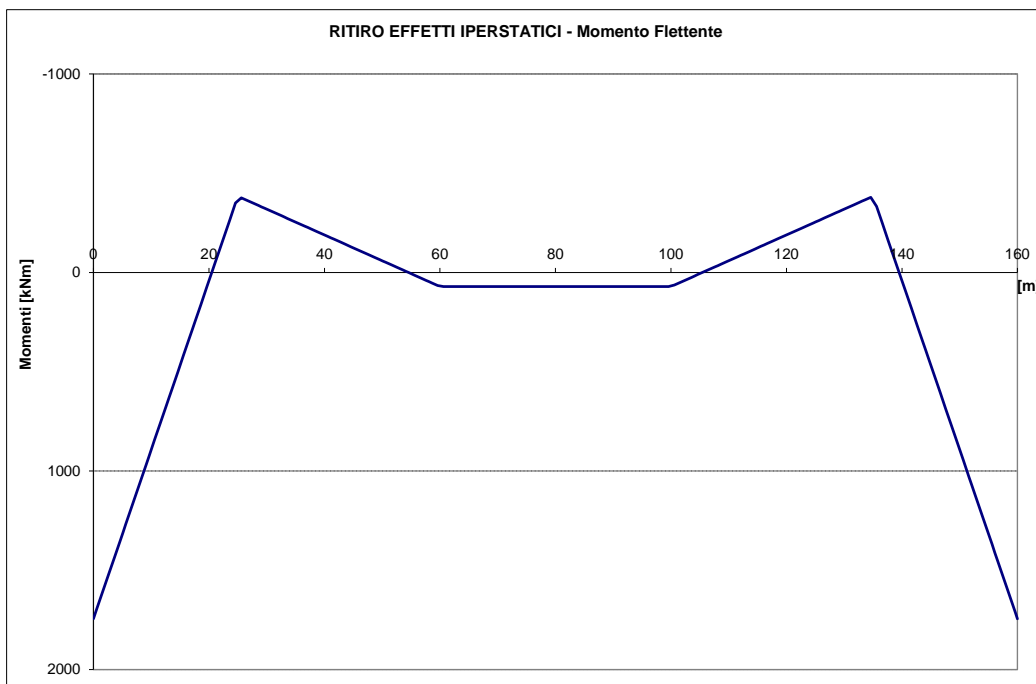
Figura 41 – Ritiro
