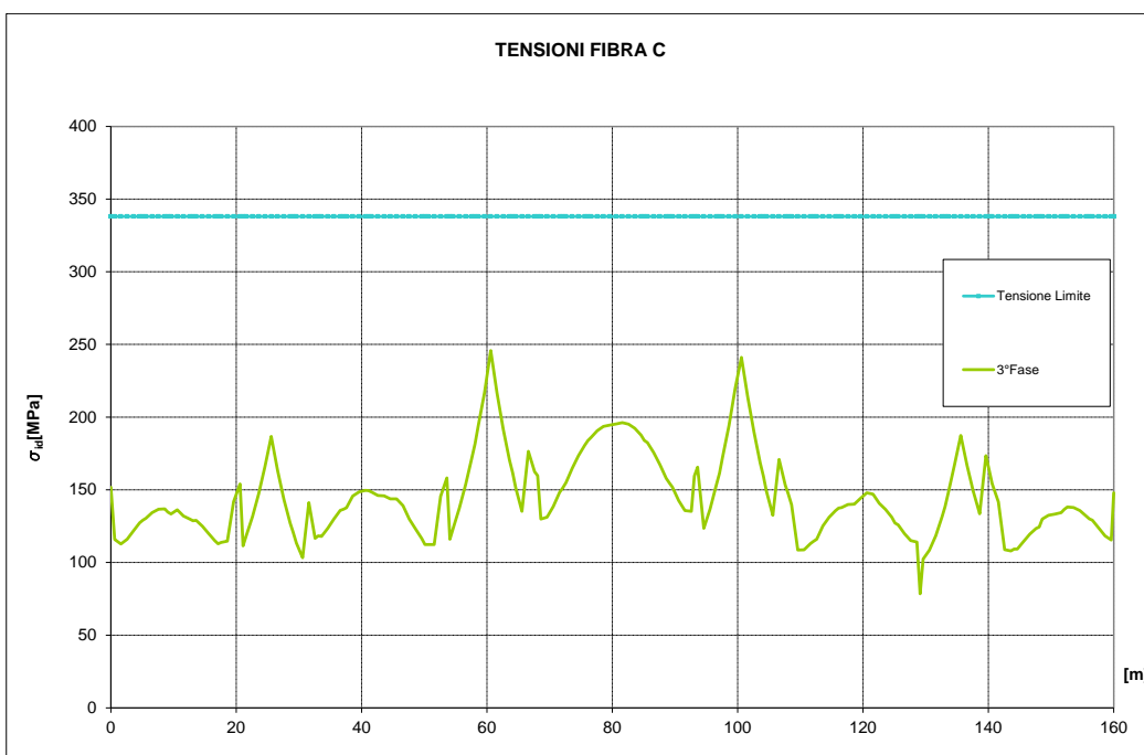
Figura 51 – Involuppo tensioni ideali
