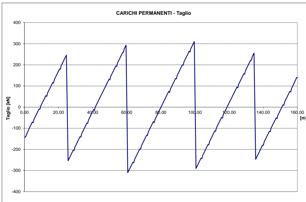
Figura 39 – Carichi permanenti
