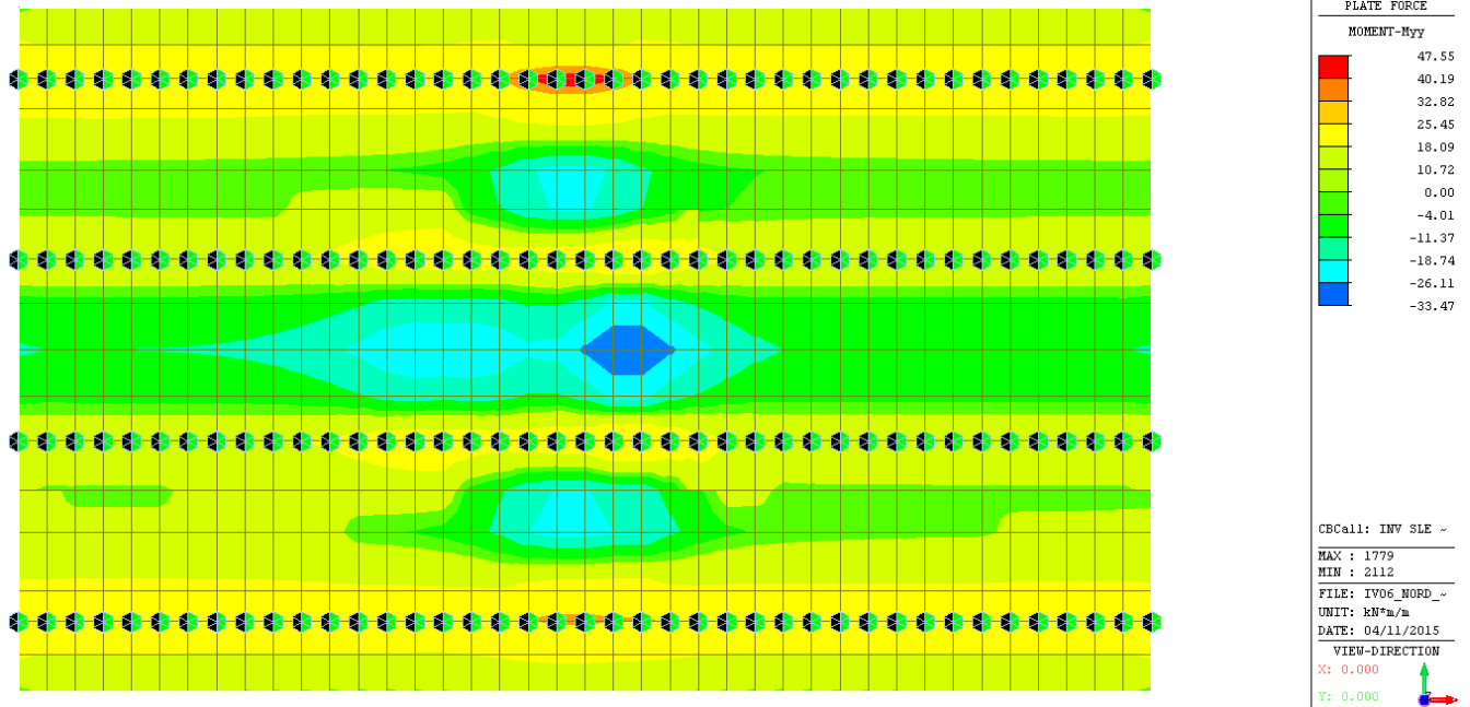
Figura 68: Sollecitazione flessionale allo SLE frequente (INVUPPO)
