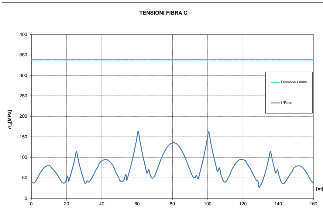
Figura 47 – Peso travi + Peso Soletta (Tensioni ideali)
