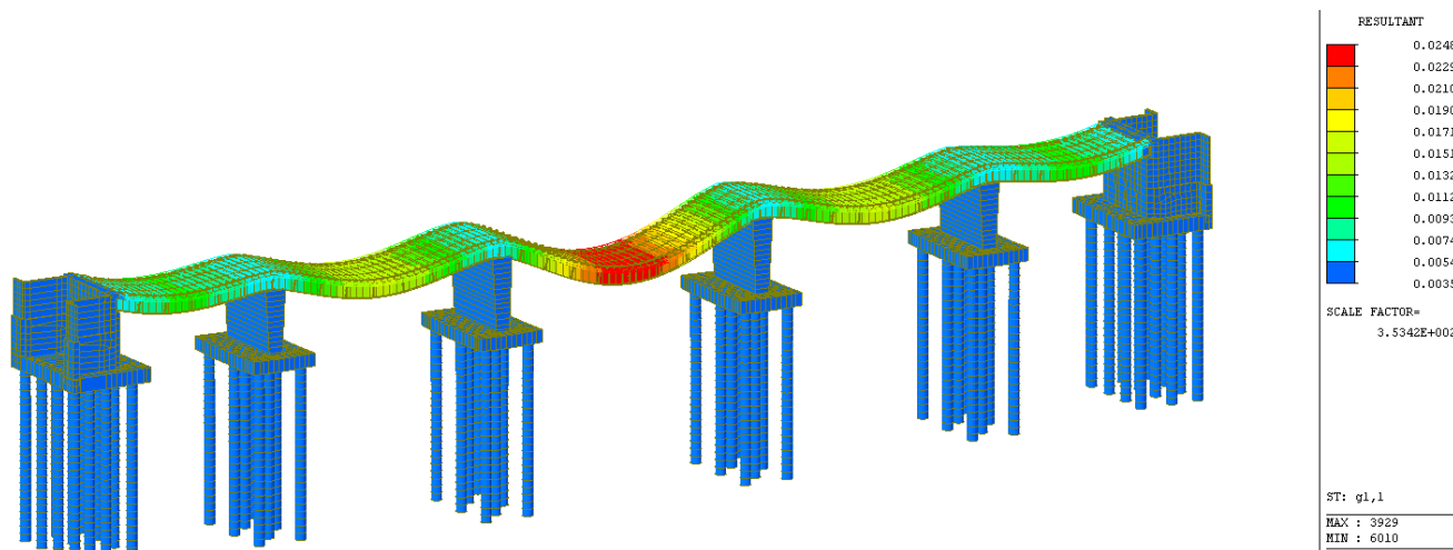
Figura 55: Peso proprio – Abbassamenti
