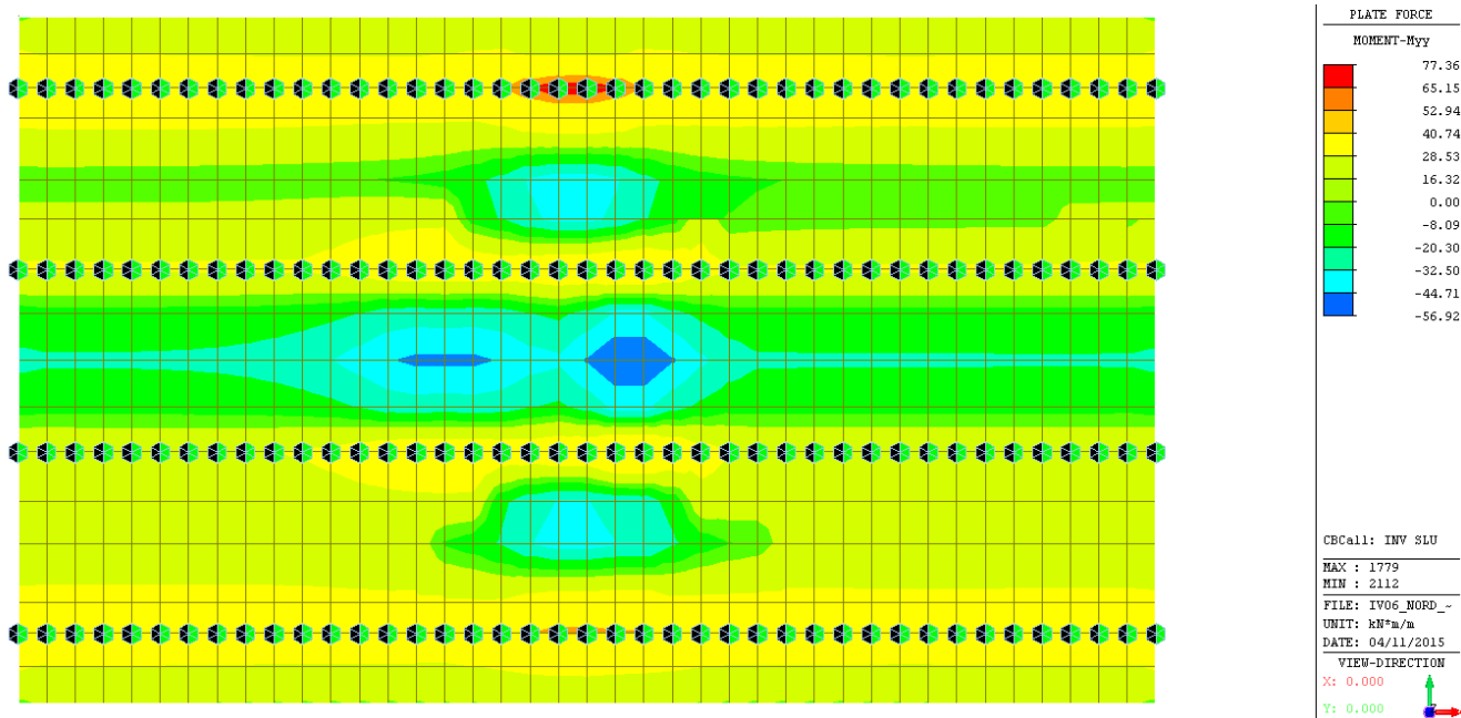
Figura 65: Sollecitazione flessionale allo SLU (involuppo)
