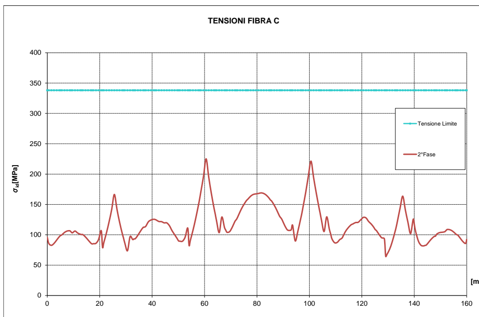
Figura 49 – Involuppo tensioni ideali
