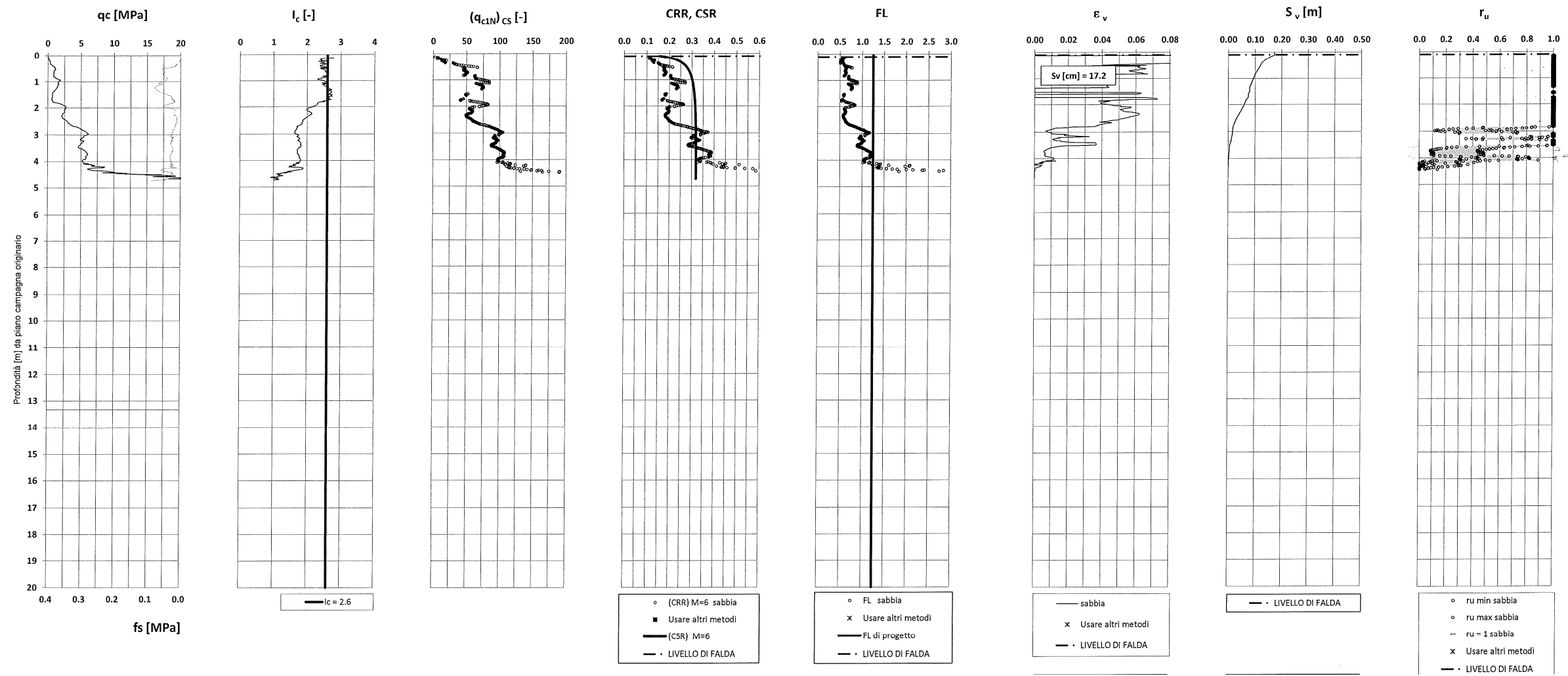
Figura 15: Analisi di liquefazione CPTU31 senza rilevato
