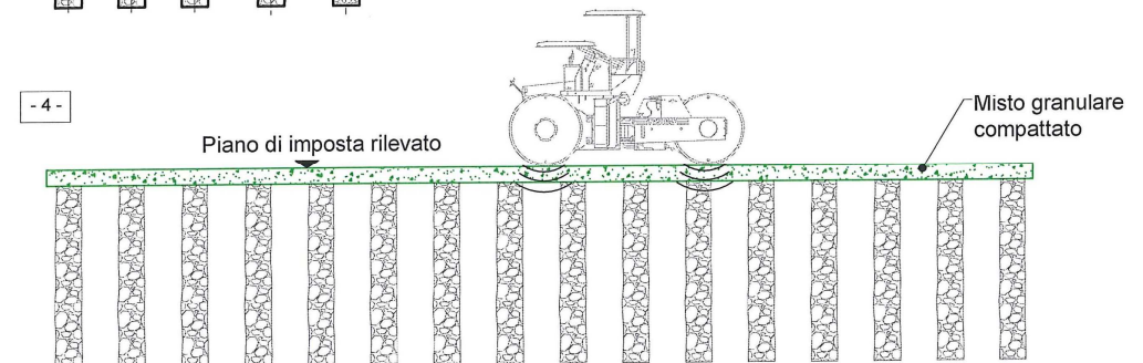
Figura 13: Fasi realizzative colonne in ghiaia
