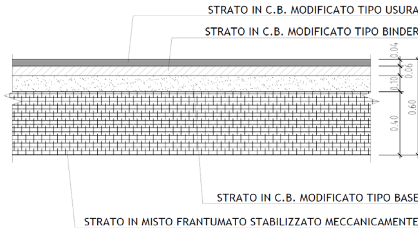
Figura 9: Particolare pavimentazione strada categoria C1
