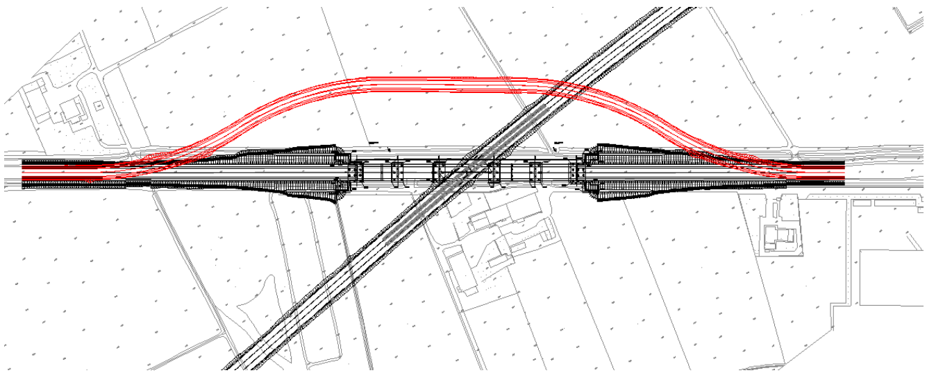
Figura 12: Deviazione provvisoria
