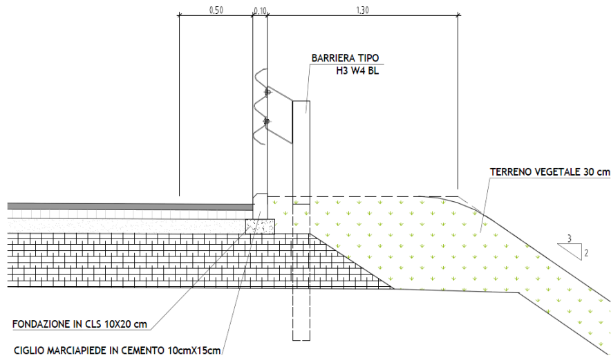
Figura 8:Particolare arginello
