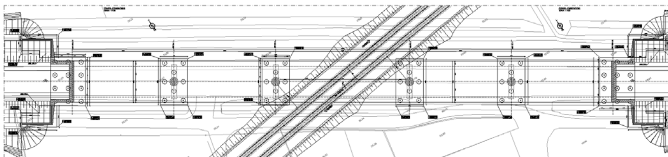
Figura 2: Pianta fondazioni
