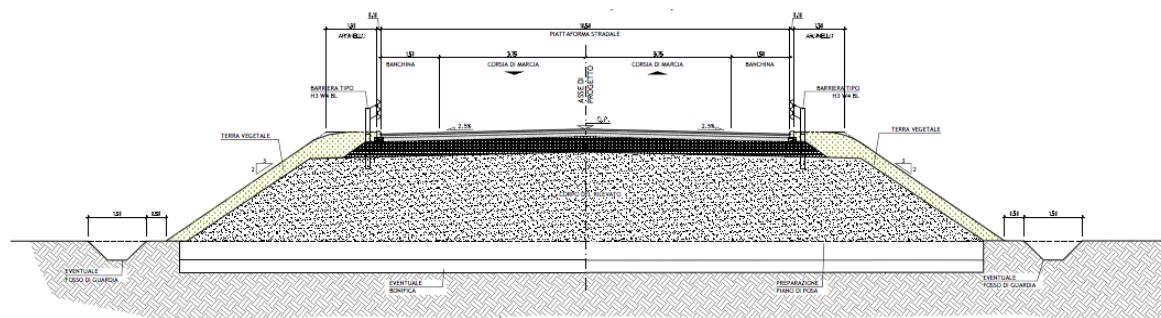
Figura 7: Sezione tipo strada C1
