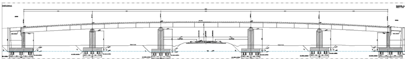
Figura 3: Profilo longitudinale
