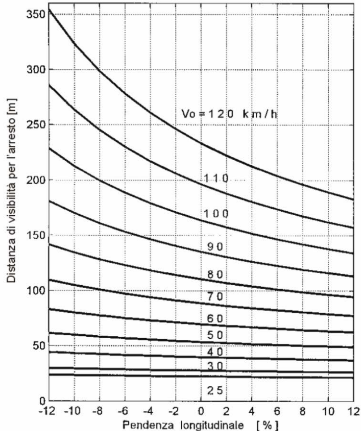
Figura 6: Abaco distanza visibilità
