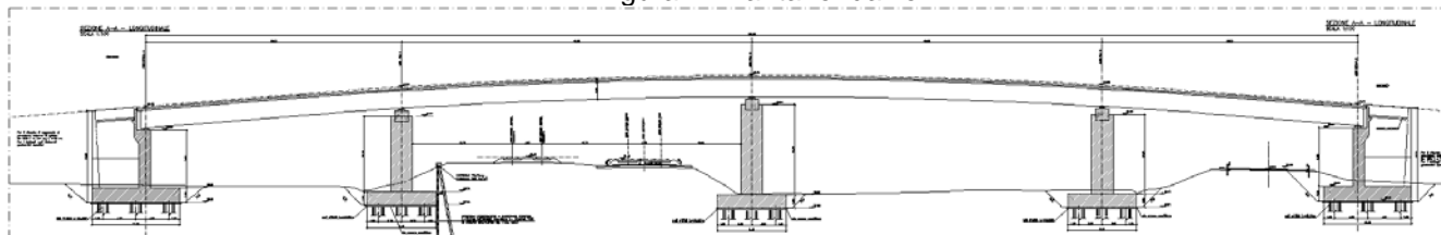
Figura 3: Profilo longitudinale
