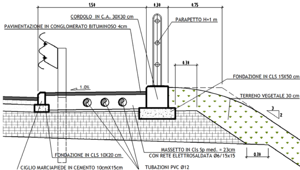
Figura 11: Particolare arginello
