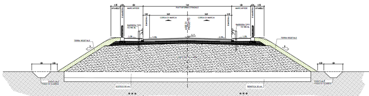
Figura 10: Sezione tipo strada E
