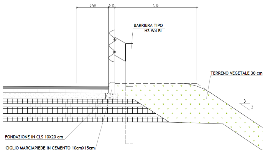
Figura 13: Particolare arginello
