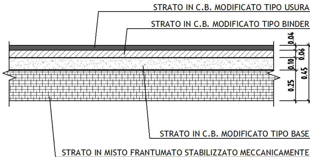
Figura 14: Particolare pavimentazione strada categoria E ed F2
