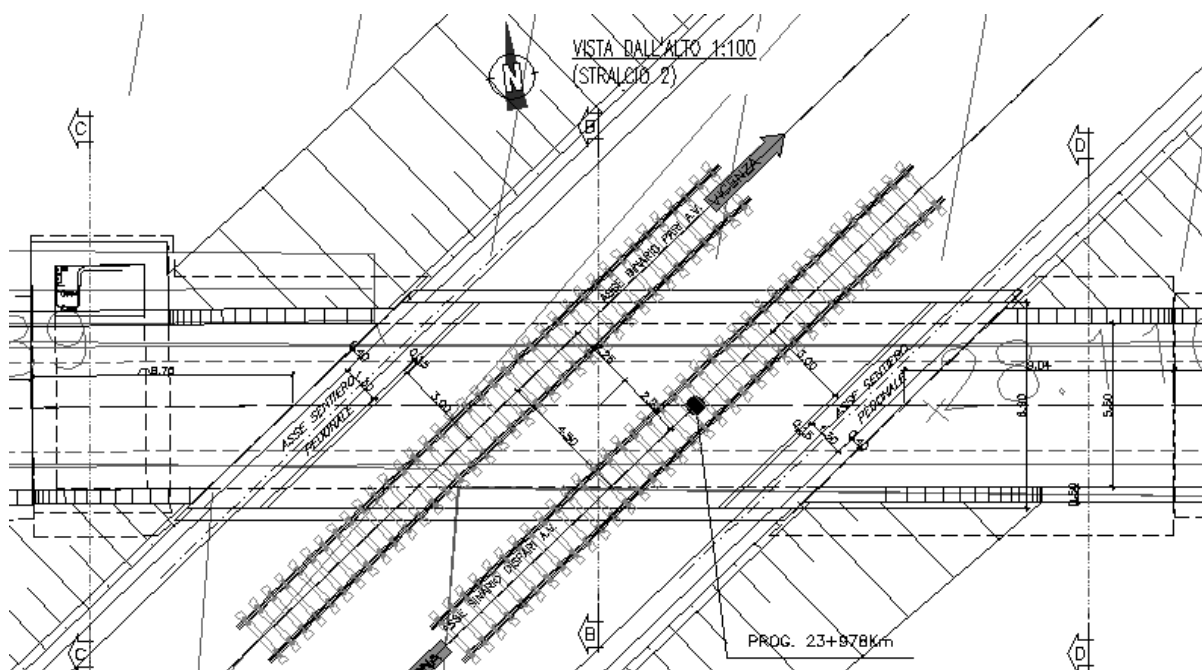
Figura 1 – Vista dall'alto
