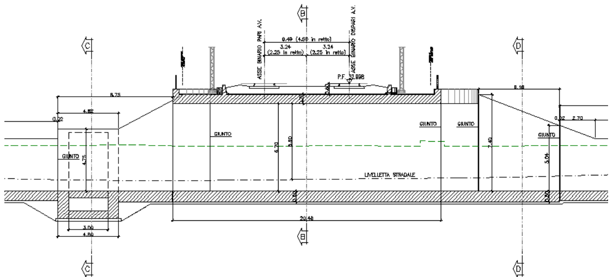
Figura 2 - Sezione longitudinale
