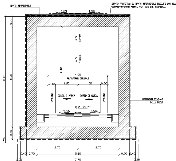
Figura 3 - Sezione trasversale
