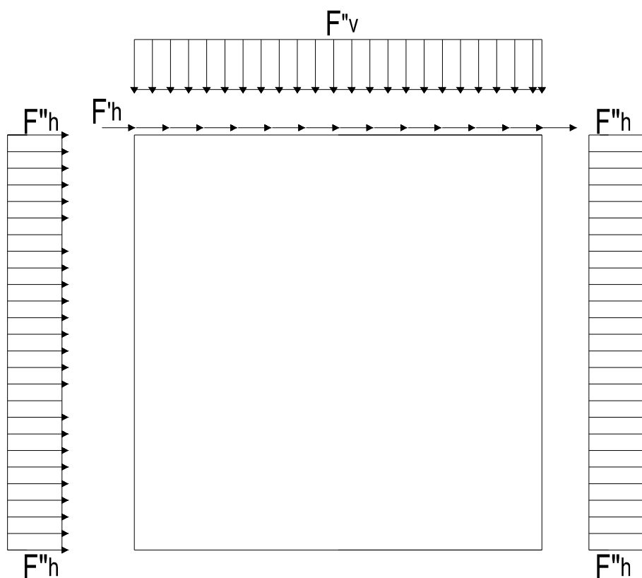
Figura 4 - Forze sismiche agenti sulla struttura
