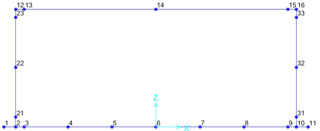
Figura 6 - Modello F.E.M struttura - numerazione nodi
