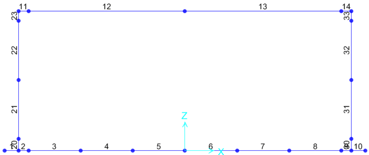
Figura 7 - Modello F.E.M. struttura – numerazione aste
