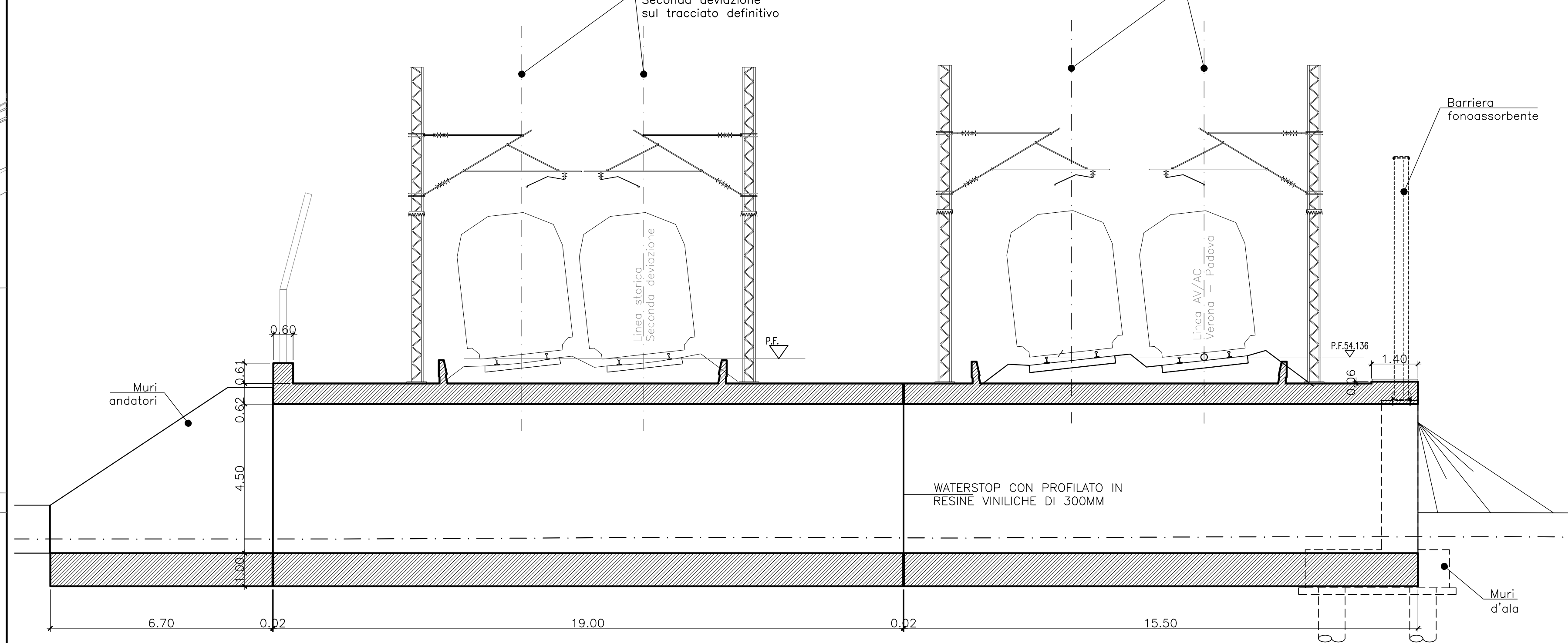
SEZIONE FASE 3 1:100
