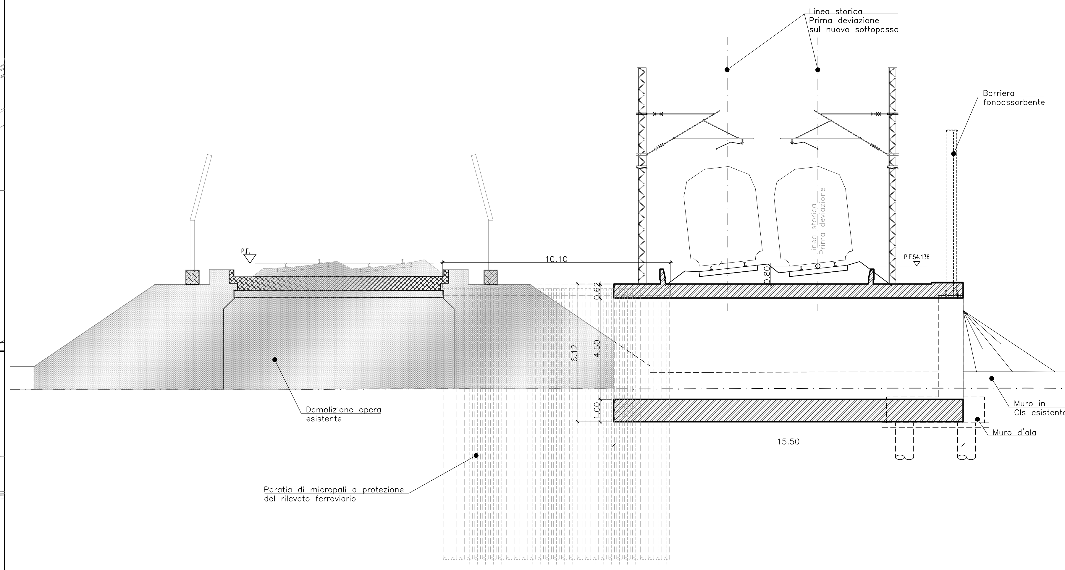
SEZIONE FASE 2 1:100
