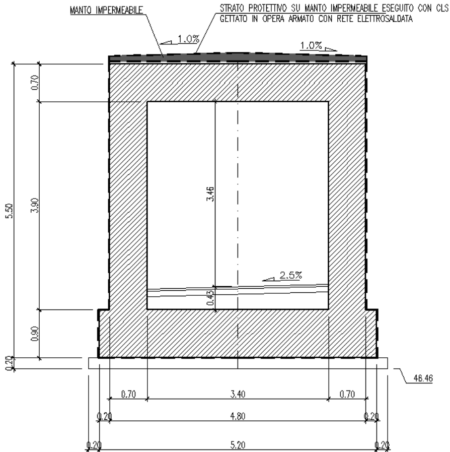
Figura 3 - Sezione trasversale
