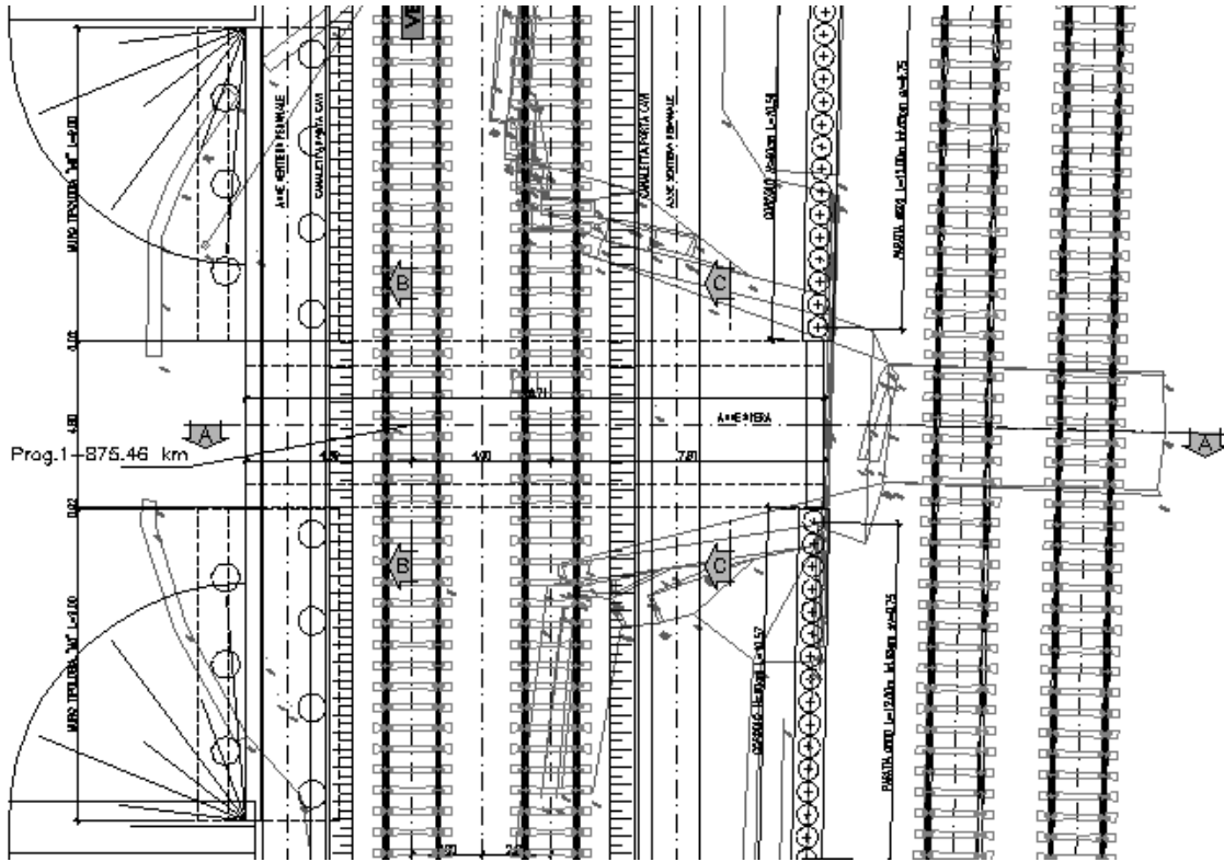
Figura 1 – Vista dall'alto
