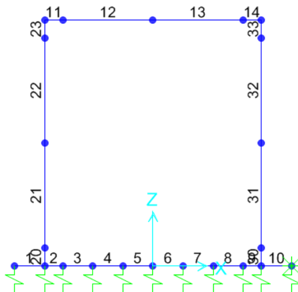
Figura 10 - Modello F.E.M. struttura – numerazione aste
