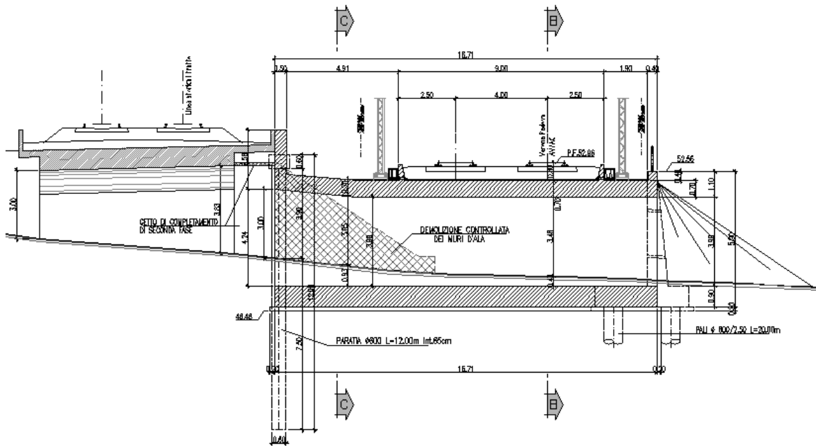
Figura 2 - Sezione longitudinale
