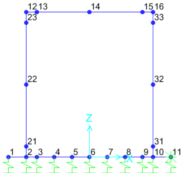
Figura 9 - Modello F.E.M struttura - numerazione nodi
