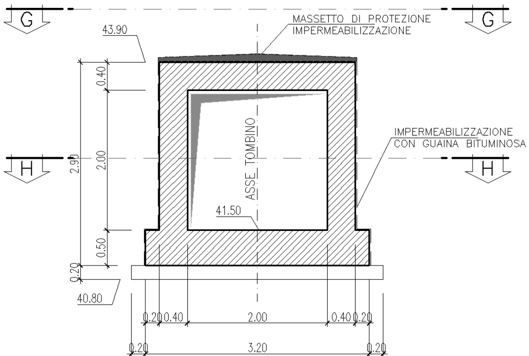
Figura 3 - Sezione trasversale
