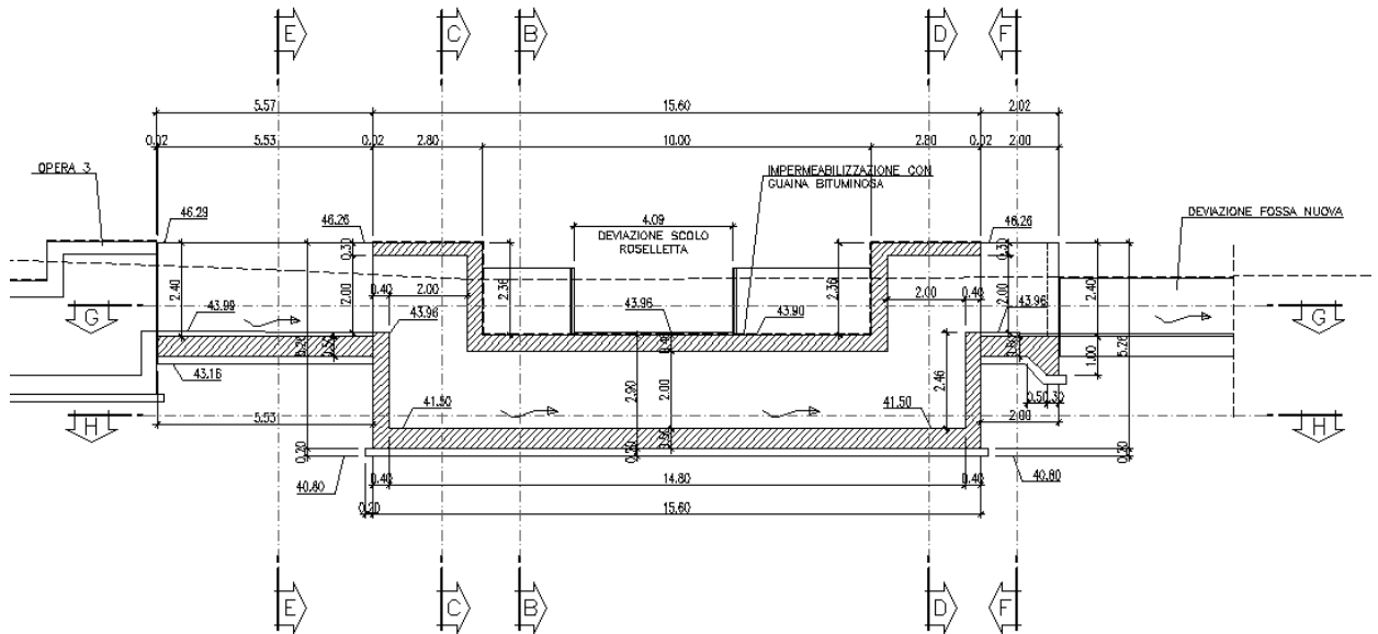
Figura 2 - Sezione longitudinale
