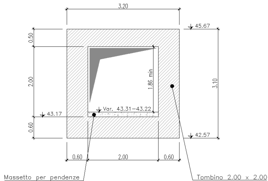
Figura 3 - Sezione trasversale
