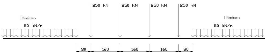
Figura 4 - Treno LM71
