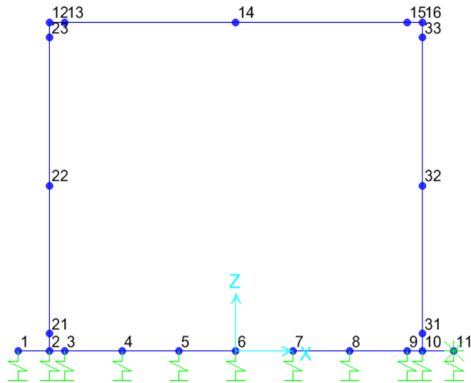
Figura 6 - Modello F.E.M struttura - numerazione nodi
