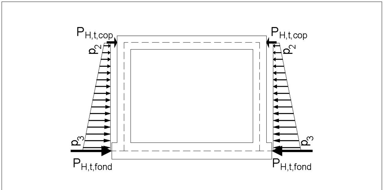
Figura 3 - Spinte del terreno
