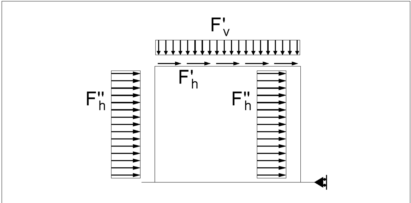
Figura 5 - Forze sismiche agenti sulla struttura
