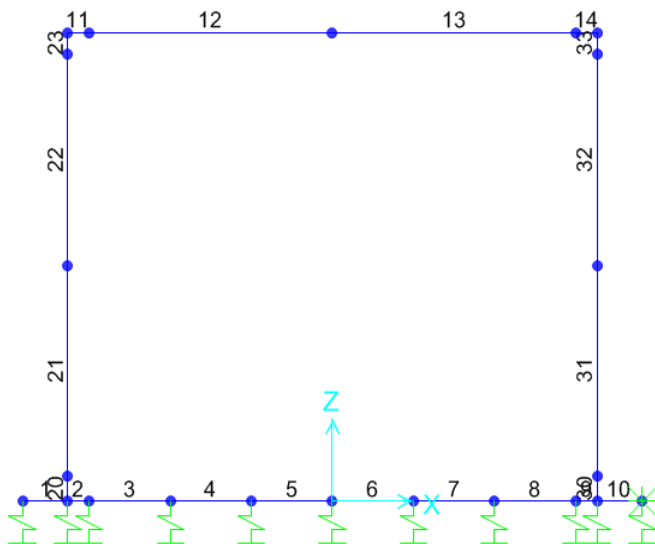
Figura 7 - Modello F.E.M. struttura – numerazione aste
