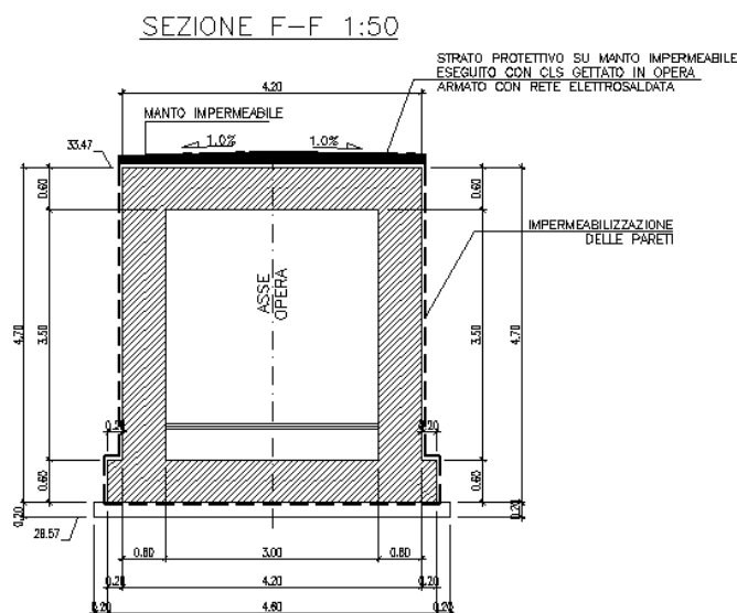
Figura 1 - Sezione trasversale
