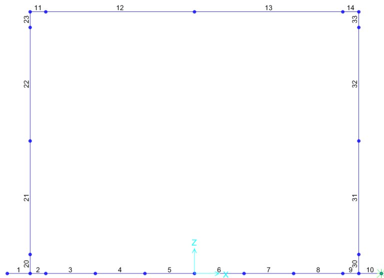
Figura 9 - Modello F.E.M. struttura – numerazione aste
