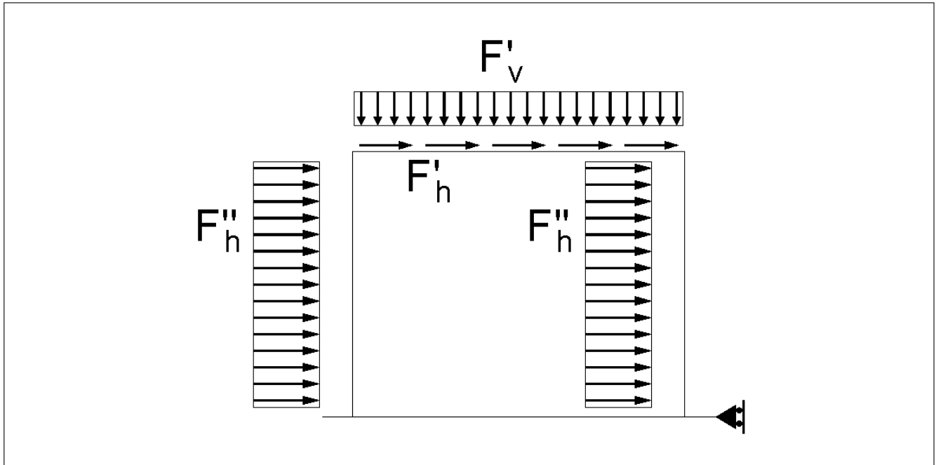
Figura 7 - Forze sismiche agenti sulla struttura
