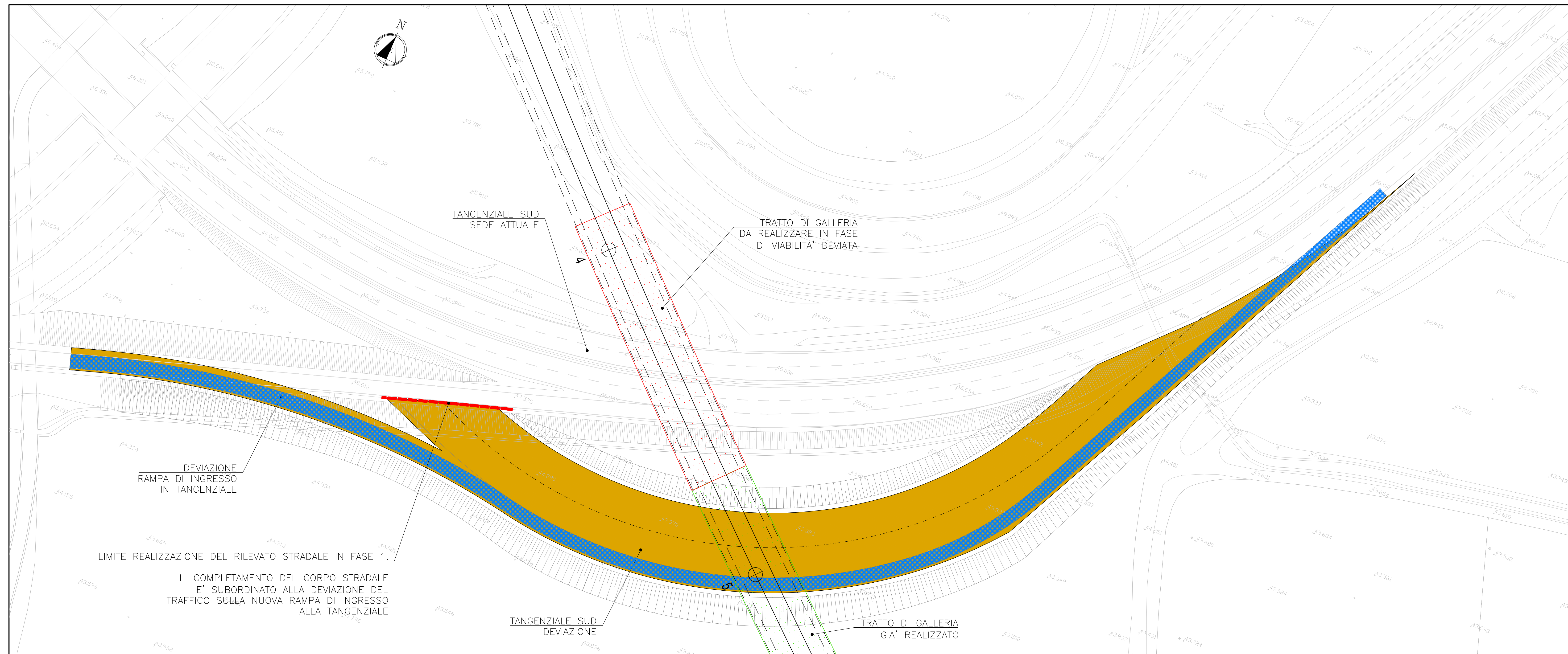
DEVIAZIONE TANGENZIALE SUD – FASE 1 PLANIMETRIA 1:500
