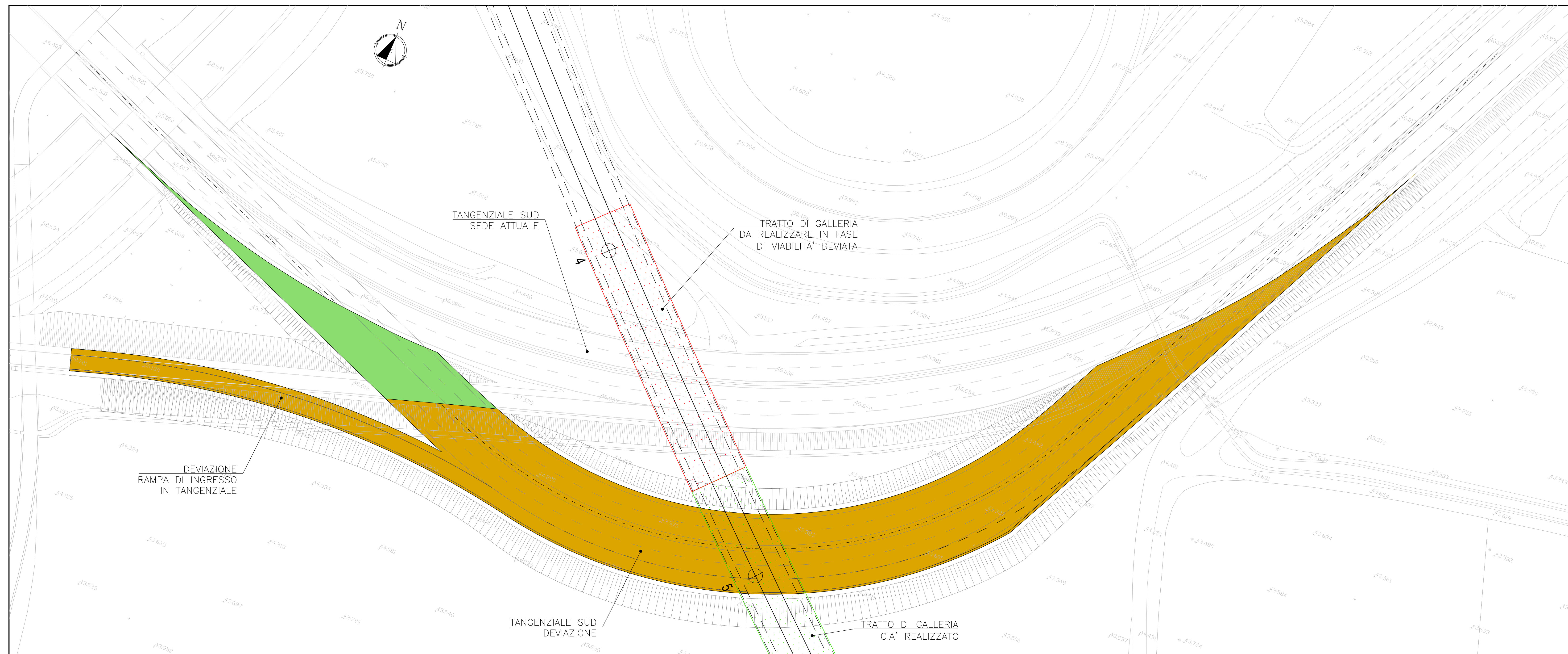
DEVIAZIONE TANGENZIALE SUD – FASE 2 PLANIMETRIA 1:500
