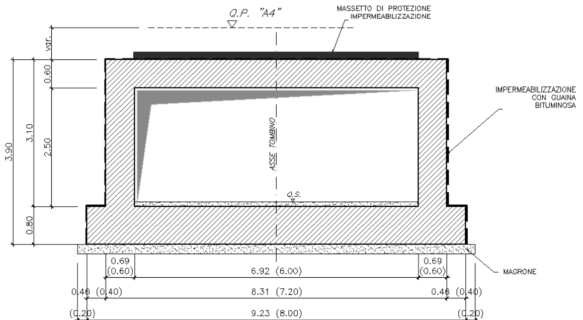
Figura 3 - Sezione trasversale
