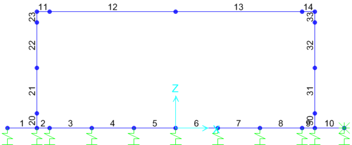
Figura 8 - Modello F.E.M. struttura – numerazione aste
