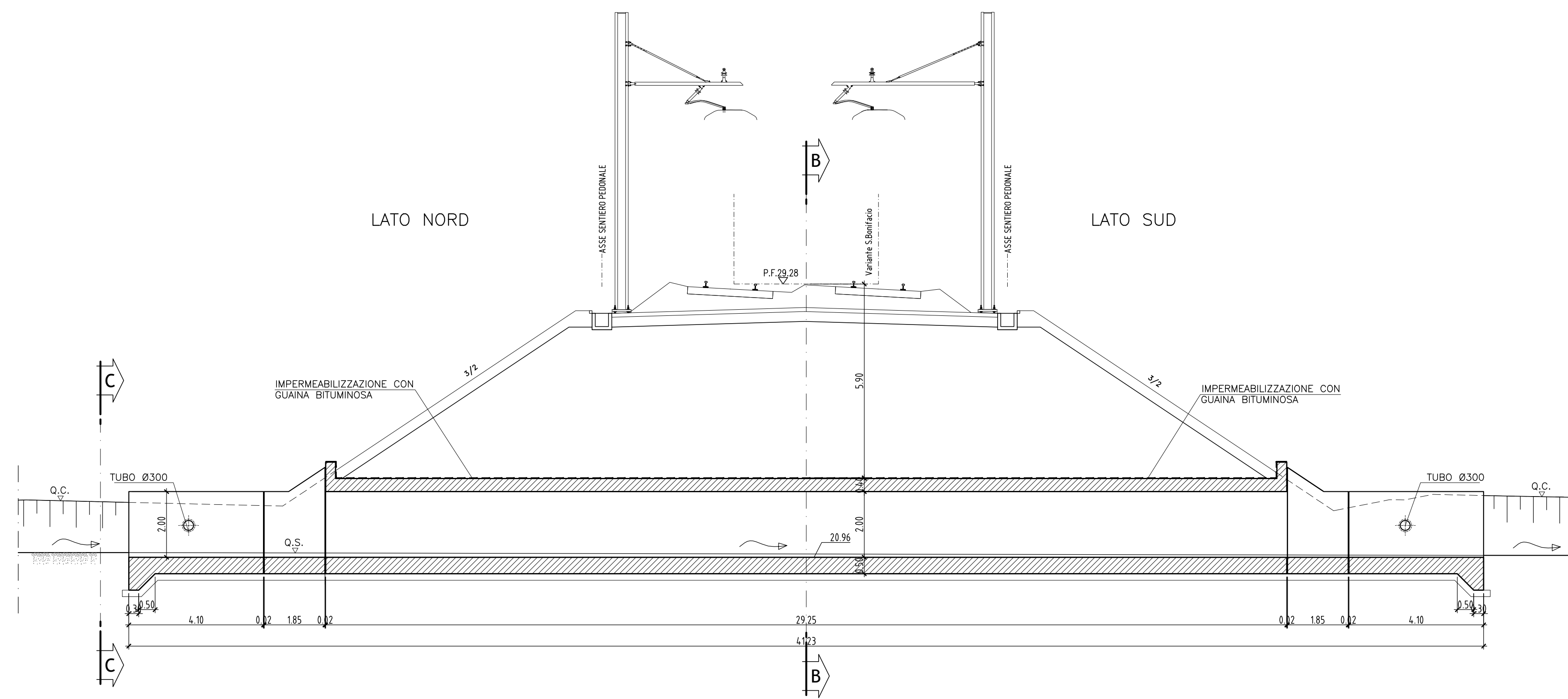
SEZIONE LONGITUDINALE A-A 1:100
