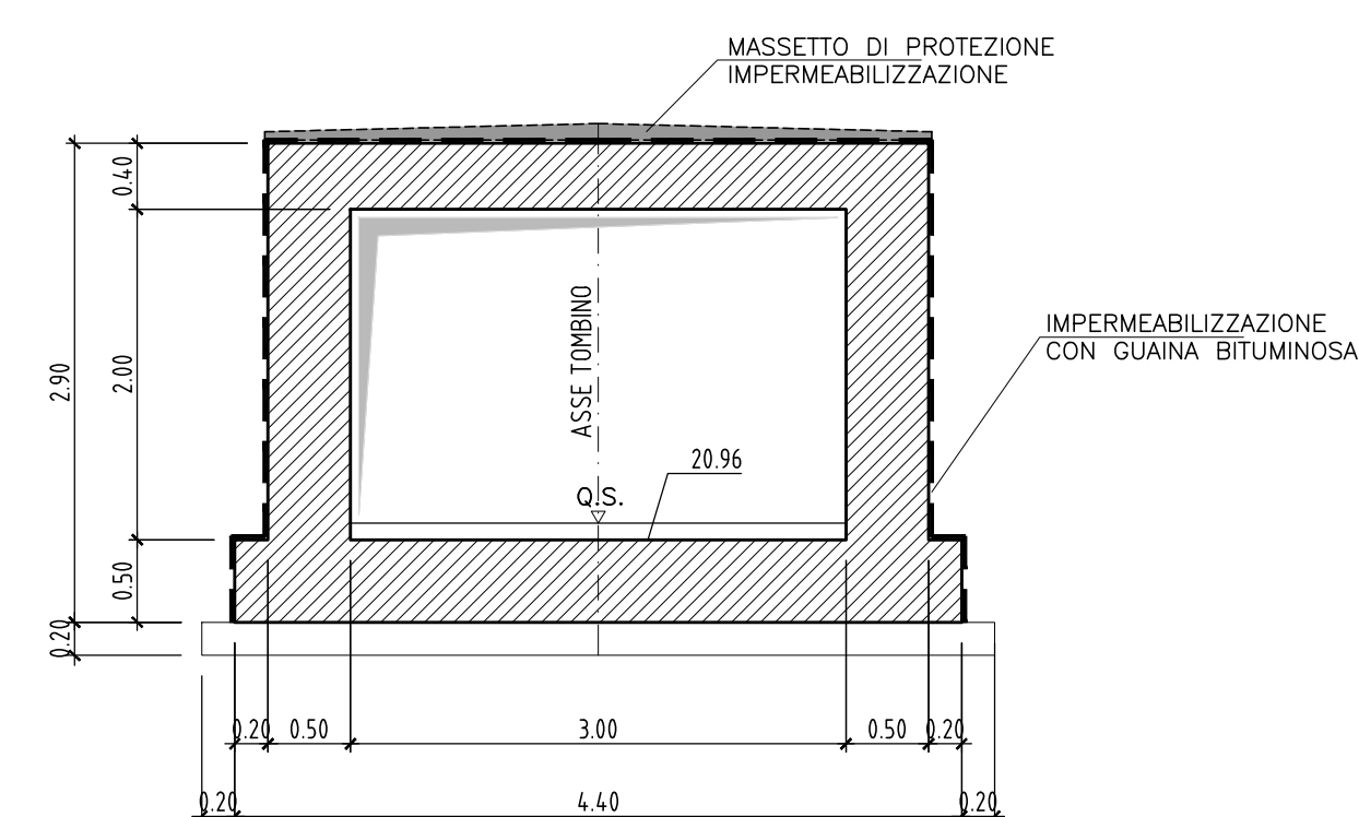
SEZIONE B-B 1:50
