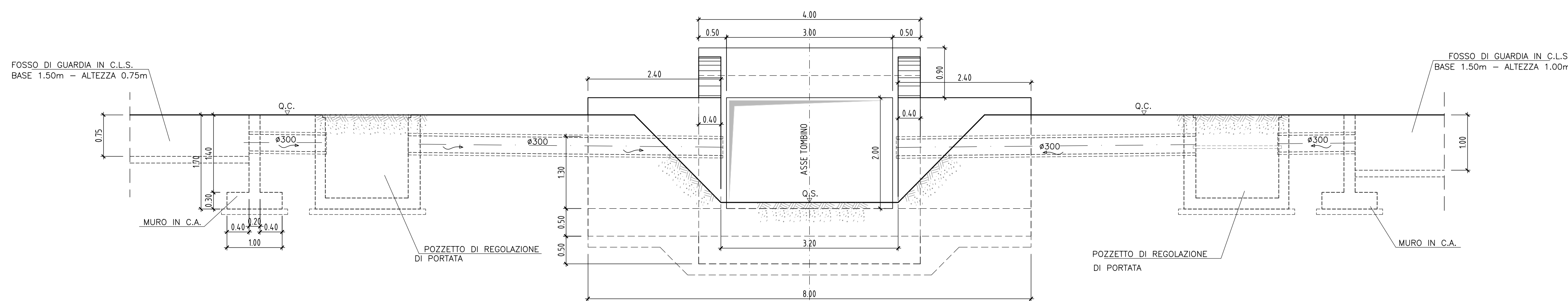
VISTA C-C 1:50
