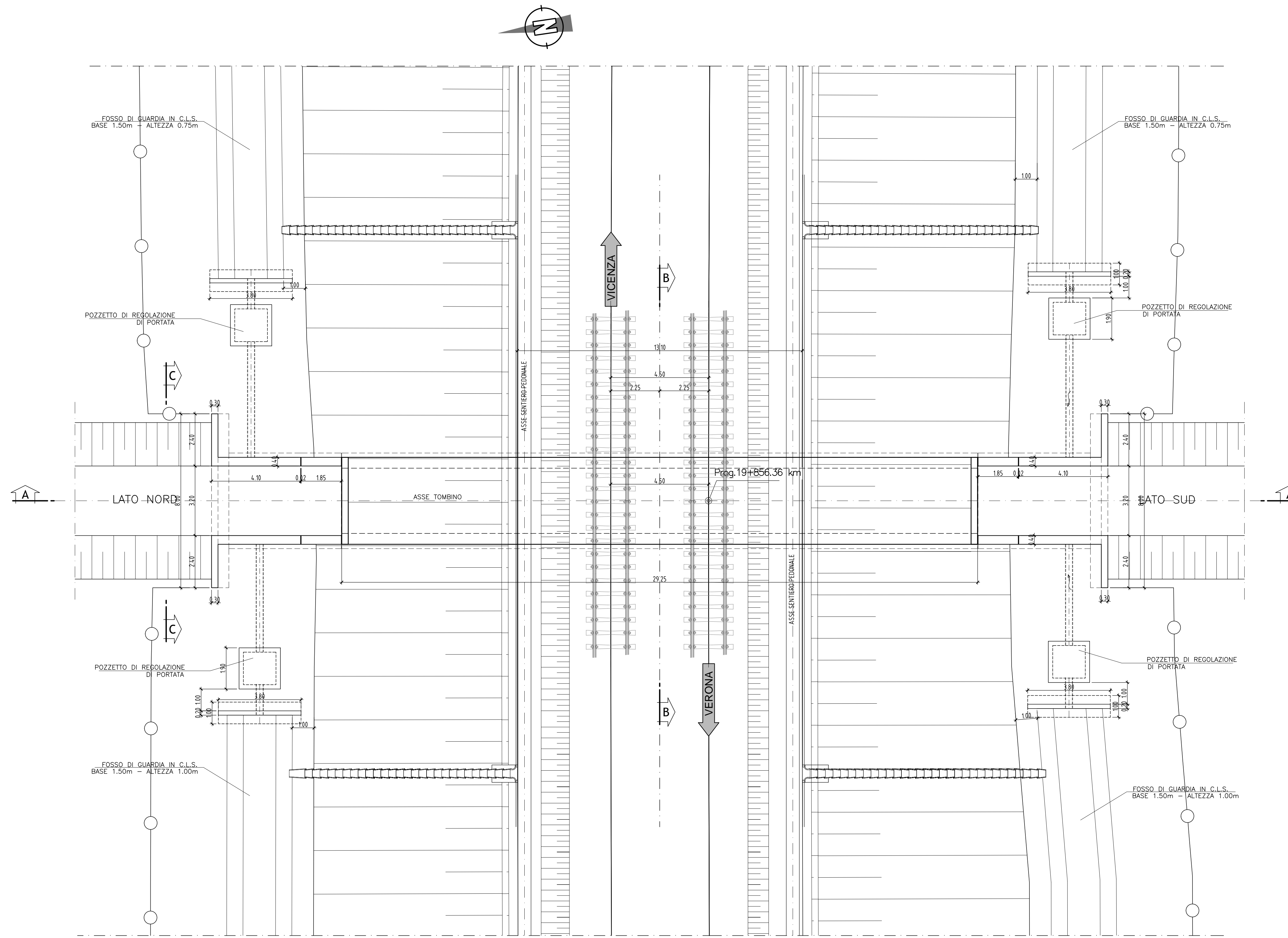
VISTA DALL'ALTO 1:100
