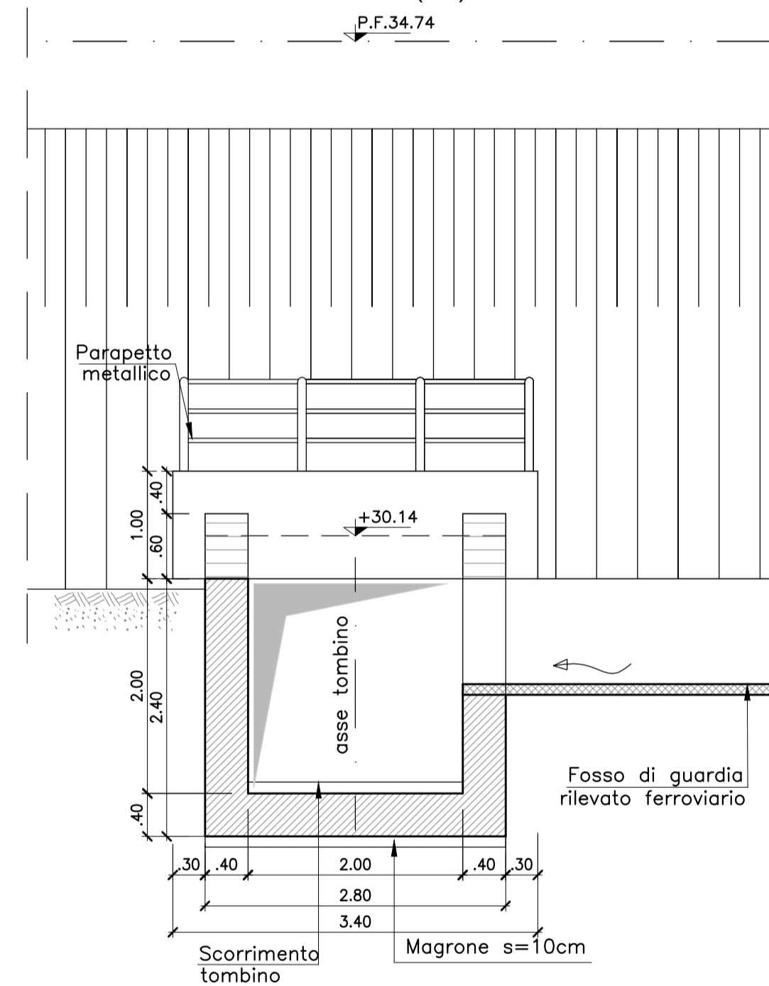
SEZIONE B-B (1:50)
