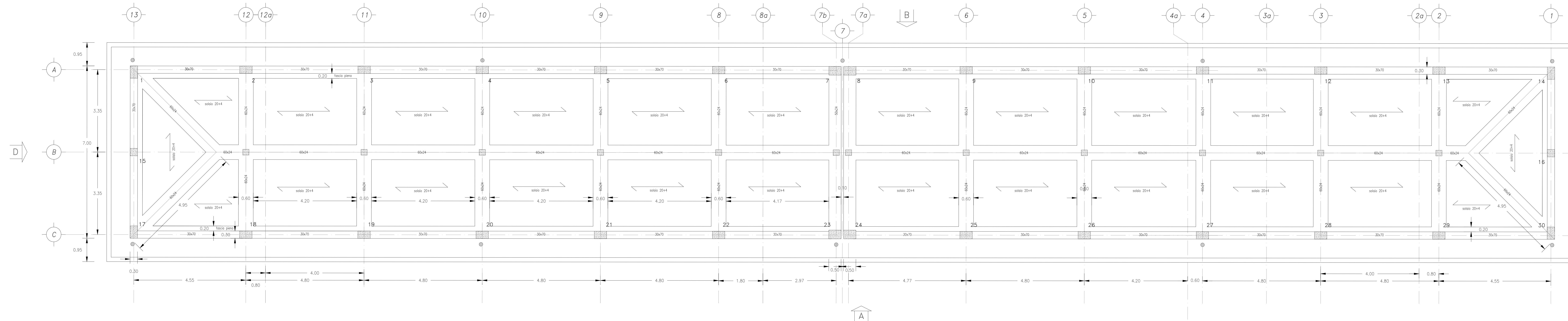
PIANTA COPERTURA a quota +5.69 Scala 1:50
