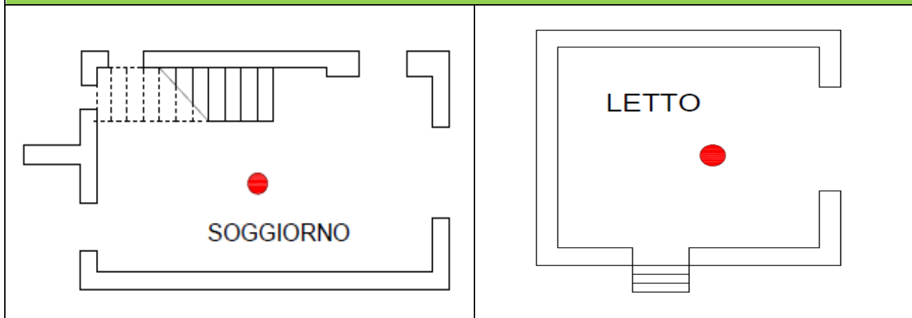
Posizionamento accelerometro triassiale, 1° piano f.t.
