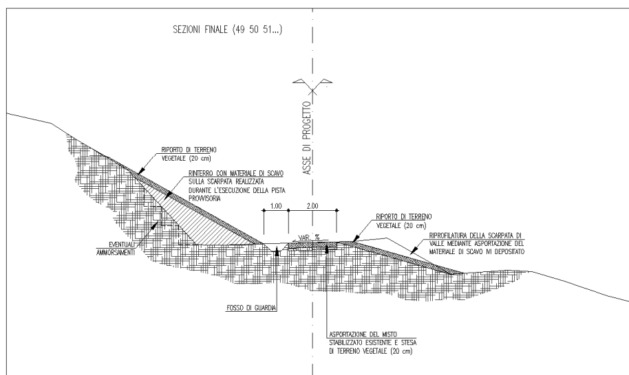
Figura 7 – Sezioni tipo
