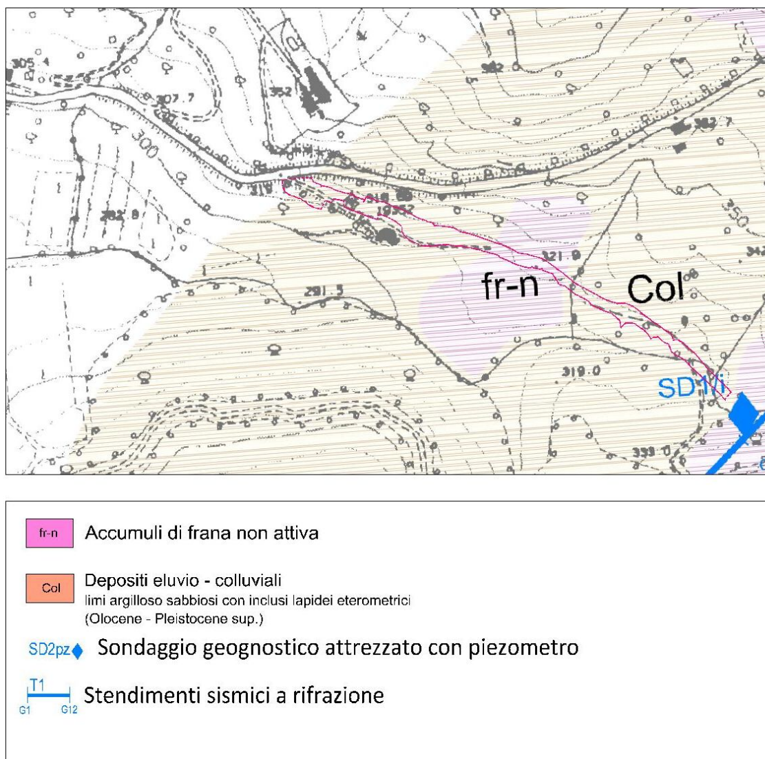
Figura 4 – Stralcio della Carta geologica della strada di cantiere.
