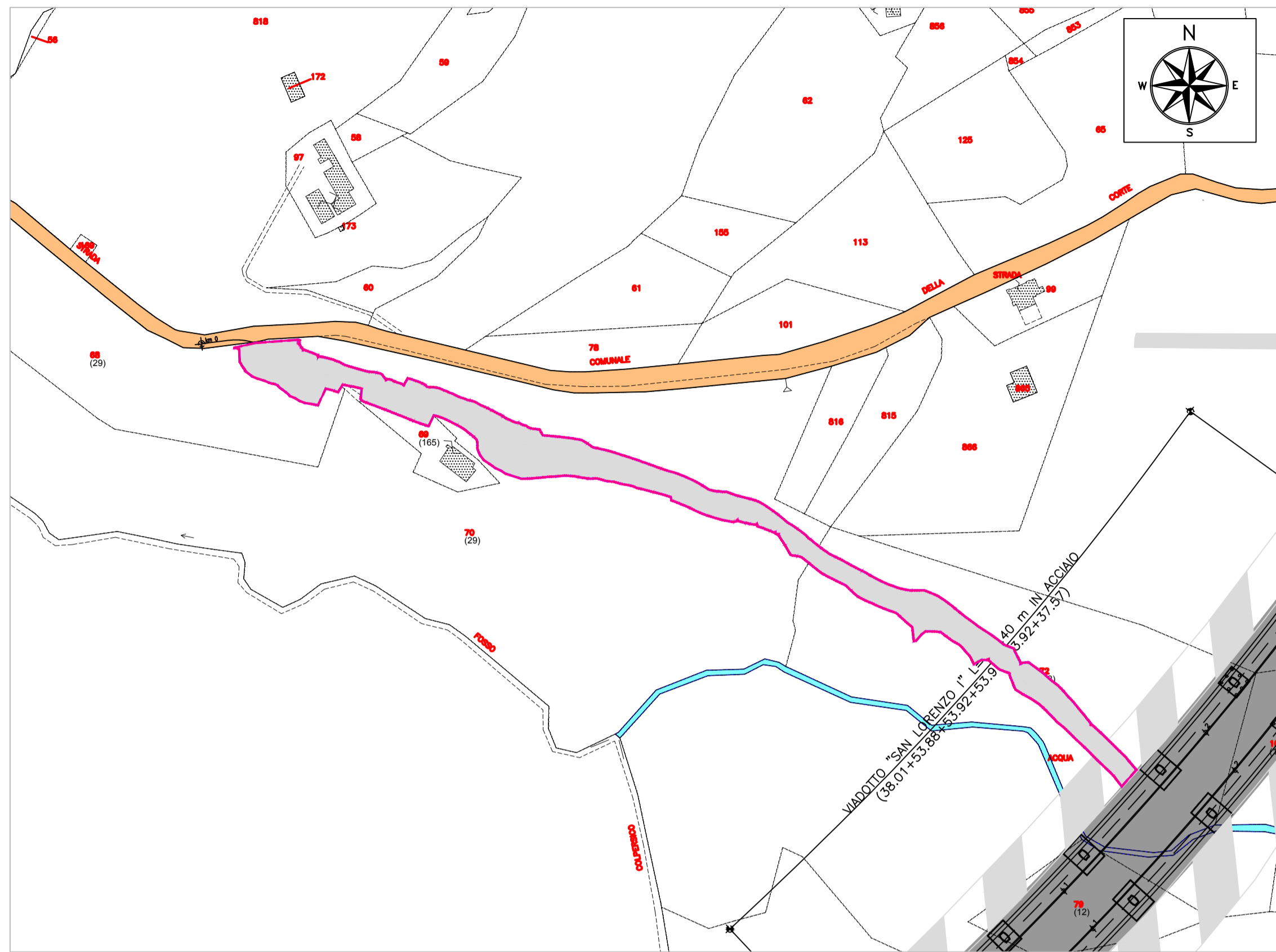
STRALCIO PLANIMETRIA CATASTALE – SCALA 1:2000
