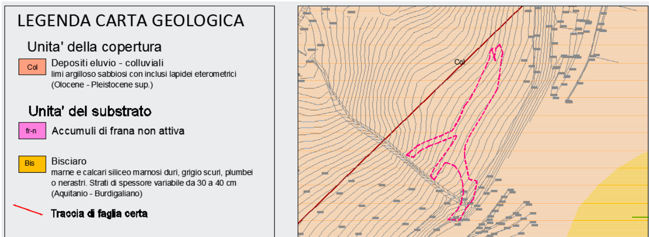
Figura 5 – Stralcio della Carta geologica della strada di cantiere.
