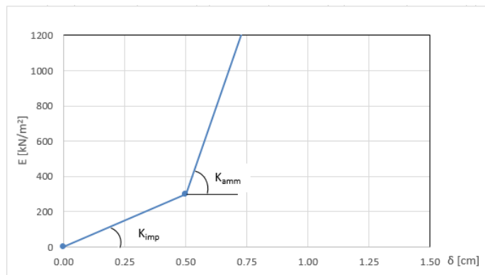
Figura 3: Schematizzazione dell'interfaccia
