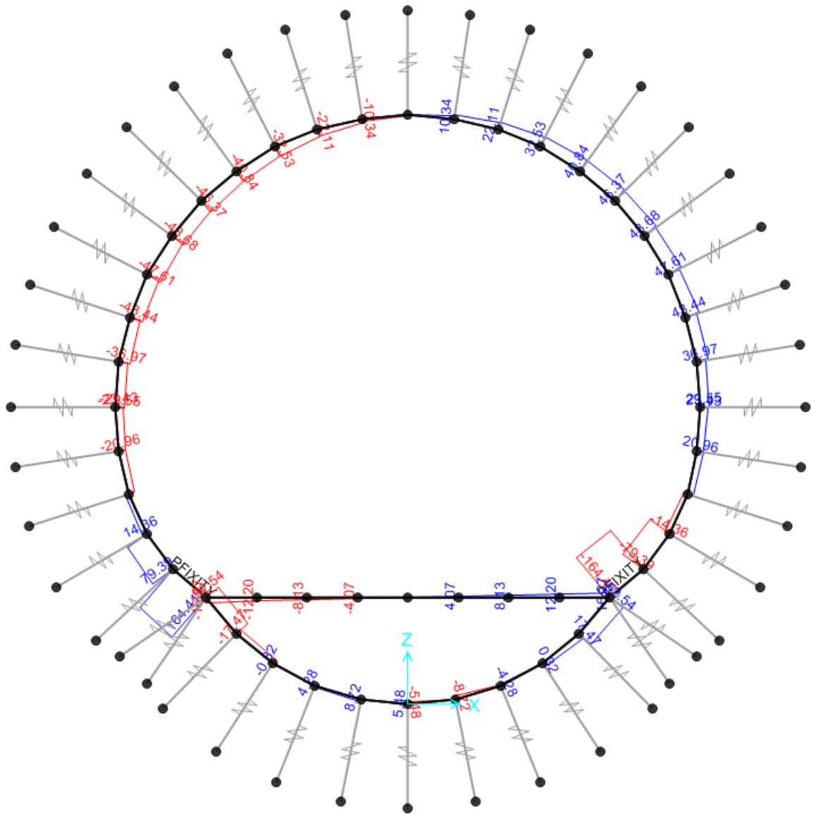
Abbildung 6: GZT06 - Schub
