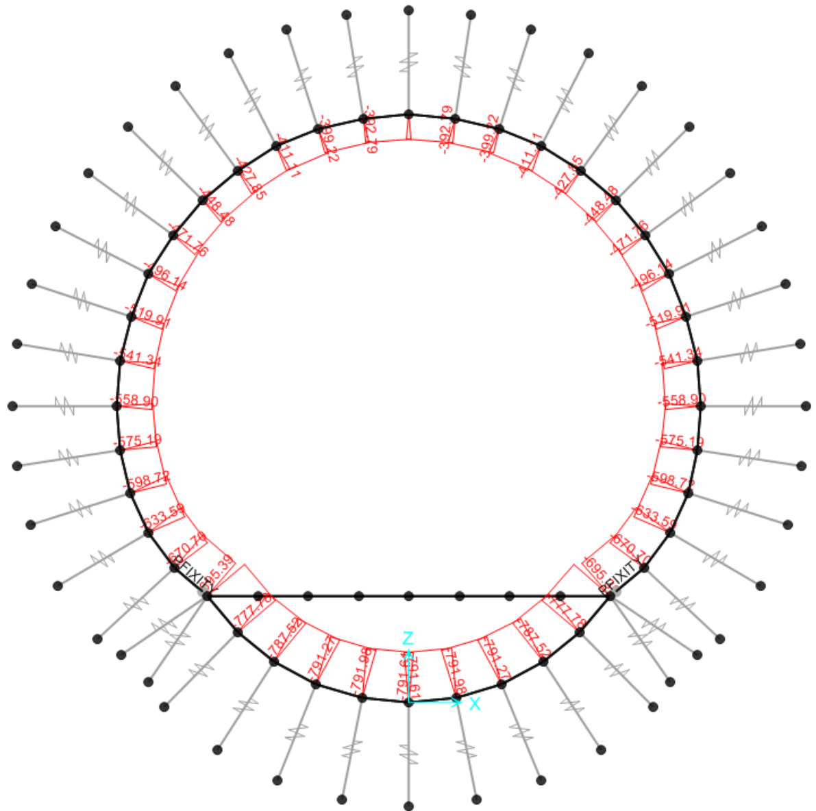
Abbildung 5: GZT06 - Axialwirkung
