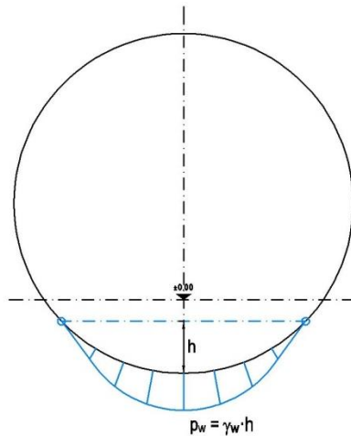
Abbildung 4: Hydrostatischer Druck – drainierter Regelquerschnitt
