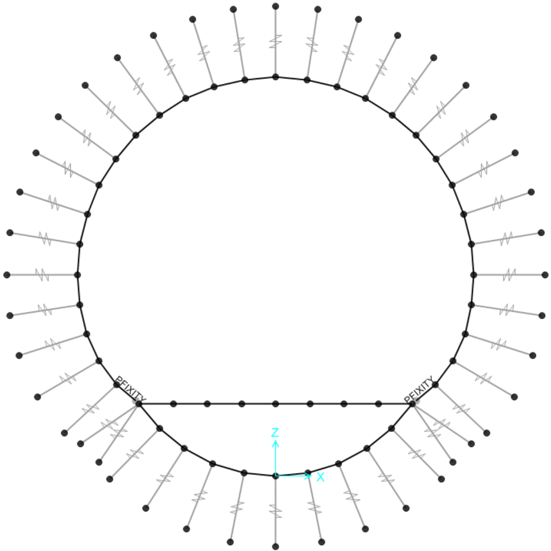
Abbildung 2: Geometrisches Modell des Ausbruchquerschnitts C-E-Ta
