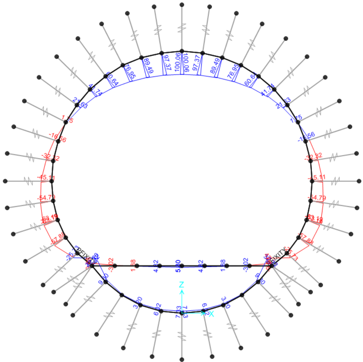
Abbildung 4: GZT06 - Biegunsmoment
