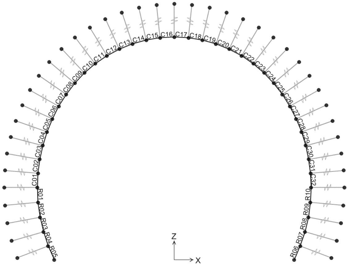
Abbildung 1: Modell CL-E-T
