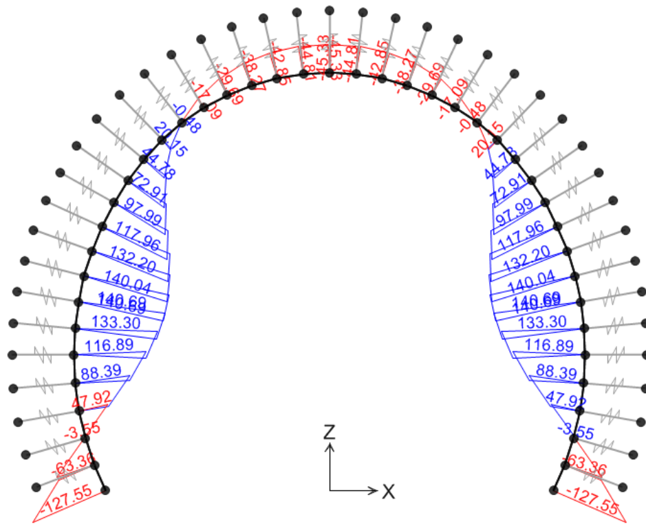
Abbildung 4: GZT06 - Biegunsmoment
