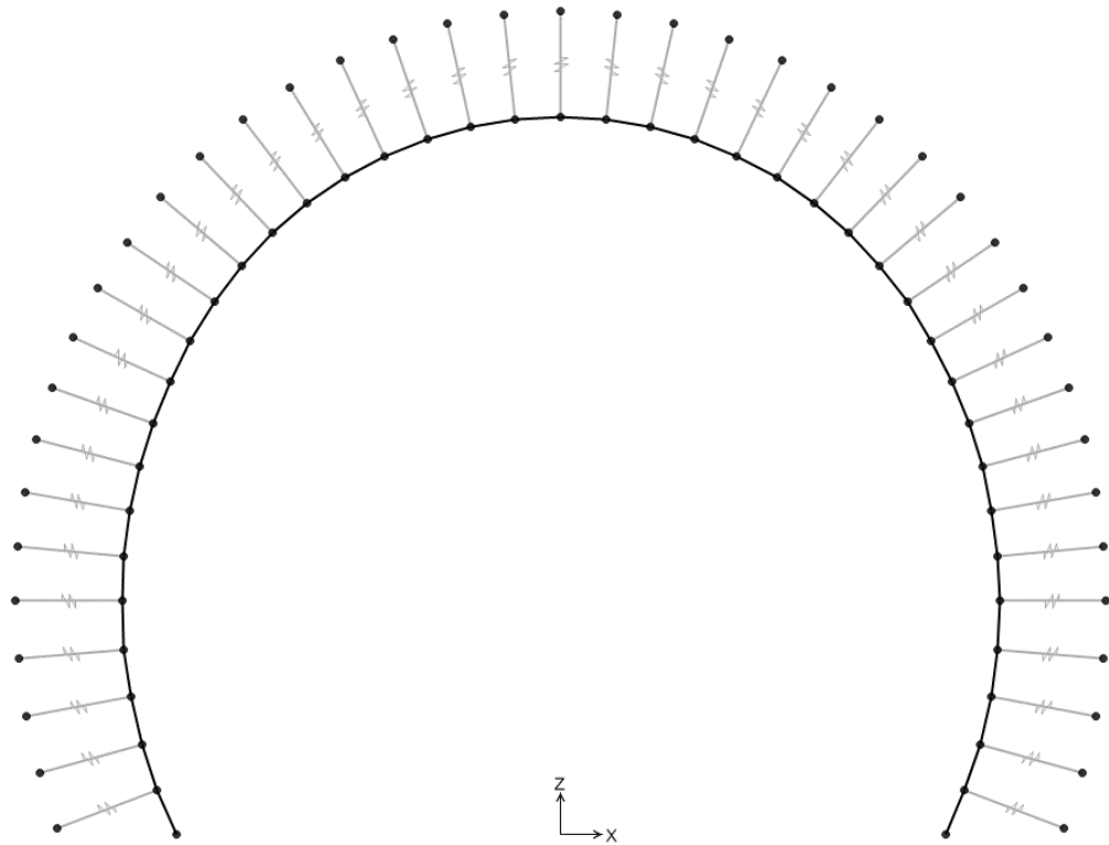
Abbildung 2: Geometrisches Modell des Ausbruchquerschnitts CL-E-T
