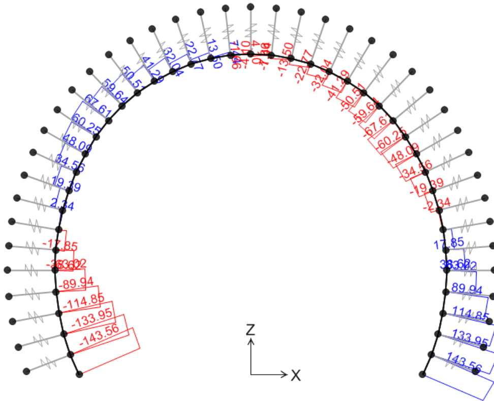
Abbildung 6: GZT06 - Schub
