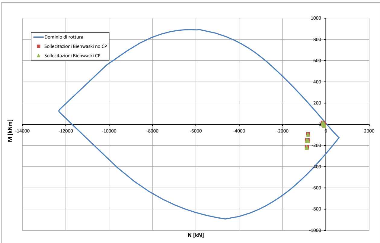
Abbildung 19: Überprüfung auf Beulspannung der Widerlager (außergewöhnliches GZT)
