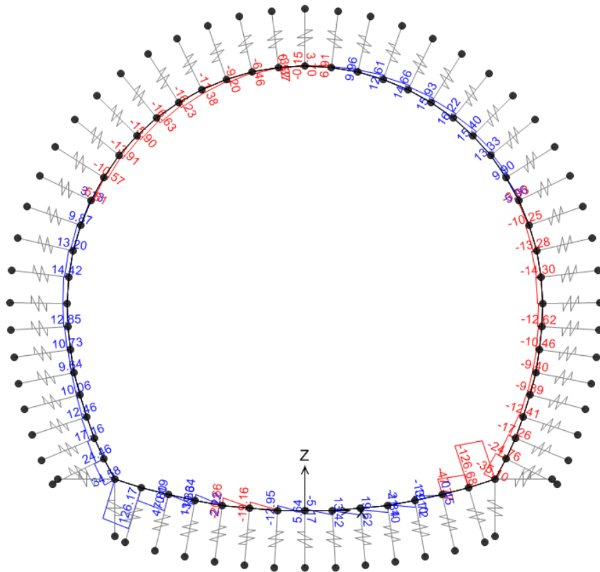
Abbildung 13: GZT04 - Schub nach Anwendung des Pöttler
