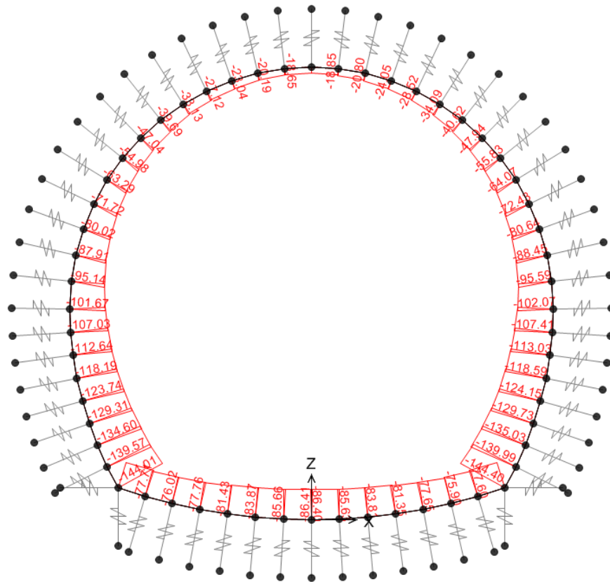
Illustrazione 9: SLU04 - Azione assiale
