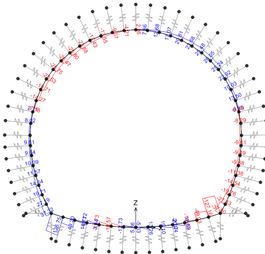
Illustrazione 10: SLU04 - Taglio
