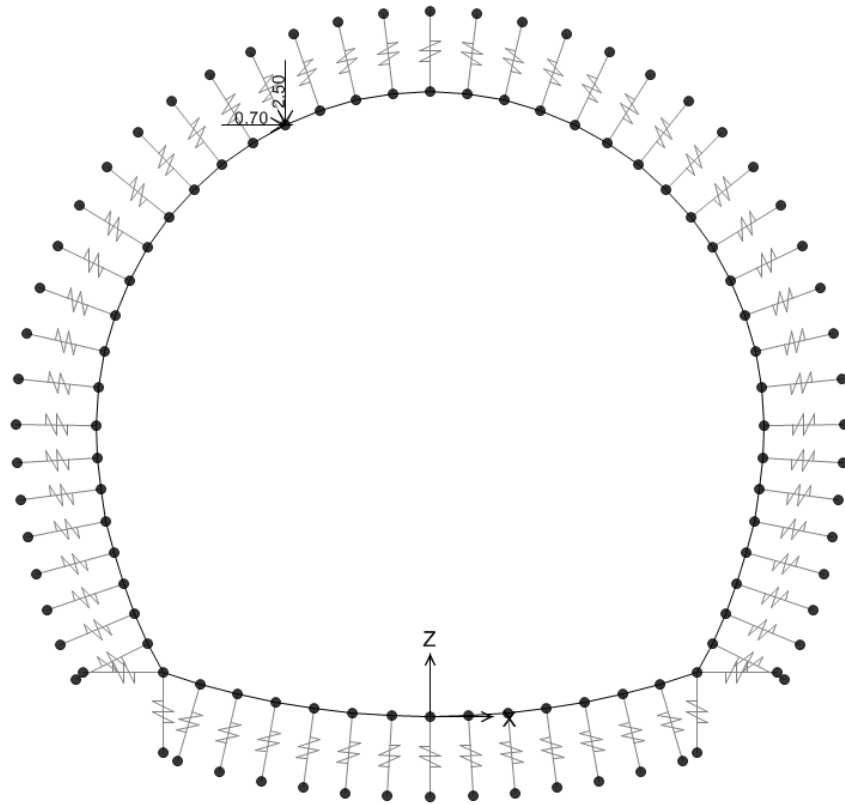
Illustrazione 3: Carico catenaria G2
