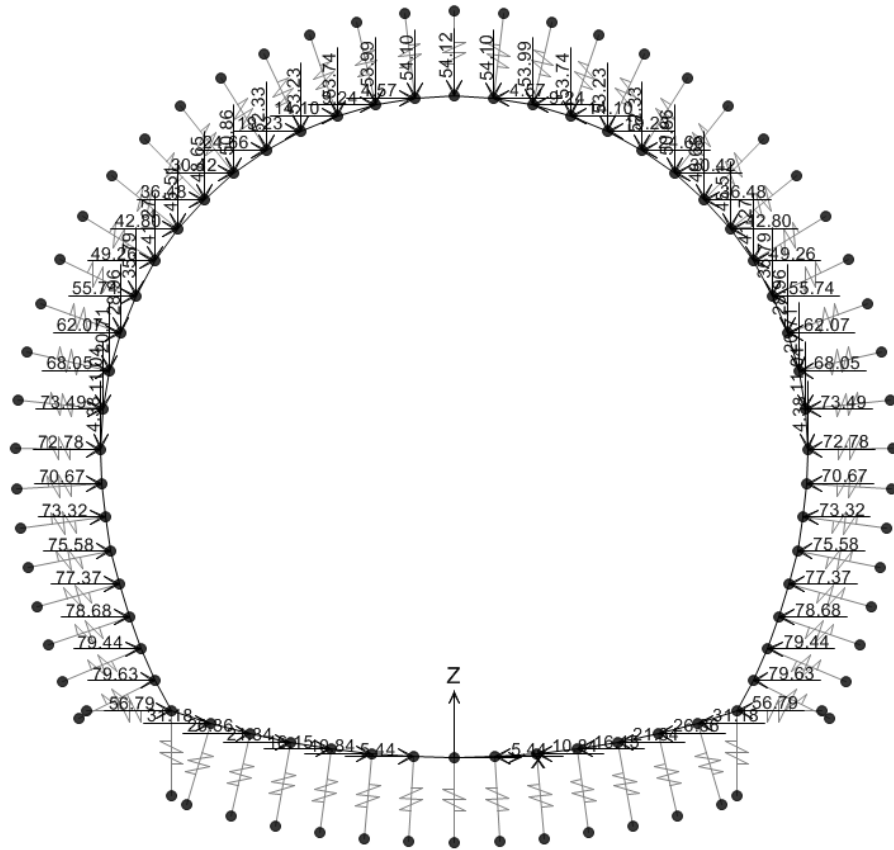
Illustrazione 5: Carico della roccia G5
