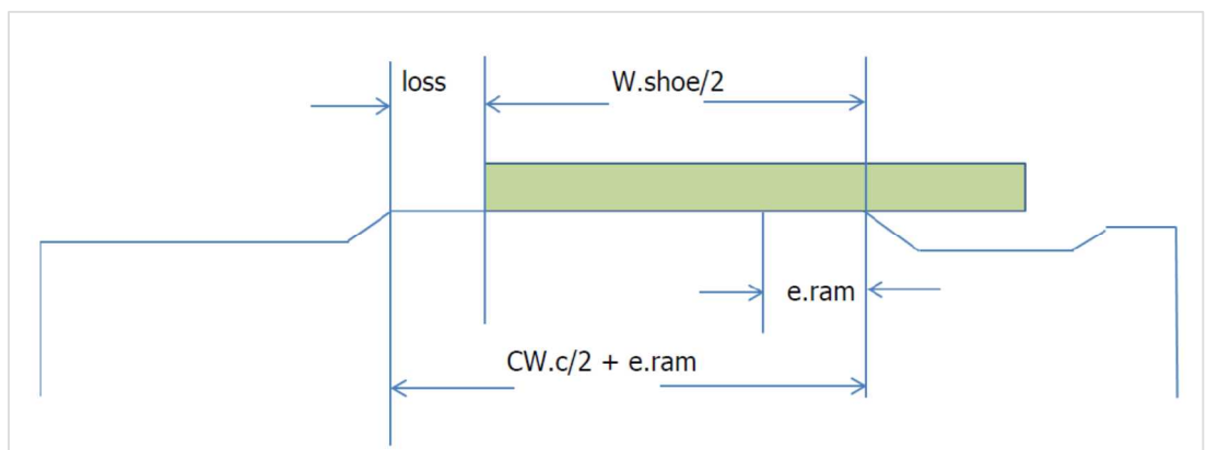
Abbildung 7: Einflussfläche der TBM-Schuhe
