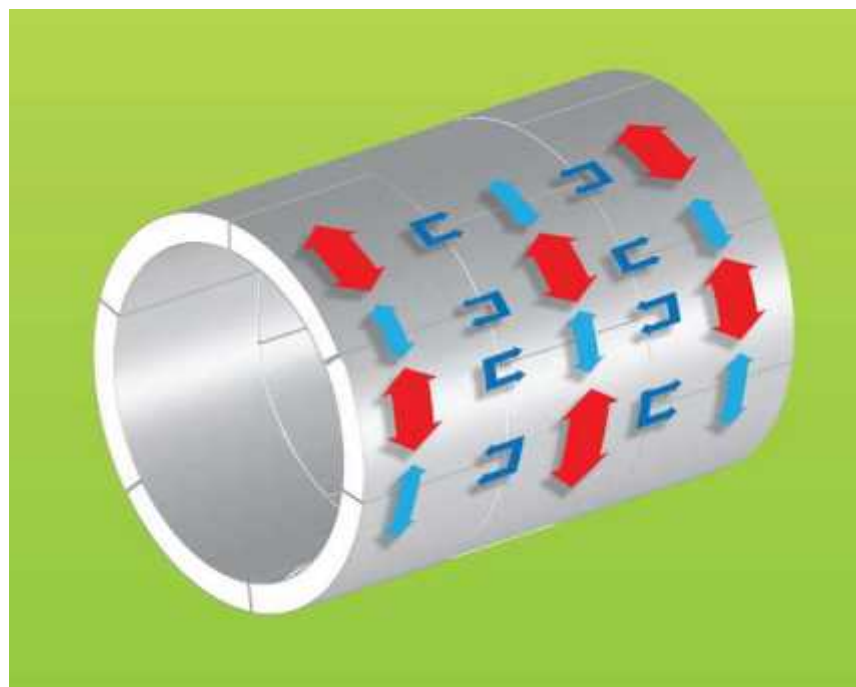
Abbildung 6: Spannungumlagerung aufgrund der Berücksichtigung einer durch Fugen verminderten Steifigkeit [11]
