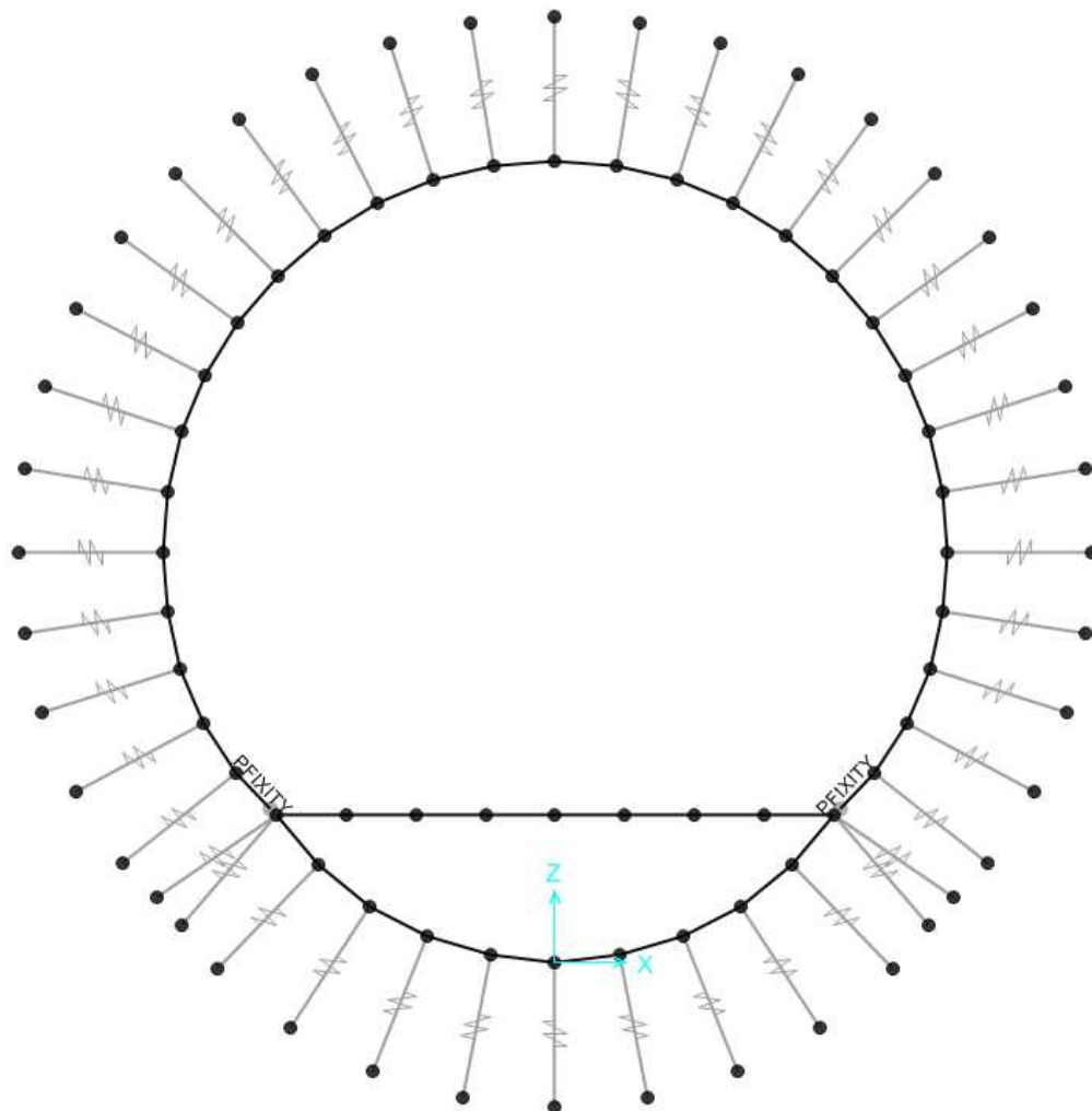
Abbildung 11: Geometrisches Modell der Regelquerschnitt C-MS
