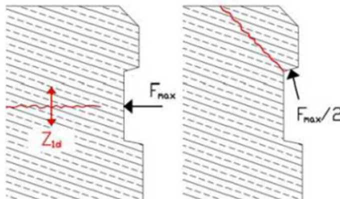
Abbildung 9: Nachweis des Spaltzugs Z_{id} und der Abplatzsicherheit unter der Rückstellkraft F_{max} des Dichtprofils
