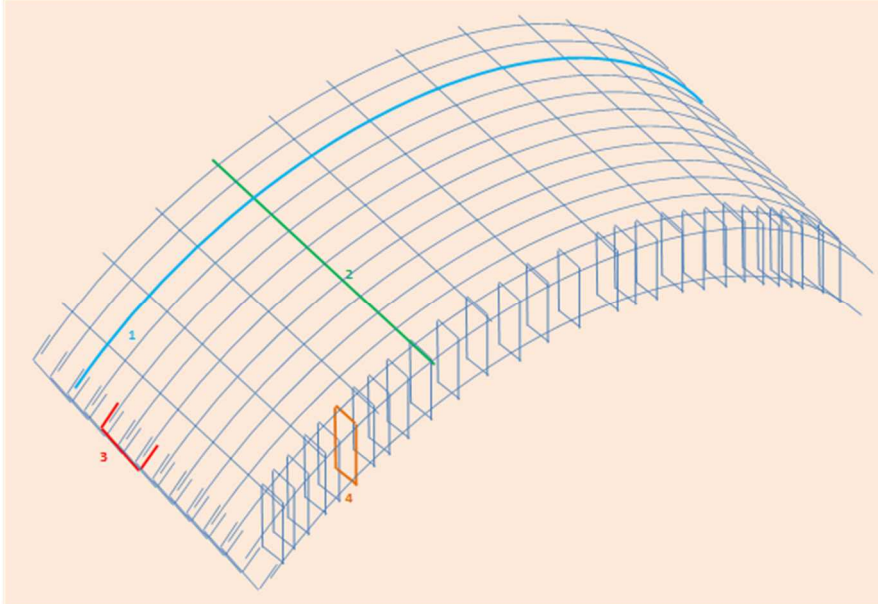
Abbildung 10: Schematische Darstellung für die Anordnung der Bewehrung in den Tübbing
