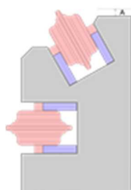
Abbildung 3: Verschiebungsmechanismus der Kronencutter
