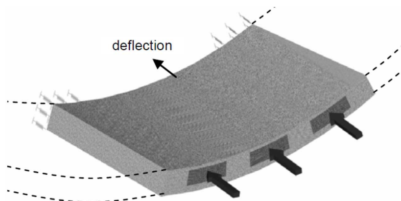
Figura 8: Mazze della TBM
