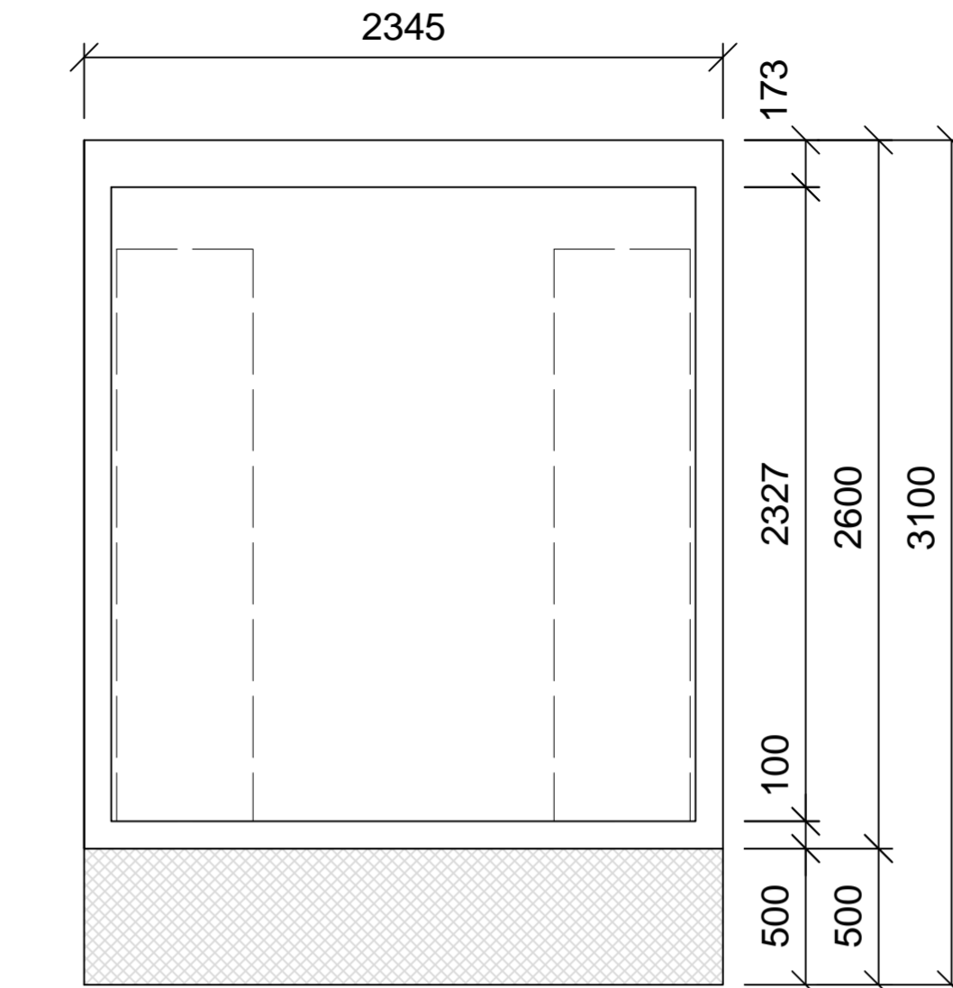
Ansicht 2 / Vista 2 1:25
