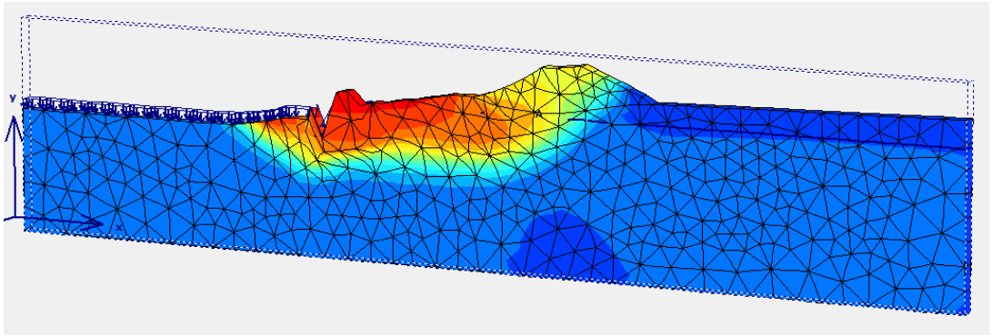
Eigengewicht + Erdbeben X-positiv (höchster Pegelstand) ohne Drainage Peso Proprio + Sisma X Positivo (livello Falda: Piena) – Condizione Non Drenata
