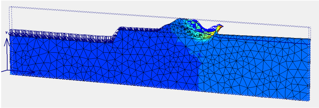
Eigengewicht + Erdbeben X-positiv (derzeitiger Pegelstand) mit Drainage Peso Proprio + Sisma X Positivo (livello Falda: Attuale) – Condizione Drenata
