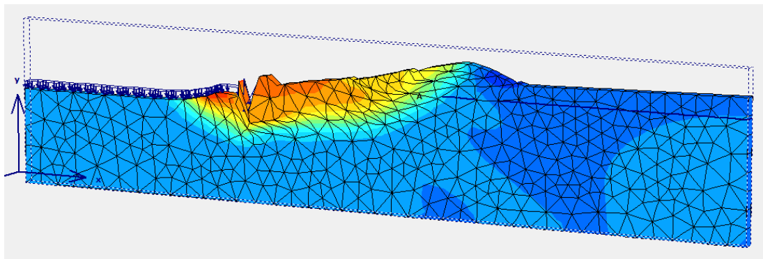
Eigengewicht + Erdbeben X-positiv (höchster Pegelstand) mit Drainage Peso Proprio + Sisma X Positivo (livello Falda: Piena) – Condizione Drenata
