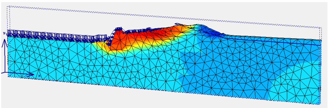
Eigengewicht + Erdbeben X-negativ (höchster Pegelstand) mit Drainage Peso Proprio + Sisma X Negativo (livello Falda: Piena) – Condizione Drenata
