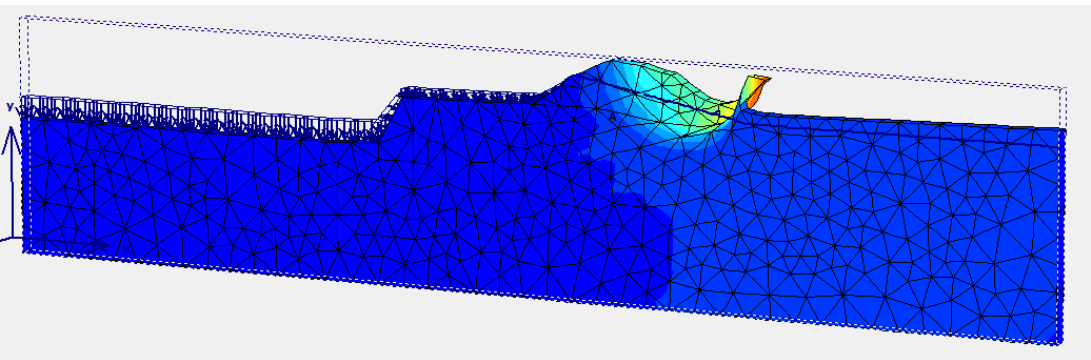
Eigengewicht + Erdbeben X-negativ (derzeitiger Pegelstand) mit Drainage Peso Proprio + Sisma X Negativo (livello Falda: Attuale) – Condizione Drenata
