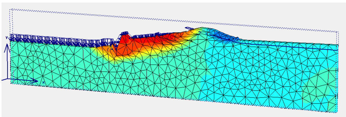
Eigengewicht + Erdbeben X-positiv (derzeitiger Pegelstand) ohne Drainage Peso Proprio + Sisma X Positivo (livello Falda: Attuale) – Condizione Non Drenata
