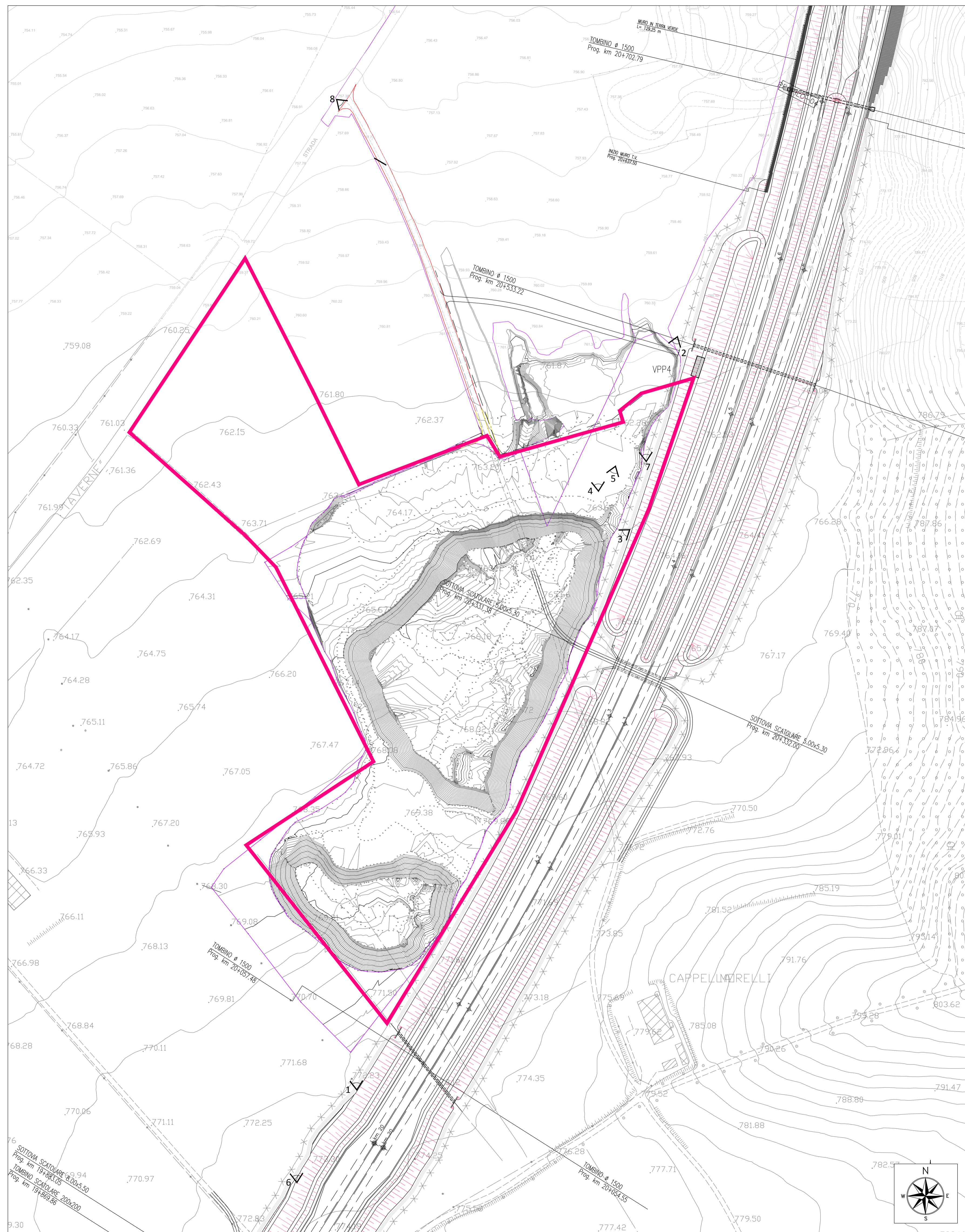
PLANIMETRIA DELLO STATO DI FATTO RILEVATO ALLA DATA DI APRILE 2014 - FUORI SCALA
