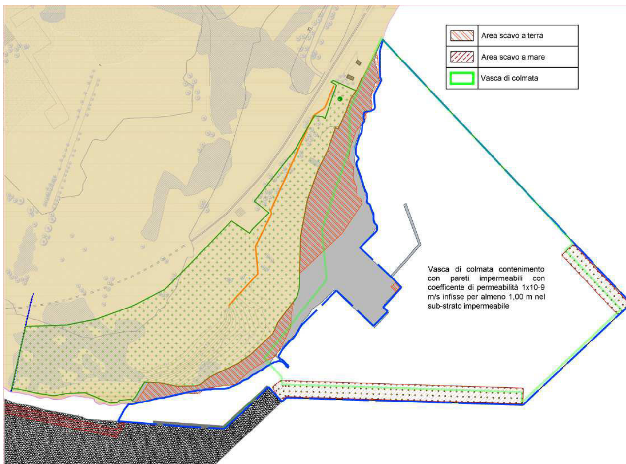
F5. Planimetria con indicazioni delle aree di scavo
