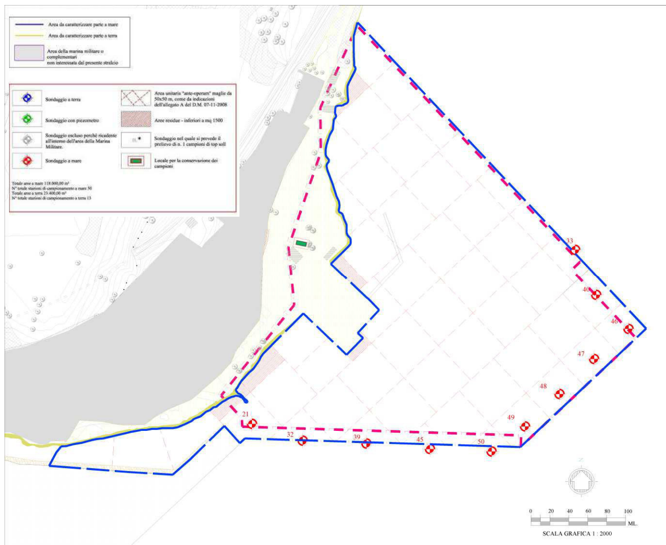
F4. Planimetria delle stazioni di campionamento a mare in corrispondenza delle banchine
