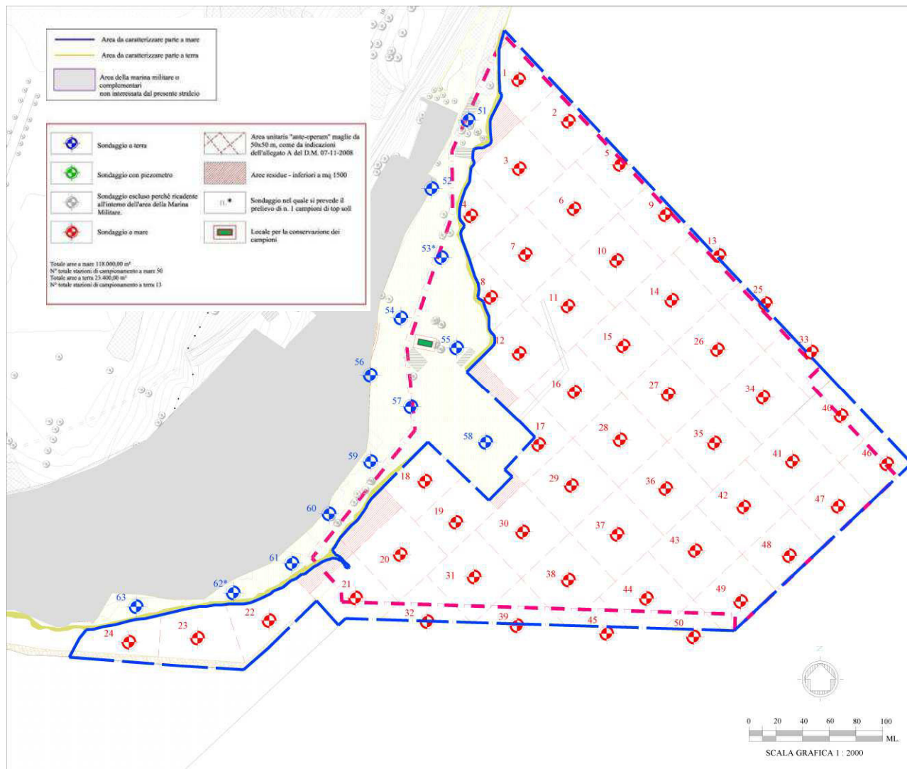
F2. Planimetria delle stazioni di campionamento
