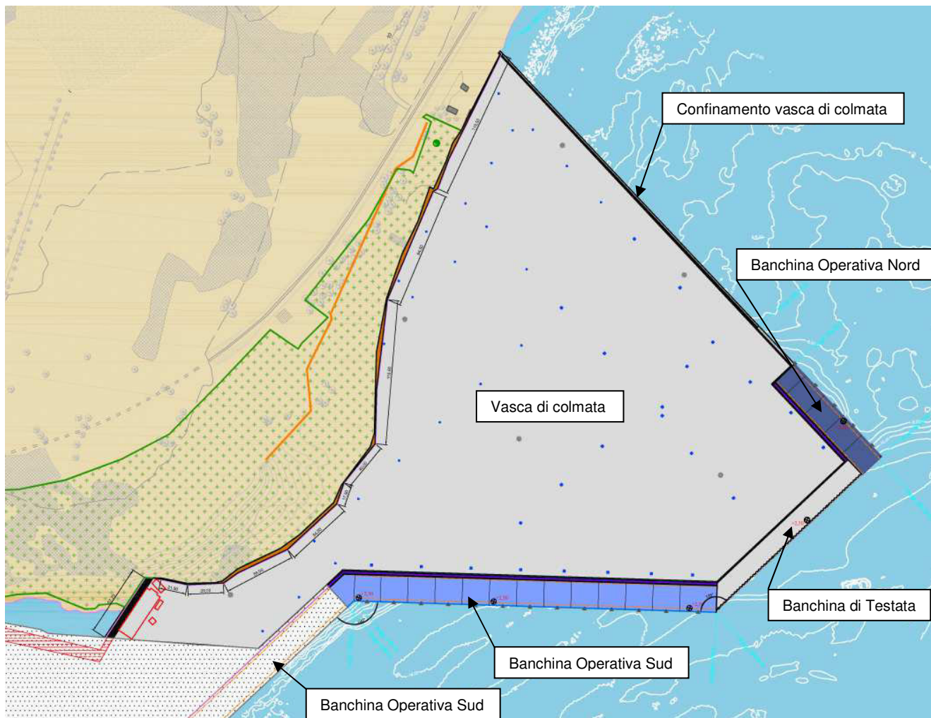
F1. Planimetria opere in progetto
