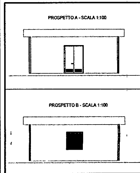
Stralci Elaborato n. A301-00-D-CV-AZ-GNVF-0X-001-A01 "Cabina TE PK 33+119.55 BD (33+112.00 BP) Copertura scala di accesso alla cabina TE"
