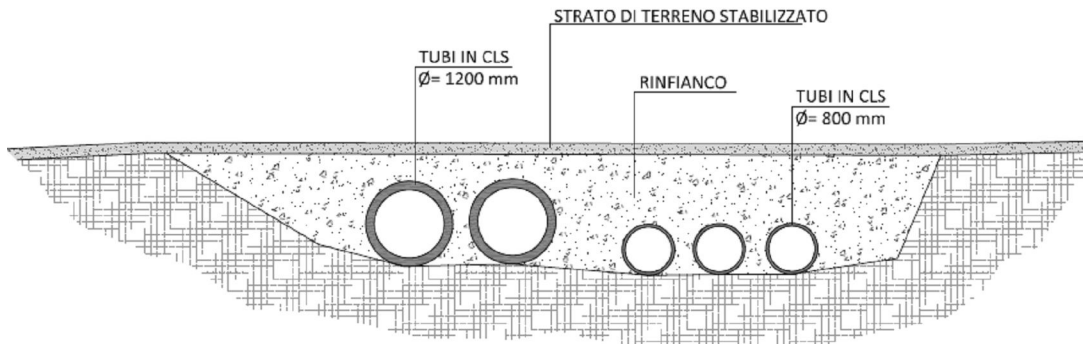
Sezione trasversale del guado esistente
