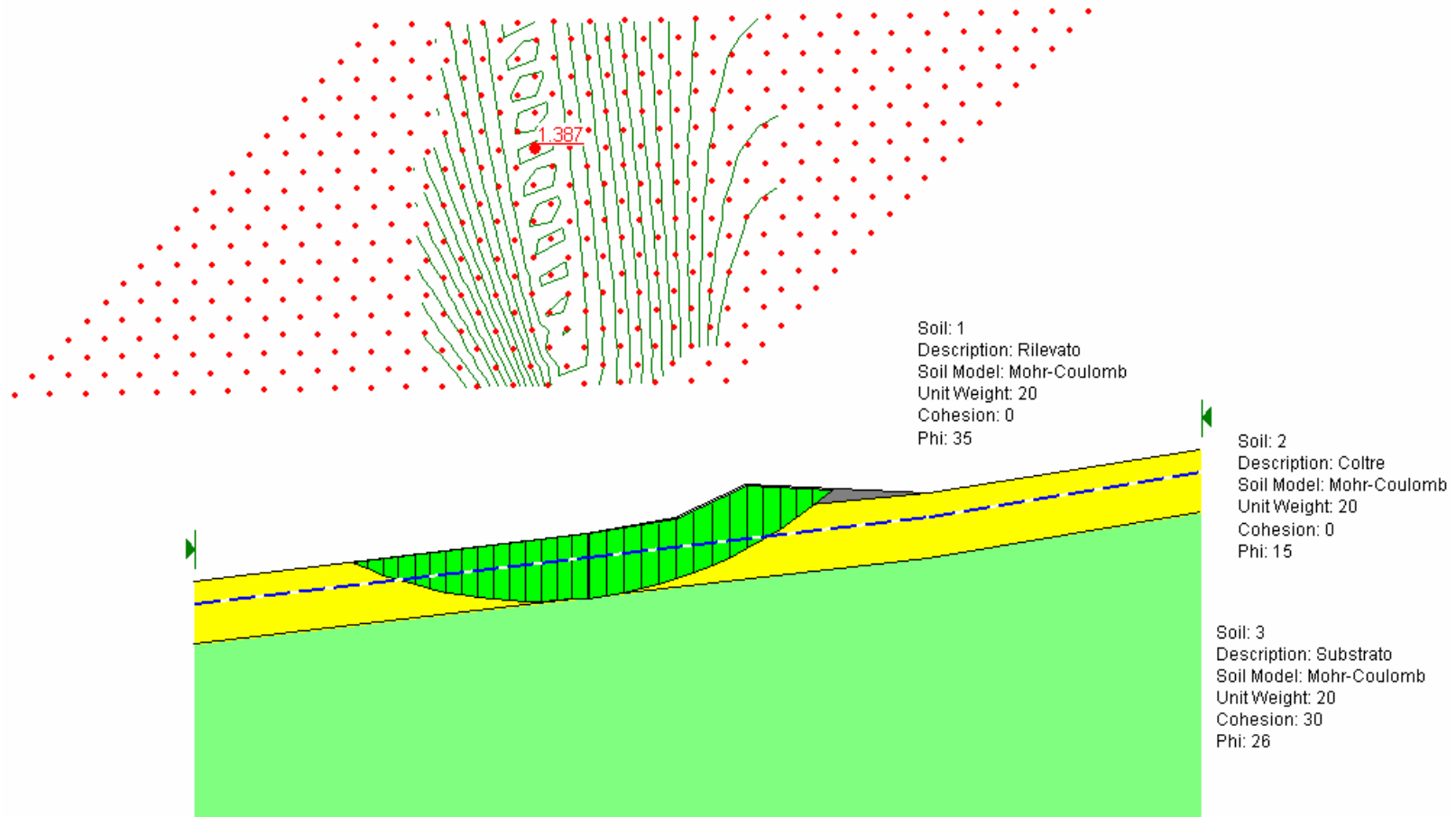
Figura 6.2- Analisi limite nelle condizioni iniziali per la definizione della superficie di rottura critica
