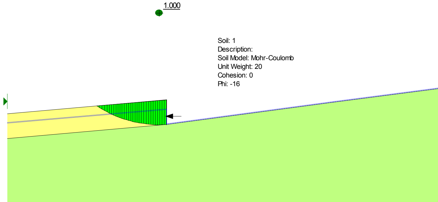
Figura 6.4- Analisi limite per la valutazione dell'azione che instabilizza il cuneo di valle con FS = 1.0 nelle condizioni iniziali
