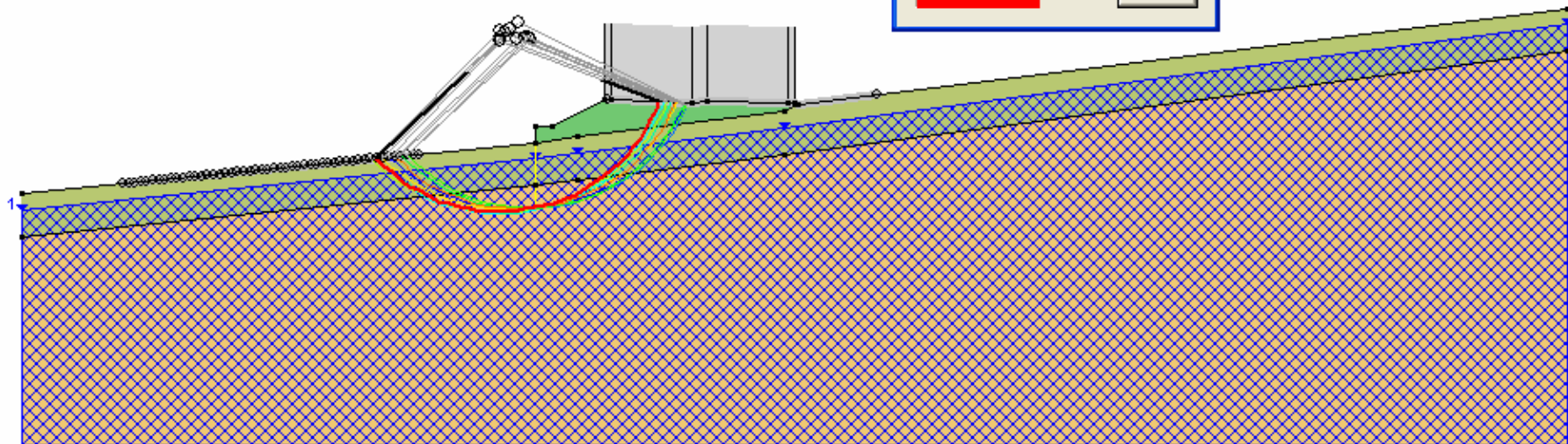
Figura 7.1- Analisi di stabilità globale nel caso statico ed individuazione della superficie di scorrimento avente F_s minimo
